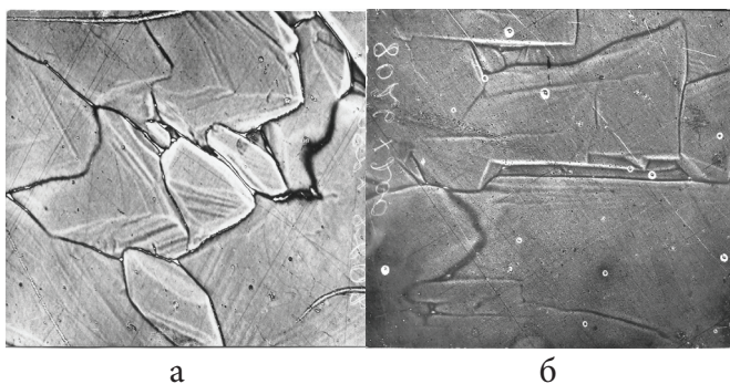
Рис. 5. Пластино-блочная структура и двойники при \delta \rightarrow \gamma превращении: а, б – сплав с С = 0,1 %, Si = 2,0 %; а, б – \times 200 , в поляризованном свете, травлено ниталем
