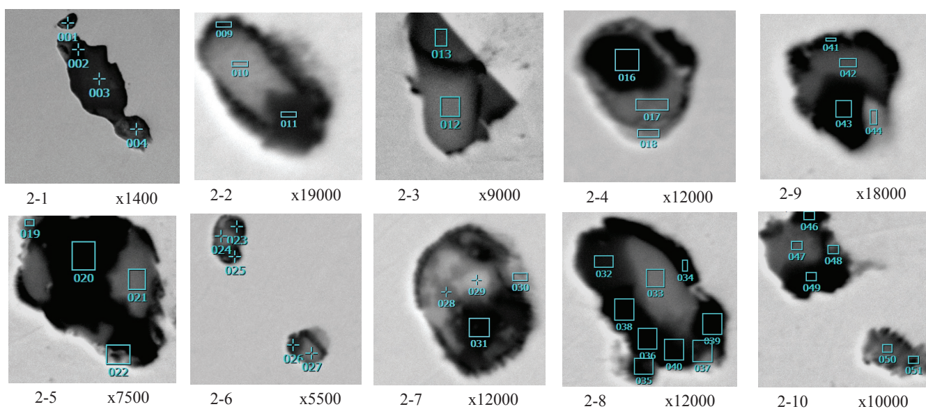
Рис. 4. Электронно-оптические изображения микроструктуры гетерофазных неметаллических включений в образца № 2, полученные в отраженных вторичных электронах; хим.составы неметаллических включений 2-1,.....2-10 приведены в табл. 11
