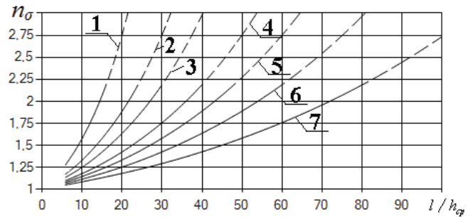
Рис. 3. Зависимости n_\sigma = \varphi(l/h_{cp}) при холодной прокатке тонких и особо тонких полос: 1 – f = 0,15 ; 2 – то же 0,10 ; 3 – то же 0,08 ; 4 – то же 0,06 ; 5 – то же 0,05 ; 6 – то же 0,04 ; 7 – то же 0,03 Погрешность расчета n_\sigma по уравнению (7) составляет не более \pm 1,5 - 2,0 \% и только при малых коэффициентах трения ( f \leq 0,035 - 0,04 ) и больших значениях фактора формы очага деформации ( l/h_{cp} > 60 - 85 ) достигает 5,0 \% . Уравнение (7) справедливо при f = 0,03 - 0,15 и l_c/h_{cp} = 4 - 85 .
