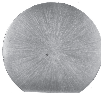
Рис. 2. Макроструктура бочки прокатного валка из чугуна с шаровидной формой графита Ø 450 мм (в осевой зоне виден след горячего спая термопары) [7]
