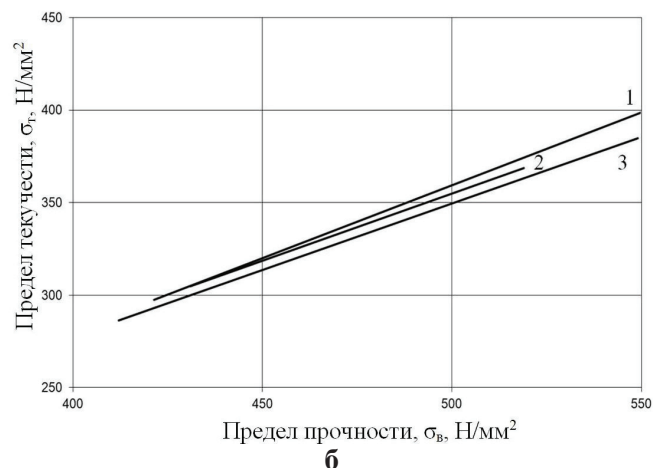
Рис. 6. Положение предела текучести в зависимости от предела прочности для горячекатаных (а) и холоднодеформированных (б) труб, изготовленных из трубной заготовки ОАО «ЧМК» (1), ОАО «ЗМЗ» (2), ОАО «ВТЗ» (3)
