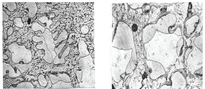
Рис. 3. Начало образования перитектического аустенита (зерна \gamma при фазовом контакте \delta/\delta/\gamma ): а, б – сплав с C = 0,5 %, Si = 8,0 %; а – \times 800 , б- \times 1500 , травление пикратом натрия
