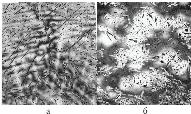
Рис. 4. Частичное превращение \delta \rightarrow \gamma при закалке от 1300 °С: а – сплав с С = 0,17 %, Si = 2,5 %, Mn = 0,5 %; б – сплав с С = 0,04 %, Si = 2,0 %, Mn = 0,8 %; а – охлаждение 100 °С/мин; б – 10 °С/мин; а – \times 50 ; б – \times 300 ; травление пикратом натрия
