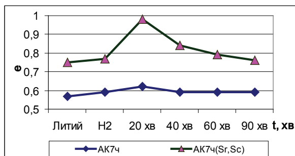
Рис. 3. Залежності технологічної деформівності сплавів АК7ч та АК7ч (Sr, Sc) від часу водневого оброблення розплаву
