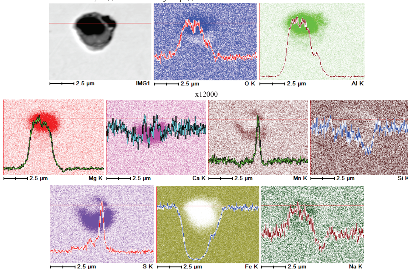
Рис. 6. Колесная сталь, обр. 2. Результаты PCMA неметаллического включения в режиме линейного сканирования
