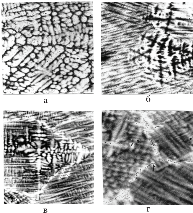
Рис. 2. Первичная рекристаллизация и границы зерен в дендритной структуре стали с \delta -стабилизаторами: а, б – сплав с содержанием C = 0,1 %; Al = 2 %; Si = 0,08 %, Mn = 0,45 %; в, г – сплав с содержанием C = 0,05 %, Si = 2,26 %; а – \times 200 ; б, в, г – \times 100 ; травление пикратом натрия
