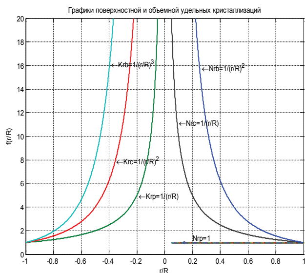
Рис. 4. Влияние положения фронта затвердевания по глубине отливок различной конфигурации на изменение количества центров кристаллизации на единицу поверхности ( Nr ) и объема ( Kr ) затвердевающего сплава: R – радиус (половина толщины) отливок; r – не затвердевшая часть металла; r/R = 0 – осевая зона отливок; r/R = 1 , r/R = -1 – наружная поверхность отливок; индексы для конфигурации отливок: p – плоская полубесконечная пластина; c – цилиндр полубесконечный; b – шар; N_r = 1 , K_r = 1 на поверхности отливок
