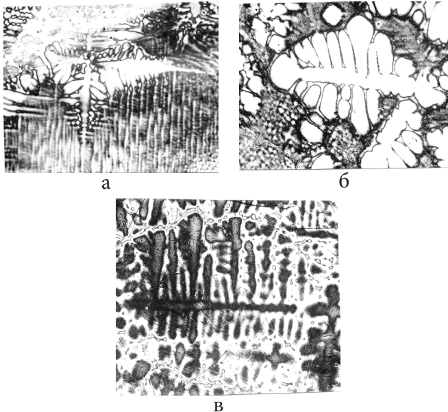
Рис. 1. Структура дендритов при кристаллизации низкоуглеродистых сталей: а – дендриты и упорядоченная остаточная жидкость в сплаве с C = 0,05 %, Si = 0,25 %; б – автономные дендриты в жидкости в сплаве с C = 0,03 %, Si = 0,50 %; в – окончание затвердевания сплава с C = 0,05 %, Si = 0,20 %; а, в – \times 100 ; б – \times 200 ; травление пикратом натрия
