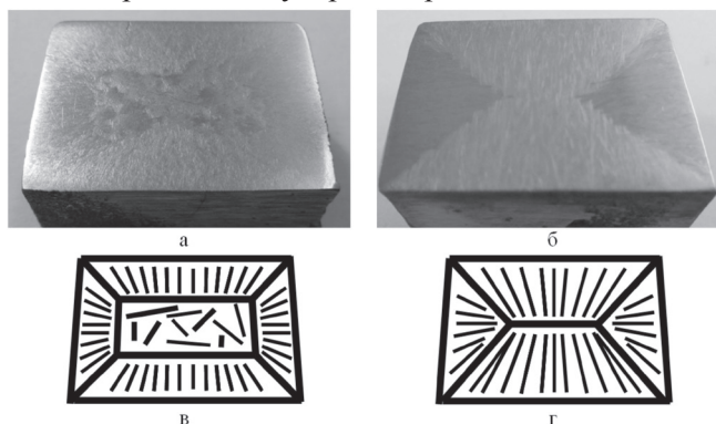
Рис. 1. Макроструктура (а, б) и схема кристаллизации (в, г) хромомарганцевого чугуна 280Х20Г4Л не модифицированного (а, в) и модифицированного присадками титана и РЗМ (б, г)
