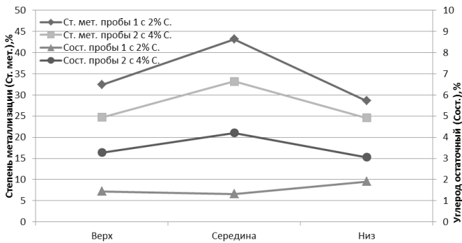
Рис. 3. Влияние содержания топлива в слое на степень металлизации и содержание остаточного углерода в спеке
