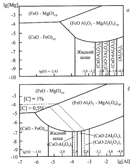
Рис. 7. ПРМК системы Fe-C-O-Al-Ca-Mg при 5ppm (а) и 50 ppm (б) Ca; 1550 °С, P = 101 кПа [3]
