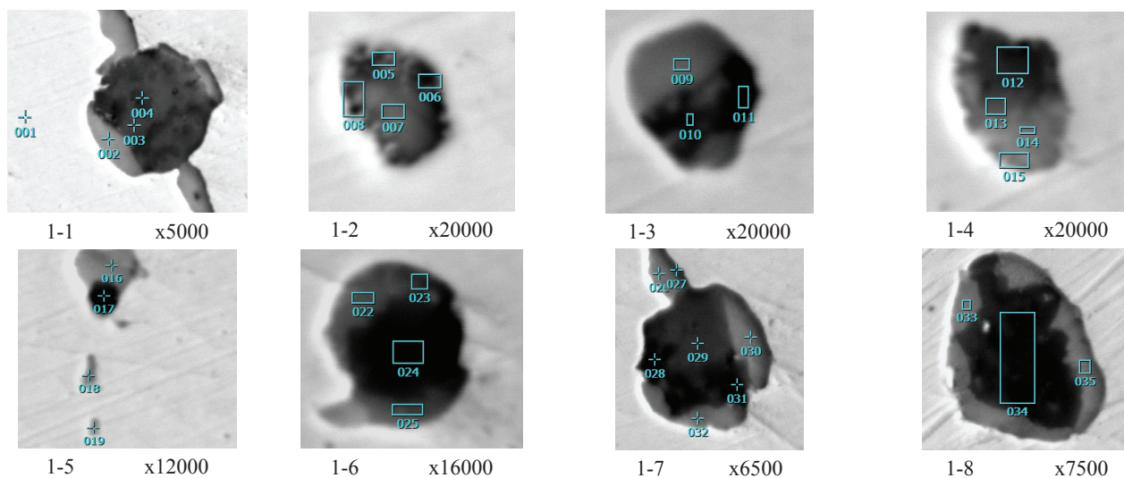
Рис. 3. Электронно-оптические микроструктуры гетерофазных неметаллических включений в образце № 1, полученные в отраженных вторичных электронах; хим.составы неметаллических включений 1-1,..1-8 приведены в табл. 10
