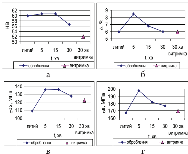
Рис. 1. Вплив гідроциркуляційного оброблення на показники механічних властивостей сплаву АК7ч, що містить 0,1 % Sr, 0,5 % Sc: а – твердість сплаву; б – відносне подовження; в – межа плинності; г – межа міцності
