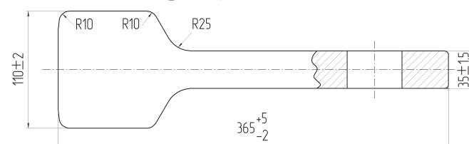
Рис. 1. Готовый фасонный профиль Методика исследований
