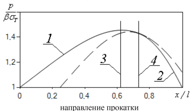
Рис. 1. К определению положения нейтрального сечения при холодной прокатке: 1, 2 – кривые, описываемые, соответственно, уравнениями (5) и (6) (пунктиром показана действительная часть кривых 1, 2); 3 – положение максимума эпюры нормальных контактных напряжений; 4 – положение нейтрального сечения
