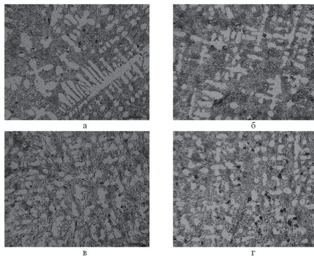
Рис. 2. Микроструктура хромомарганцевого чугуна 280Х20Г4Л в зависимости от присадки титана и РЗМ (х 100), %: а – 0,0 РЗМ, 0,0 Тi; б – 0,1 РЗМ, 0,2 Тi; в – 0,2 РЗМ, 0,15 Тi; г – 0,5 РЗМ, 0,15 Тi
