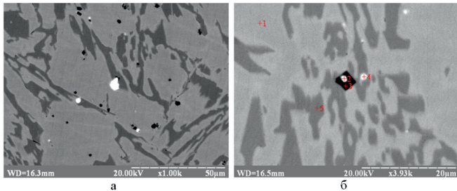
Рис. 3. Микроструктура хромомарганцевого чугуна 280Х20Г4Л, содержащего присадки титана и РЗМ ×1000 (а) и ×4000 (б)
