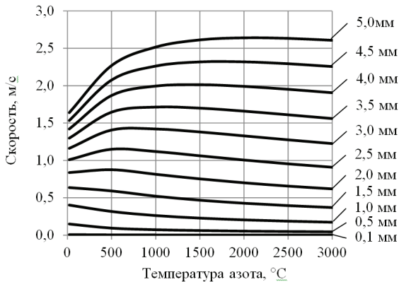
Рис. 1. Зависимость первой критической скорости псевдоожога от температуры азота (частицы графита 0,1-5,0 мм)
