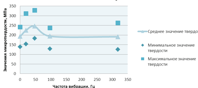
Рис. 5. Зависимость микротвердости Al в эвтектическом сплаве Al-Si от частоты вибрации в кристаллизаторе
