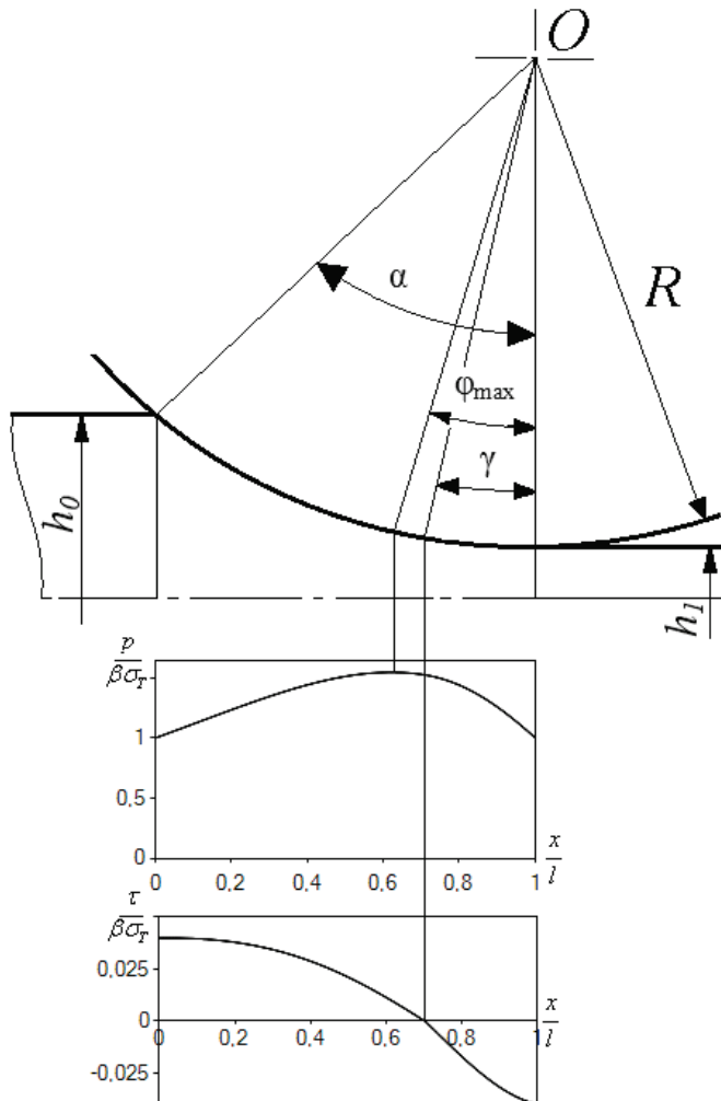
Рис. 2. Эпюры нормальных контактных напряжений и напряжений трения при холодной прокатке ( R = 300 мм; R/h_0 = 1000 ; f = 0,04 ; \varepsilon = 0,35 )
