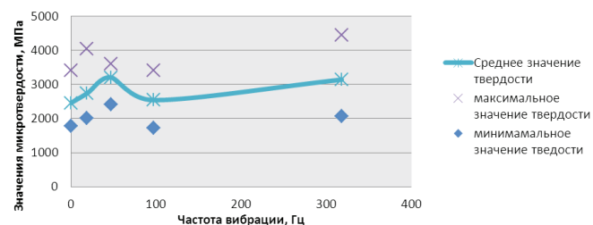
Рис. 6. Зависимость микротвердости Si в эвтектическом сплаве Al-Si от частоты вибрации в кристаллизаторе
