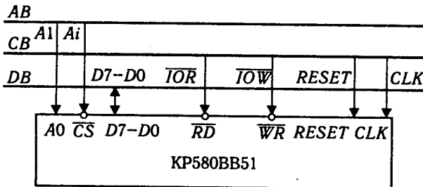
Рис. 5.52. З'єднання УСАПП із шинами МП
