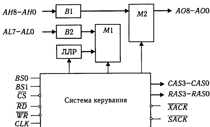
Рис. 4.7. Структурна схема контролера динамічної пам'яті і8207
