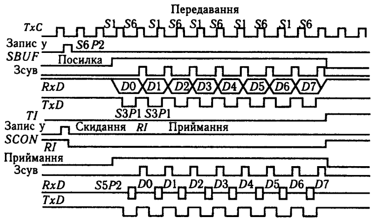
Рис. 6.12. Послідовний порт в режимі 0: а – функціональна схема; б – діаграми
