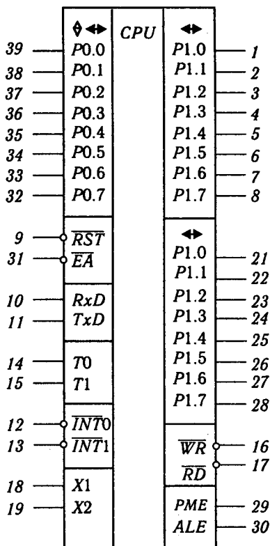
KP1816BE51 (20=GND, 40=+5V)
