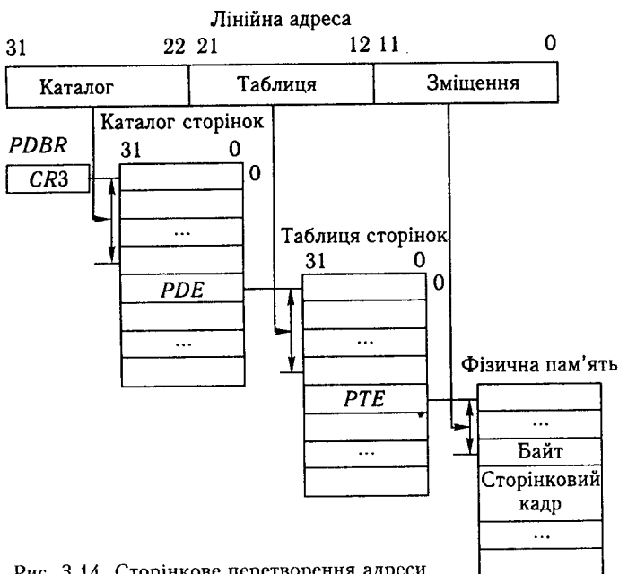
Рис. 3.14. Сторінкове перетворення адреси
