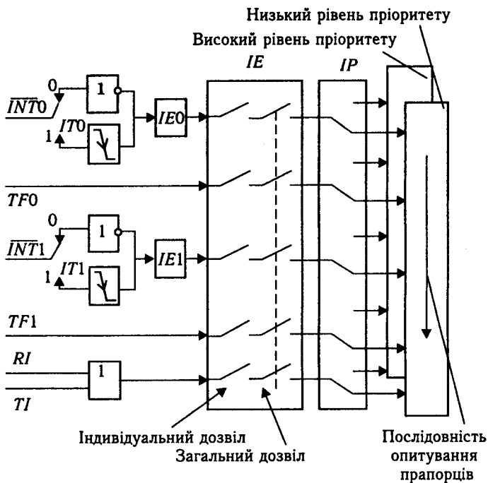
Рис. 6.19. Функціональна схема системи переривань
