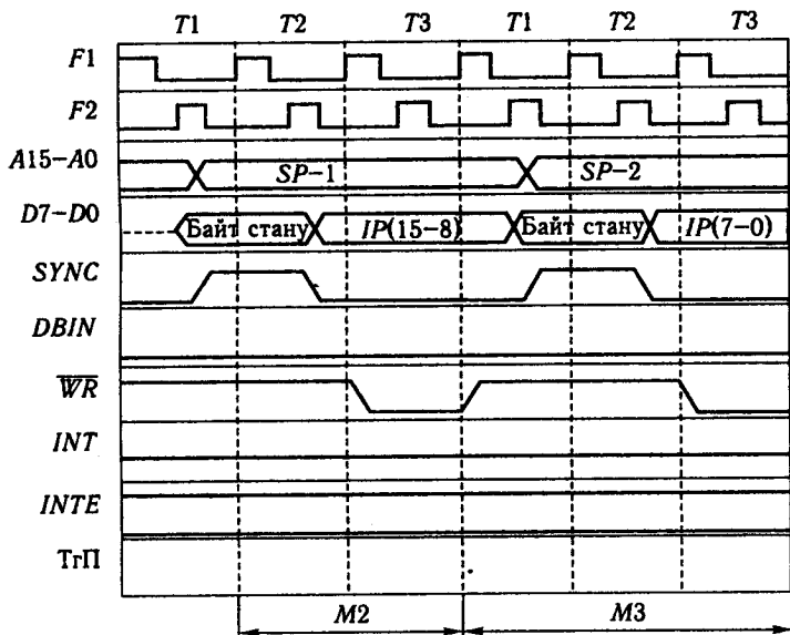
Рис. 2.7. Часові діаграми циклу ПЕРЕРИВАННЯ:
