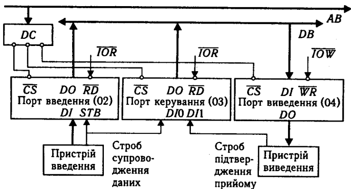
Рис. 5.3. Схема введення-виведення даних за стробом готовності
