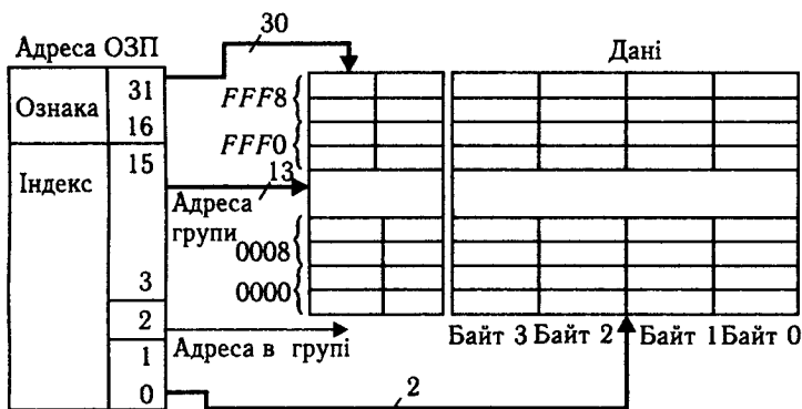
Рис. 4.12. Структурна схема двовходової множинної асоціативної кеш-пам'яті
