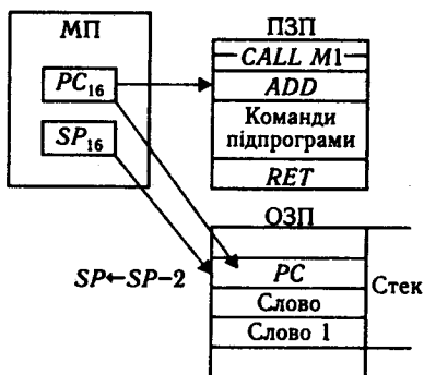
Рис. 4.17. Робота стеку під час виклику підпрограми
