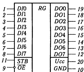
Рис. 2.28. Графічне позначення буферного регістра i8282
