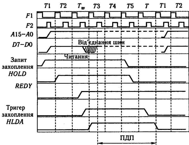
Рис. 2.8. Цикл ЧИТАННЯ ПАМ'ЯТІ в режимі ПДП
