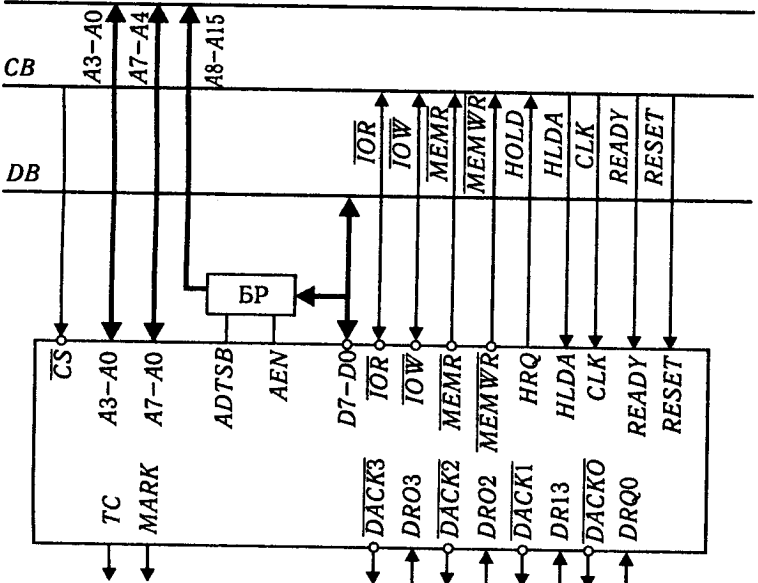
Рис. 5.46. Схема з'єднання КПДП із системою шиною з використанням буферного регістра
