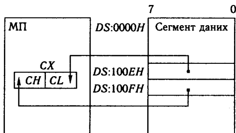
Рис. 2.20. Виконання команди MOV [100EH], CX
