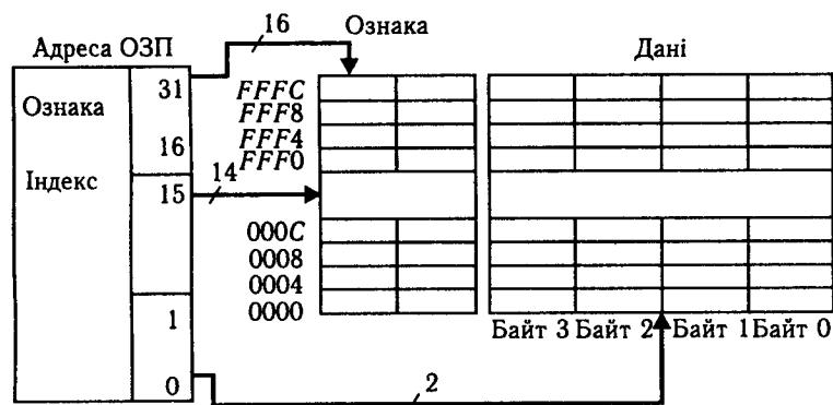
Рис. 4.10. Структурна схема кеш-пам'яті з прямим відображенням
