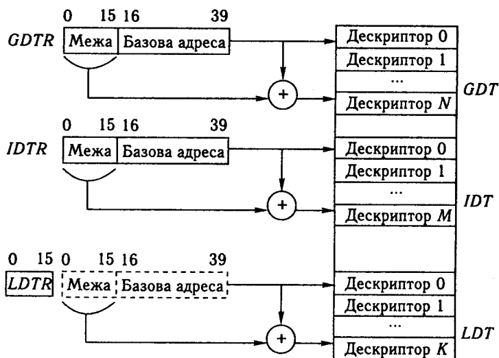
Рис. 3.5. Розміщення дескрипторних таблиць у пам'яті
