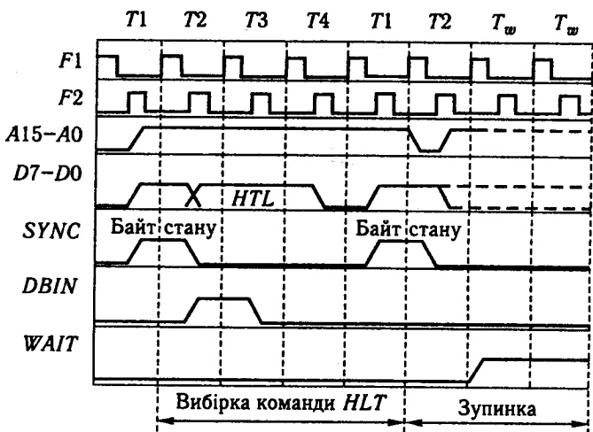
Рис. 2.9. Цикл ЗУПИНКА
