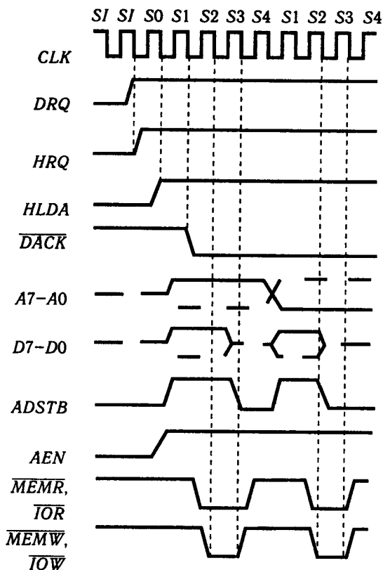
Рис. 5.50. Часові діаграми основних сигналів
