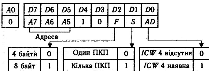
Рис. 5.58. Формат керуючого слова ініціалізації ICW1
