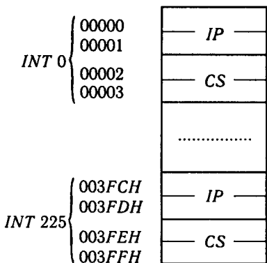
Рис. 2.18. Карта векторів переривань
