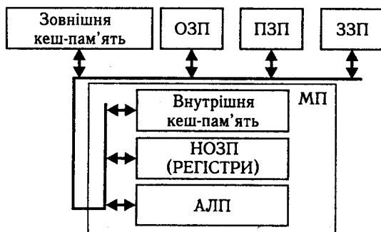
Рис. 4.1. Типи пам'яті в МПС
