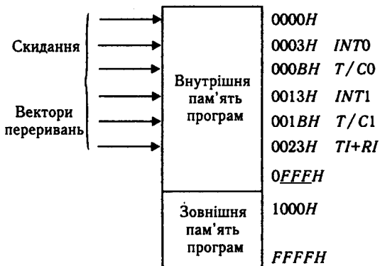
Рис. 6.3. Розподіл адресного простору РПП
