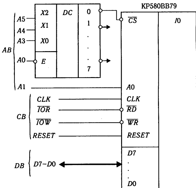
Рис. 5.19. З'єднання ВІС KP580BB79 із системною шиною МПС
