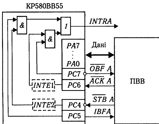
Рис. 5.16. Схема під'єднання ПВВ до ВІС КР580ВВ55 у режимі 2
