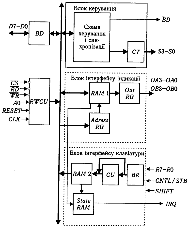
Рис. 5.18. Структурна схема програмованого інтерфейсу клавіатури індикації
