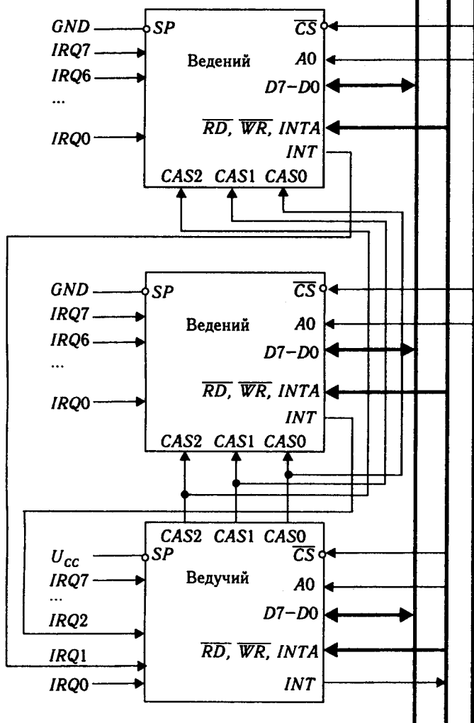
Рис. 5.57. Каскадне з'єднання ПМКП
