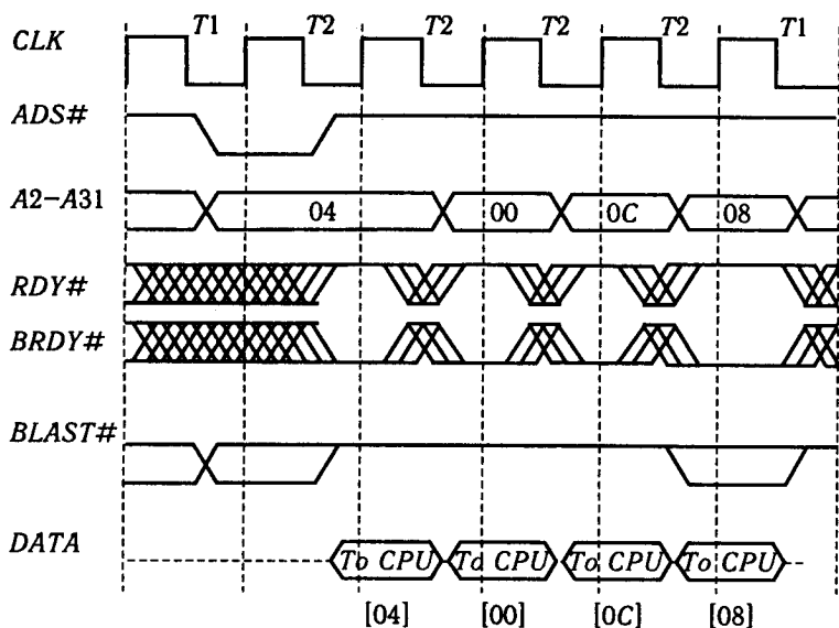
Рис. 3.15. Діаграма пересилання вмісту чотирьох 32-розрядних комірок пам'яті
