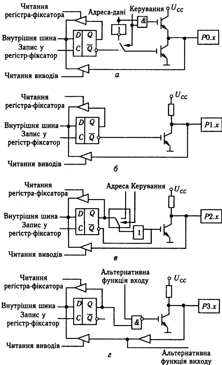
Рис. 6.11. Принципові схеми ліній портів: a – P0; б – P1; в – P2; г – P3
