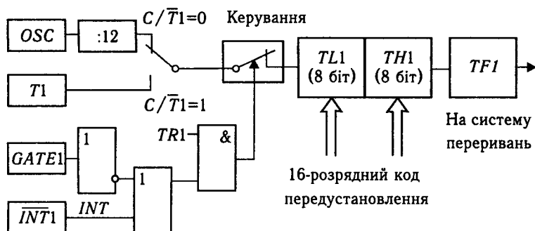
Рис. 6.16. Функціональна схема T/C1 у режимі 1
