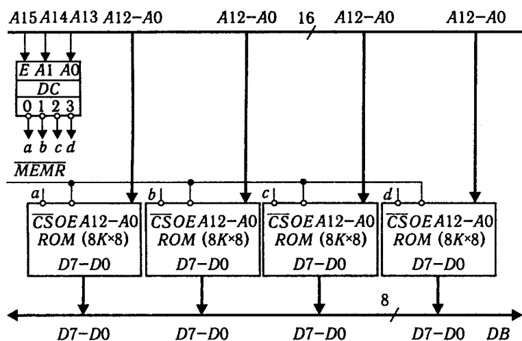
Рис. 4.3. Модуль ПЗП ємністю 32 Кбайт \times 8
