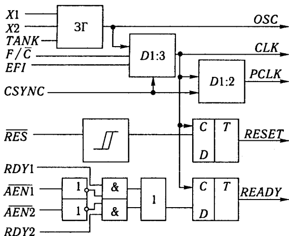
Рис. 2.25. Структурна схема ВІС генератора i8284
