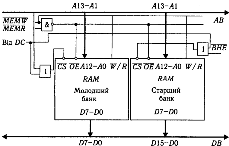
Рис. 4.6. Модуль ОЗП у 16-розрядних МПС
