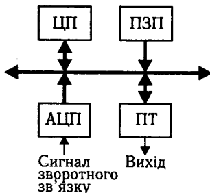
Рис. 5.64. Структурна схема МПС керування
