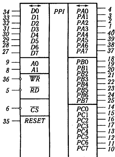
Рис. 5.8. Графічне позначення VIC KP580BB5
