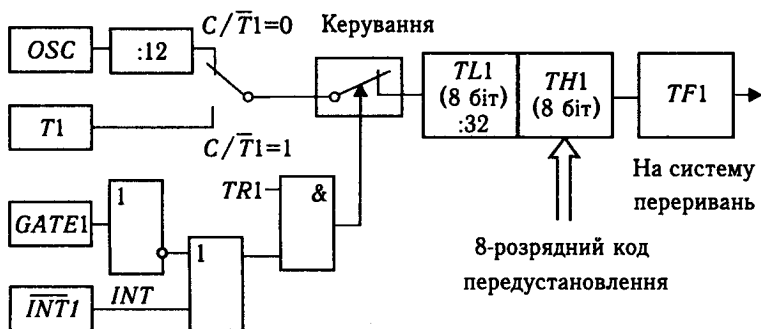
Рис. 6.15. Функціональна схема T/C1 у режимі 0
