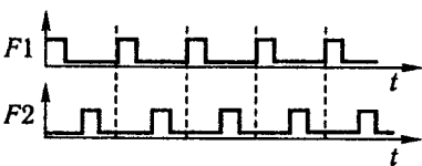
Рис. 2.2. Часові діаграми імпульсів синхронізації F1 і F2
