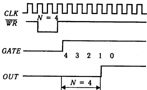
Рис. 5.40. Режим программованої затримки
