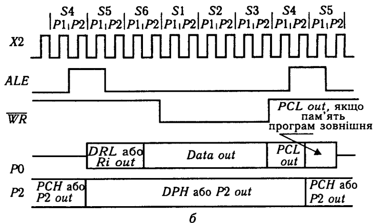
Рис. 6.25. Часові діаграми циклів: а — читання зовнішньої пам'яті даних; б — запису у зовнішню пам'ять даних
