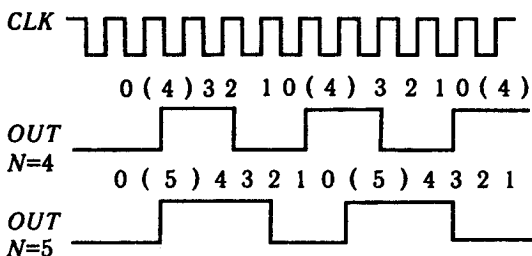
Рис. 5.43. Режим генератора прямокутних імпульсів
