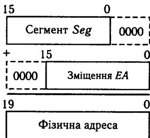
Рис. 2.14. Формування фізичної адреси
