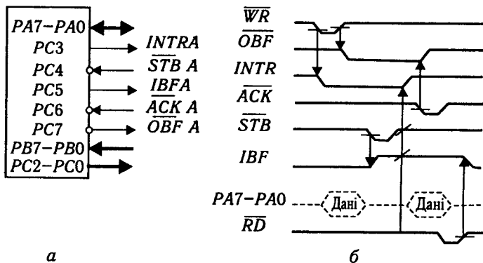
Рис. 5.17. Робота BIC у режимі 2:
