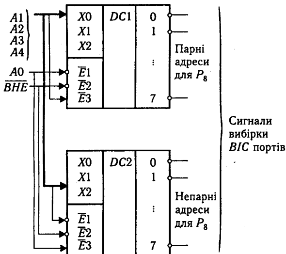
Рис. 5.2. Функціональна схема дешифратора портів
