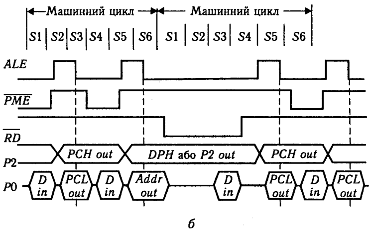
Рис. 6.23. Часові діаграми машинних циклів читання зовнішньої пам'яті програм:
