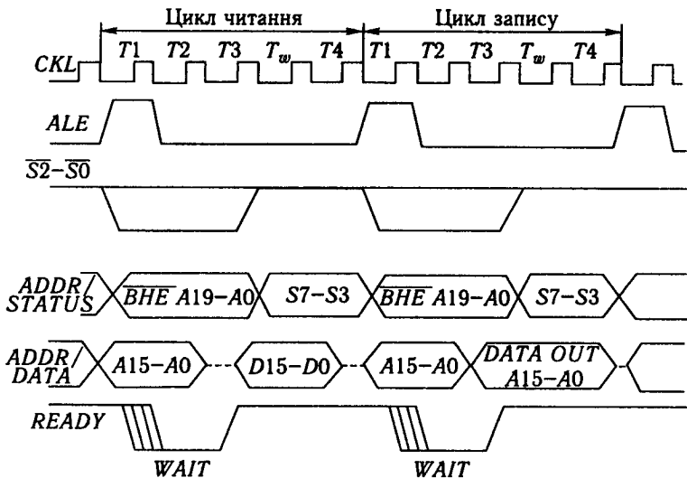
Рис. 2.17. Цикли ЧИТАННЯ і ЗАПИСУ МП і8086 у мінімальному режимі
