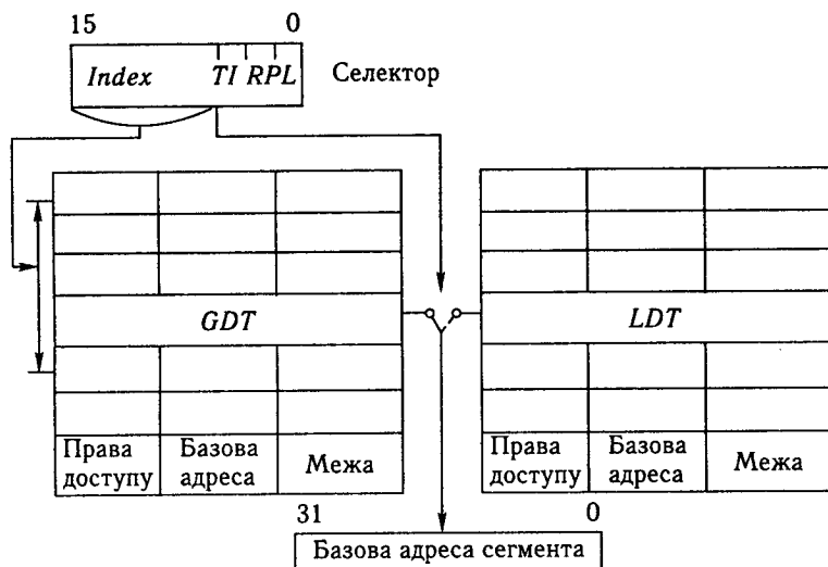
Рис. 3.11. Формування базової адреси сегмента
