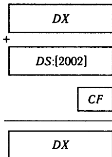
Рис. 2.23. Виконання команди ADC DX,[2002H]
