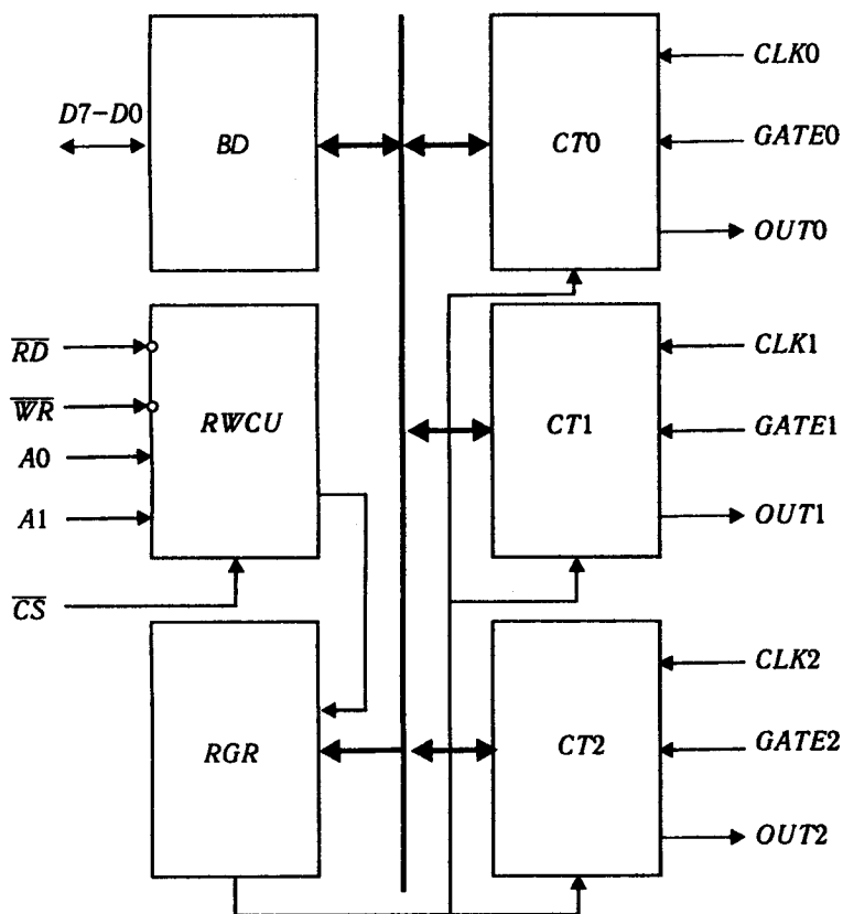
Рис. 5.34. Структурна схема ВІС таймера КР580ВИ54:
