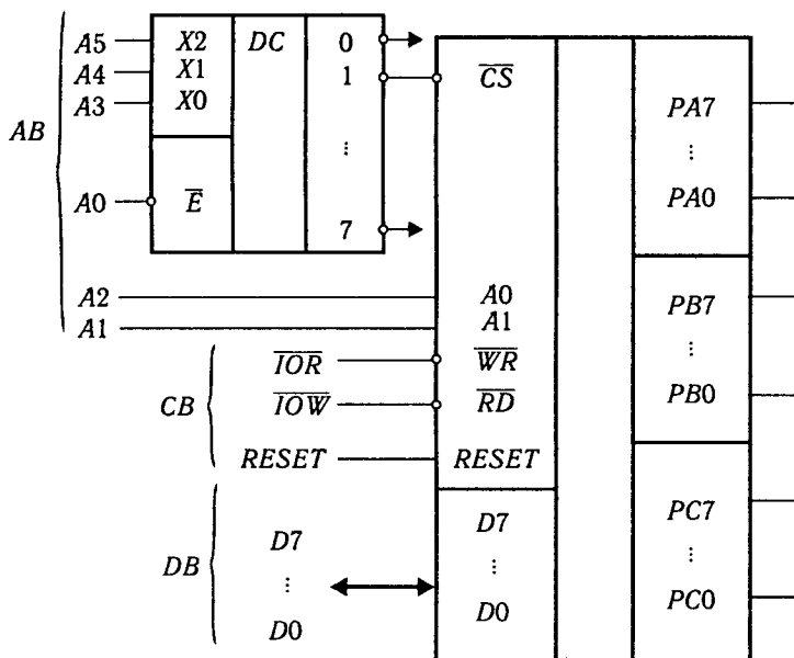
Рис. 5.9. Функціональна схема з'єднання ВІС КР580ВВ55 із системною шиною
