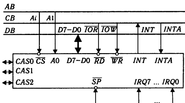
Рис. 5.56. З'єднання BIC KP580BH59 зі стандартною системою шин
