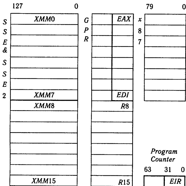
Рис. 3.18. Архітектура x86-64
