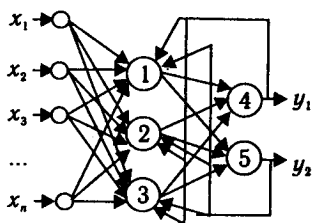
Рис. 9.5. Циклічна нейронна мережа
