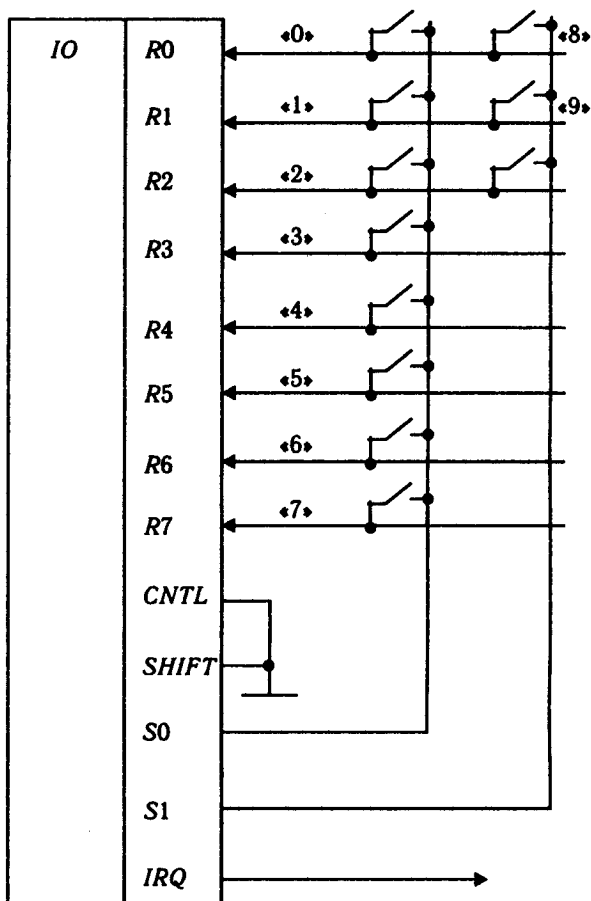
Рис. 5.33. Функціональна схема з'єднання BIC з клавіатурою
