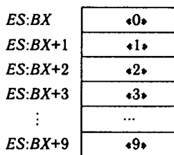
Рис. 2.21. Розміщення семисегментних кодів у пам'яті
