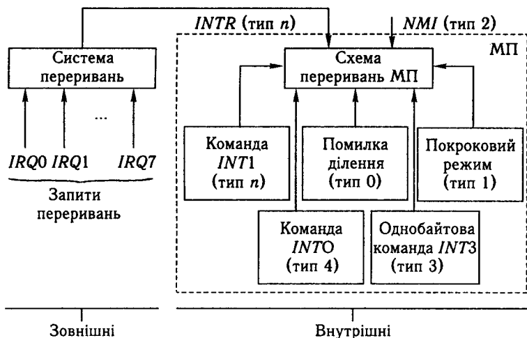
Рис. 2.19. Типи переривань
