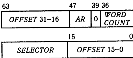
Рис. 3.13. Формат вентилів
