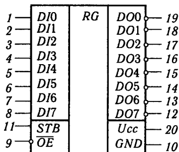
Рис. 2.29. Графічне позначення буферного регістра i8283
