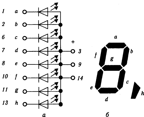
Рис. 5.28. Семисегментний індикатор АЛС321Б: а – принципова схема; б – розміщення світлодіодів
