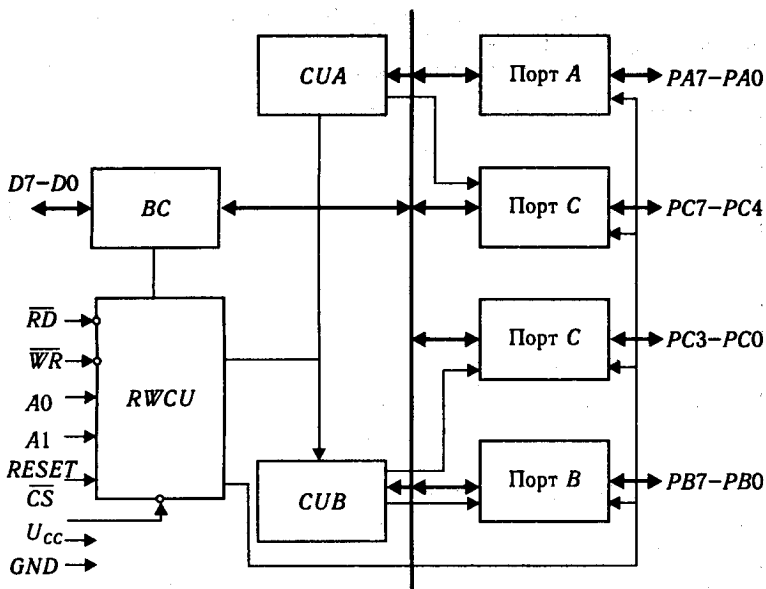
Рис. 5.7. Структурна схема VIC KP580BB5
