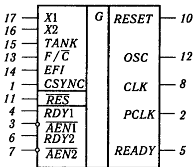
Рис. 2.26. Графічне позначення ВІС генератора i8284
