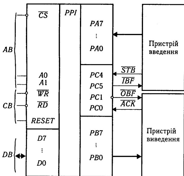
Рис. 5.13. Схема з'єднання пристрою введення з портом А, пристрою виведення – з портом В у режимі 1
