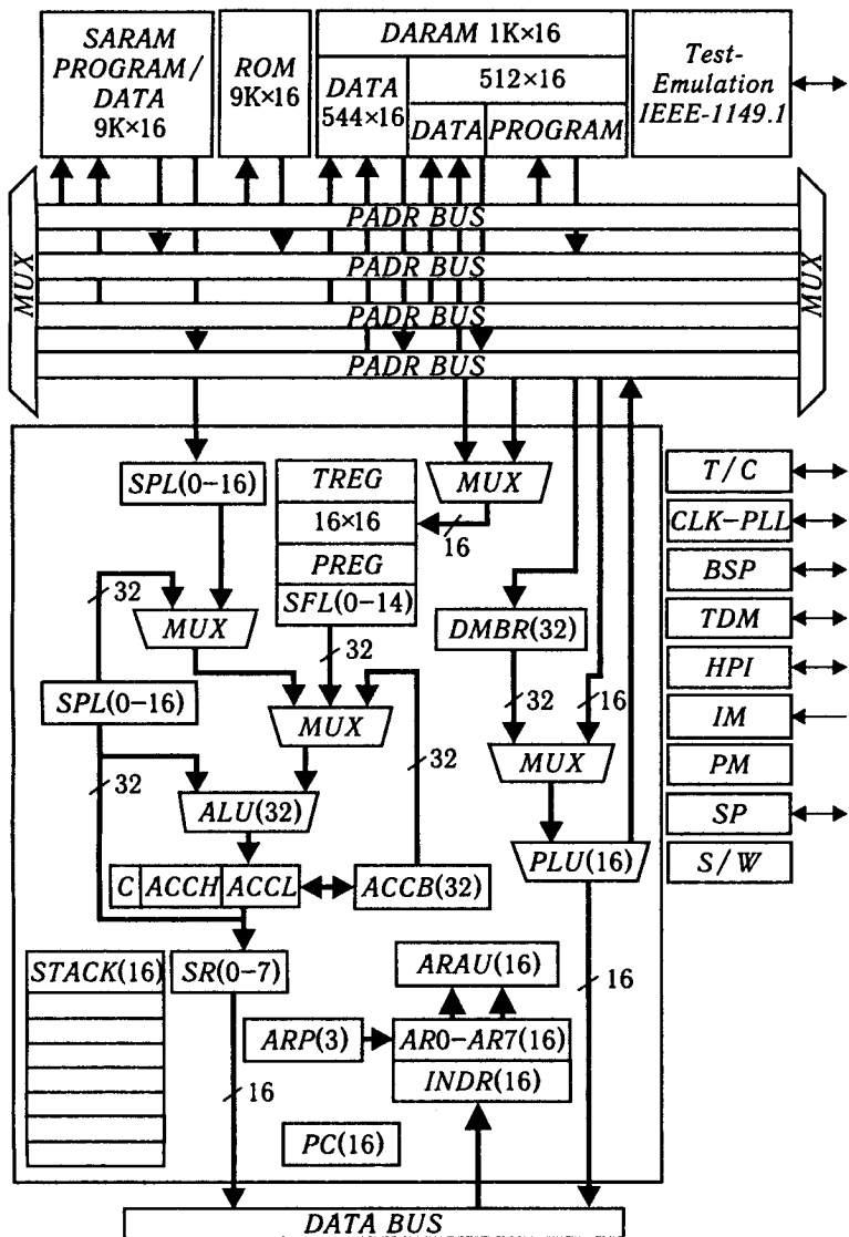
Рис. 8.1. Архітектура цифрового сигнального процесора TMS320XC5x
