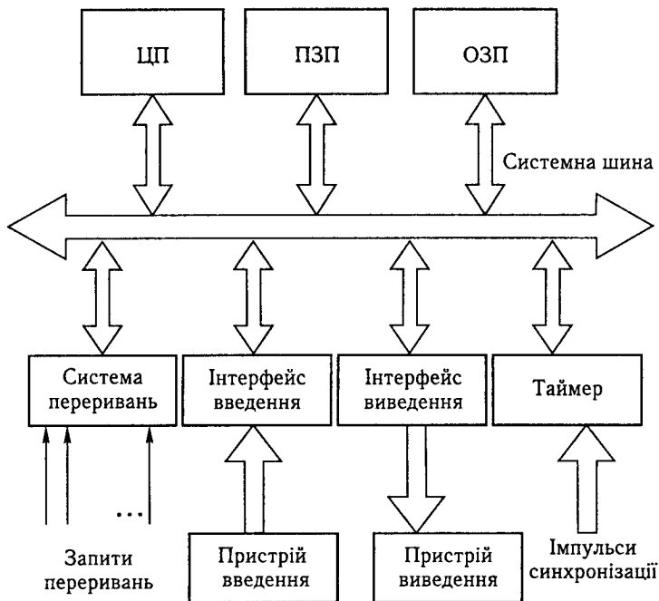
Рис. 1.4. Узагальнена структурна схема мікропроцесорної системи керування
