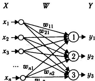
Рис. 9.3. Одношаровий персептрон
