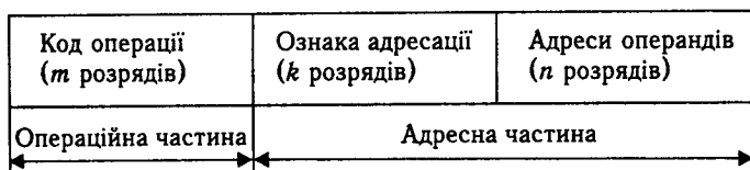
Рис. 1.8. Формат команди
