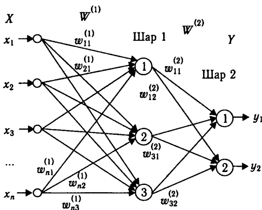
Рис. 9.4. Двошаровий персептрон
