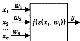
Рис. 9.2. Модель нейрона
