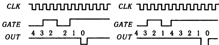
Рис. 5.44. Діаграми роботи таймера:
