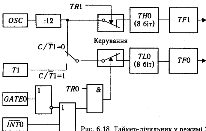
Рис. 6.18. Таймер-лічильник у режимі 3
