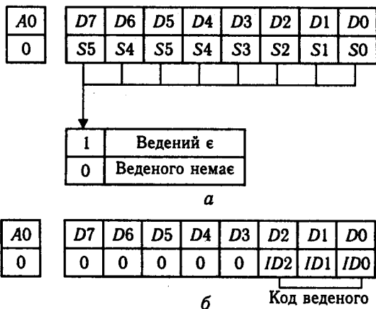
Рис. 5.60. Формати керуючих слів ініціалізації ICW3: а – для ведучого ПКП; б – для веденого
