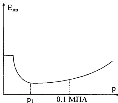
Рисунок 5.3 – Залежність електричної міцності газу від тиску
