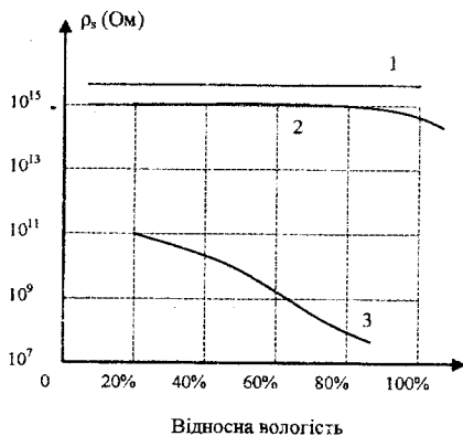
Рисунок 3.5 – Залежність питомого поверхневого опору від відносної вологості для різних типів діелектриків (1 – цезезин – неполярний діелектрик; 2 – віск бджолиний – полярний діелектрик; 3 – мармур – пористий матеріал, що має розчинні у воді домішки)
