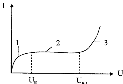
Рисунок 3.2 – Залежність струму в газі від напруги
