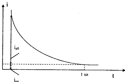
Рисунок 3.1 – Залежність струму через діелектрик від часу
