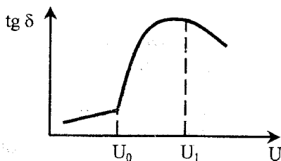
Рисунок 4.3 – Іонізаційна характеристика ізоляції
