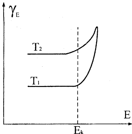
Рисунок 7.6 – Залежності питомої провідності напівпровідника від напруженості електричного поля при різних температурах навколишнього середовища ( T_1 > T_2 )
