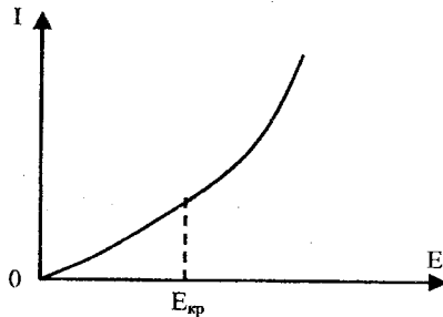
Рисунок 3.4 – Залежність струму від напруженості поля в рідких діелектриках
