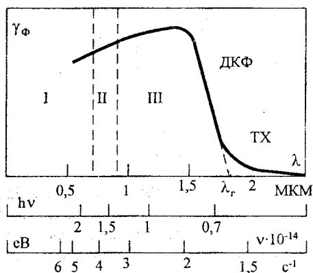
Рисунок 7.5 – Фотопровідність германія в залежності від довжини хвилі випромінювання (I – видима зона спектра, II – червона, III – інфрачервона, ДКФ – довгохвильовий край фотопровідності, ТХ – «теплі хвіст» кривої)
