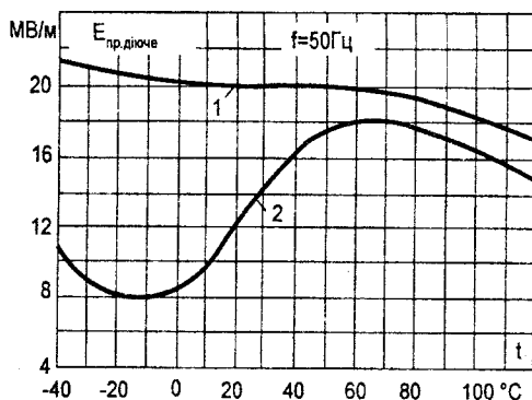
Рисунок 5.5 – Залежність електричної міцності трансформаторного масла від температури ( 1 – висушене масло; 2 – експлуатаційне масло)
