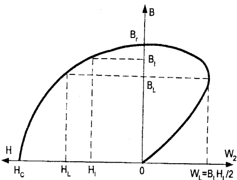
Рисунок 9.5 – Криві розмагнічування і магнітної енергії
