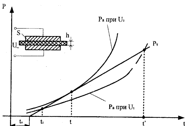
Рисунок 5.7 – Пояснення до розрахунку пробивної напруги при тепловому пробі
