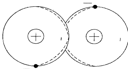
Рисунок 1.1 – Схематичне зображення двохатомної молекули з ковалентним зв'язком
