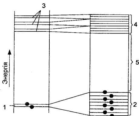
Рисунок 1.5 – Схема розташування енергетичних рівнів відокремленого атома (ліворуч) і неметалевого твердого тіла (праворуч) (1 – нормальний енергетичний рівень атома, 2 – заповнена електронами зона, 3 – рівні збудженого стану атома, 4 – вільна зона, 5 – заборонена зона)
