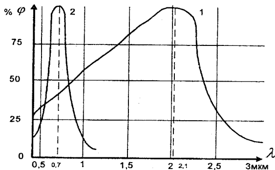
Рисунок 7.8 – Спектральна чутливість при 200 ^{\circ}\text{C} фоторезисторів з полікристалічного сірчастого свинцю (1) і сірчастого вісмуту (2)
