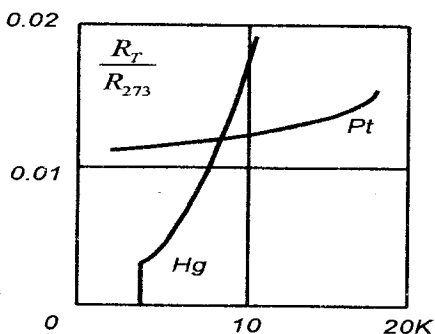
Рисунок 8.2 – Зміна опору зразків ртуті і платини при глибокому охолодженні
