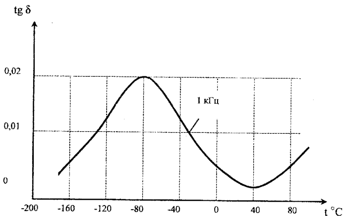
Рисунок 4.6 – Залежність \text{tg } \delta від температури для висушеного паперу
