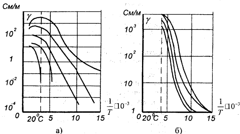
Рисунок 7.7 – Залежність питомої провідності декількох зразків n-Si (а) і p-Si (б) від температури
