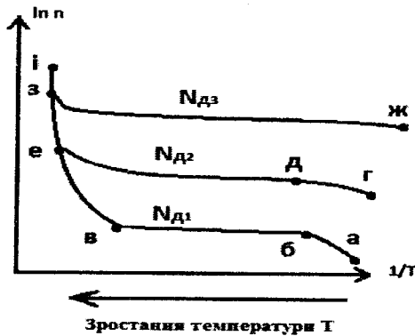
Рисунок 7.3 – Типові залежності концентрації носіїв заряду у напівпровіднику від температури при різних концентраціях донорних домішок ( N_{d1} < N_{d2} < N_{d3} )
