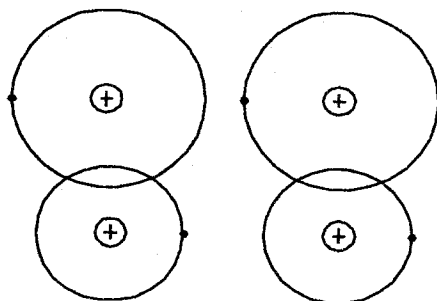
Рисунок 1.4 – Схематичне зображення двох взаємодійних молекул (зв'язок Ван-дер-Ваальса)
