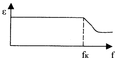
Рисунок 2.4 – Залежність діелектричної проникливості від частоти для полярної рідини
