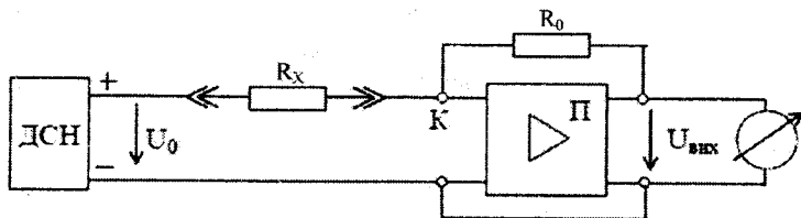
Рисунок 3.5 – Схема для вимірювання опорів у діапазоні (10^6 - 10^{14}) Ом
