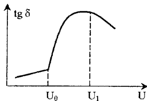
Рисунок 2.2 – Іонізаційна характеристика ізоляції
