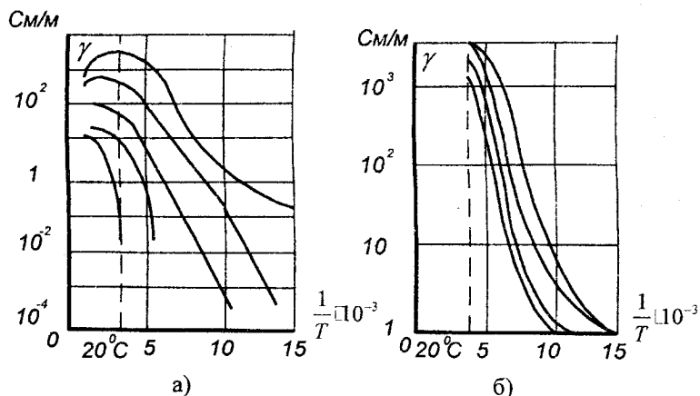
Рисунок 7.4 – Залежність питомої провідності декількох зразків n-Si (а) і p-Si (б) від температури
