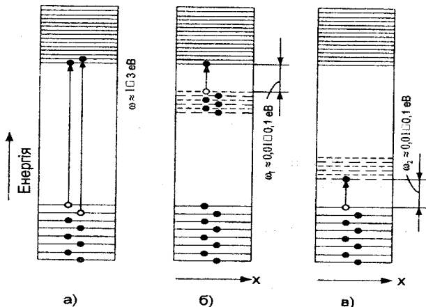
Рисунок 7.1 – Вплив домішок на енергетичну діаграму напівпровідників
