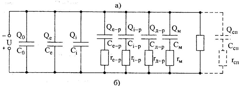
Рисунок 2.1 – Діелектрик складної сполуки з різними механізмами поляризації в електричному полі (а) та еквівалентна схема його заміщення (б).
