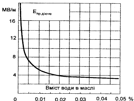
Рисунок 5.1 – Залежність електричної міцності від наявності води в трансформаторному маслі
