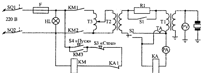
Рисунок 6.3 -- Електрична схема випробувальної установки
