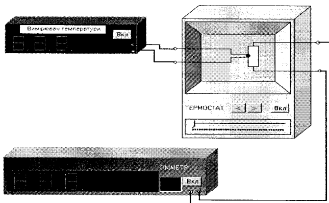
Рисунок 8.3 – Схема дослідної установки
