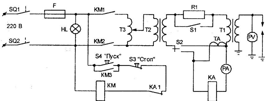
Рисунок 4.3 – Електрична схема випробувальної установки
