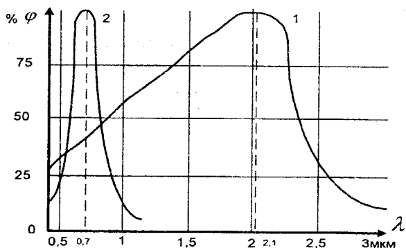
Рисунок 7.5 – Спектральна чутливість при 20^{\circ}\text{C} фоторезисторів з полікристалічного сірчистого свинцю (1) і сірчистого вісмуту (2)
