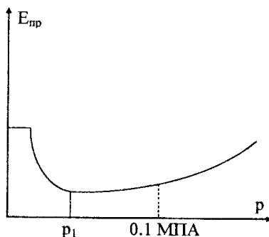
Рисунок 4.2 – Залежність електричної міцності газу від тиску
