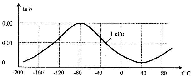
Рисунок 2.4 – Залежність \text{tg } \delta від температури для висушеного паперу
