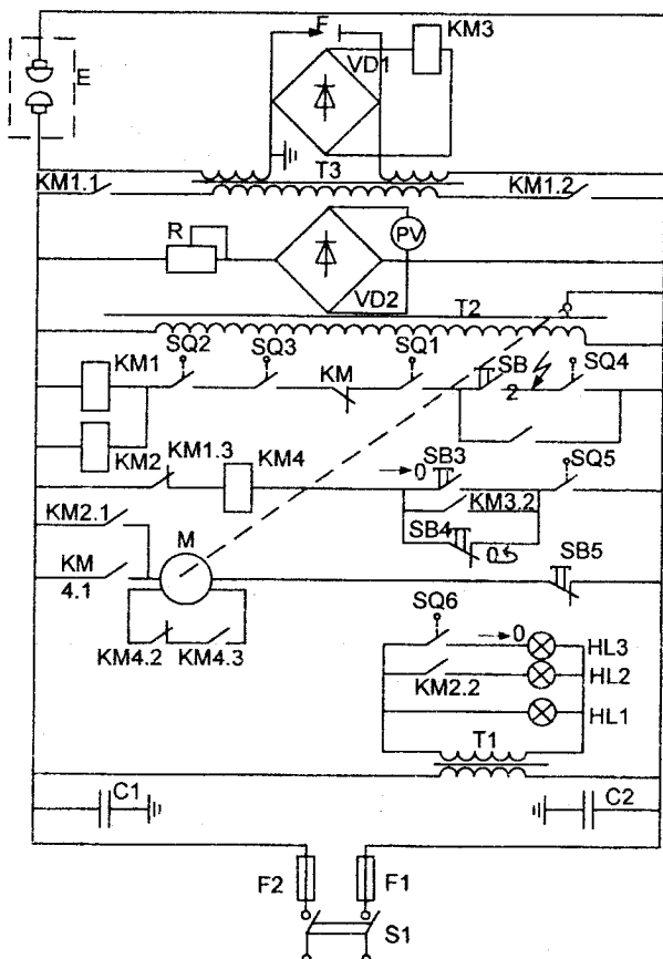
Рисунок 5.4 – Принципова електрична схема апарата АИМ-80
