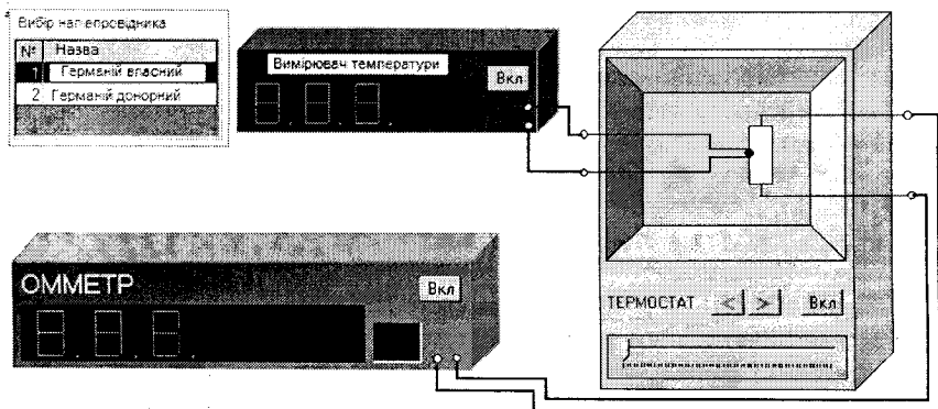
Рисунок 7.6 – Схема дослідної установки
