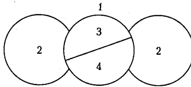
Рис. 7.3. Иллюстрация к задаче о четырех красках
