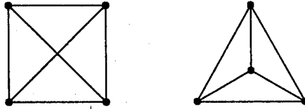
Рис. 10.7. Планарный граф и его укладка
