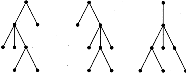
Рис. 9.8. Диаграммы деревьев
