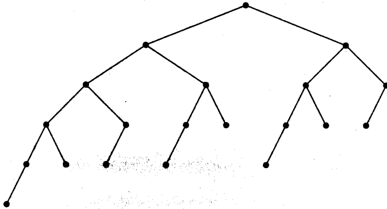
Рис. 9.14. Сбалансированное дерево
