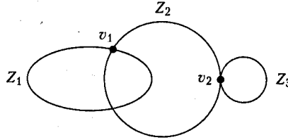
Рис. 10.4. К доказательству теоремы 10.2.1
