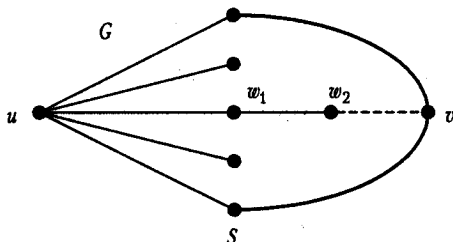
Рис. 8.5. К доказательству теоремы Менгера, случай 3
