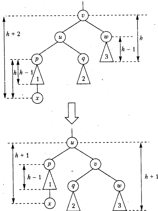
Рис. 9.15. Простое вращение
