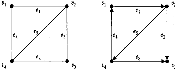
Рис. 7.10. Диаграммы графа (слева) и орграфа (справа), используемых в качестве примеров
