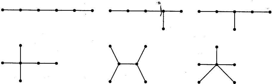
Рис. 9.2. Свободные деревья с 6 вершинами
