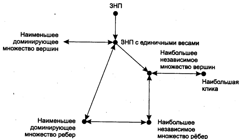
Рис. 10.6. Связь различных задач
