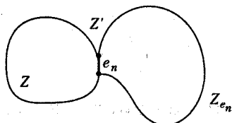
Рис. 10.1. К доказательству теоремы 10.1.2
