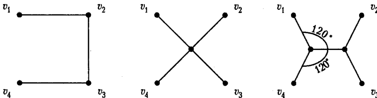
Рис. 9.18. Кратчайший остов, приближённое и точное решение задачи Штейнера
