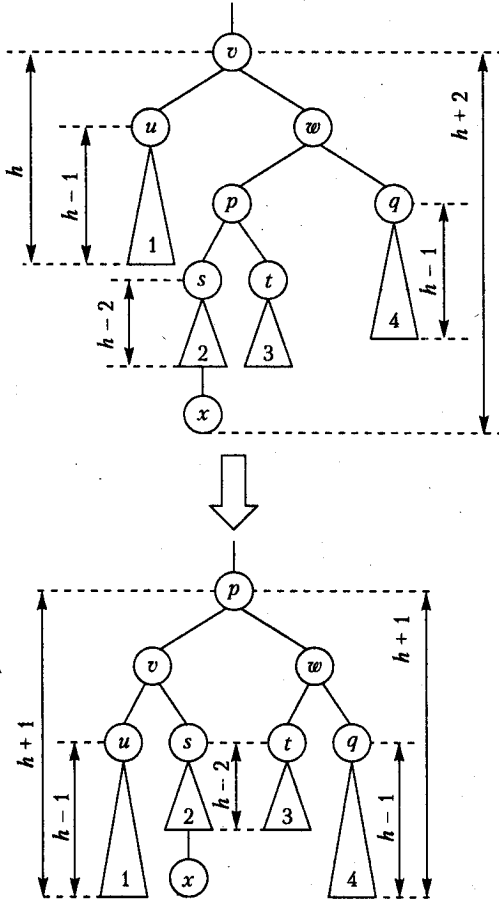
Рис. 9.16. Двойное вращение
