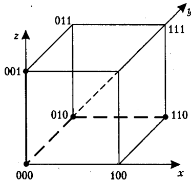
Рис. 3.1. Представление булевой функции в виде гиперкуба
