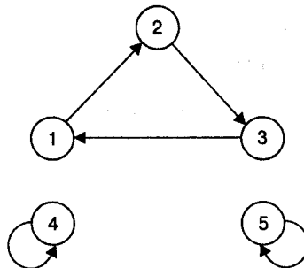
Рис. 5.1. Графическое представление перестановки
