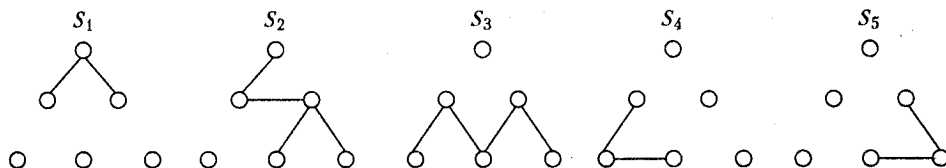
Рис. 10.3. Фундаментальные разрезы
