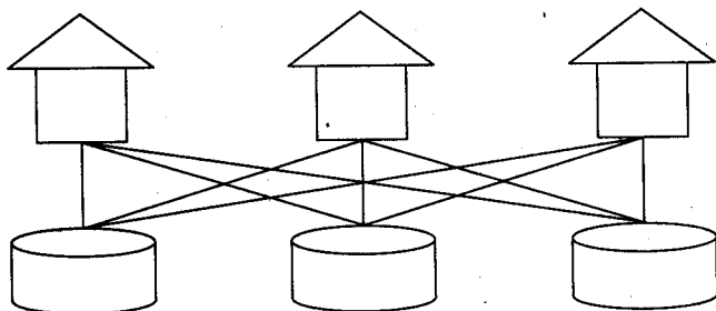
Рис. 7.2. Иллюстрация к задаче о трех домах и трех колодцах
