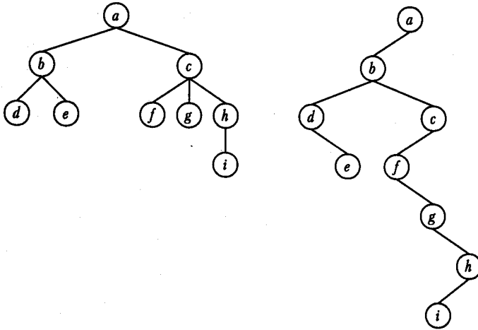
Рис. 9.11. Упорядоченное и бинарное деревья
