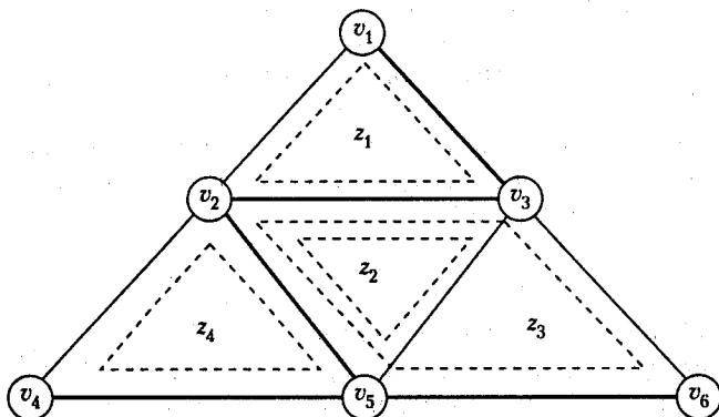
Рис. 10.2. Фундаментальные циклы
