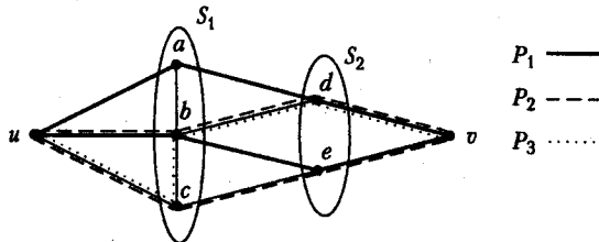
Рис. 8.2. Вершинно-непересекающиеся пути и разделяющие множества вершин
