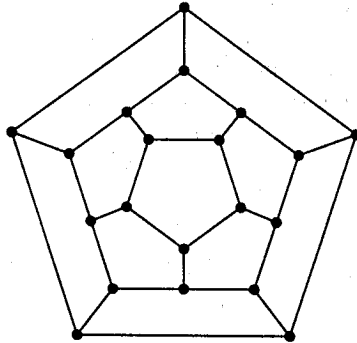
Рис. 10.5. Задача «Кругосветное путешествие»
