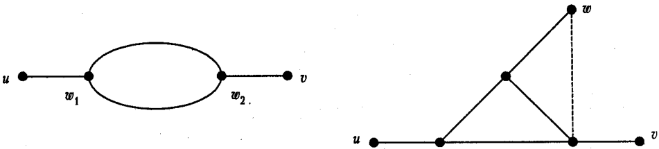
Рис. 9.3. К доказательству теоремы о свойствах деревьев
