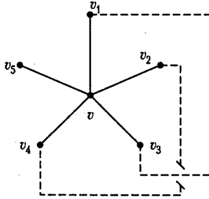
Рис. 10.8. К доказательству теоремы о пяти красках
