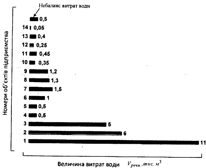
Рисунок А.4 – Баланс використання води на підприємстві
