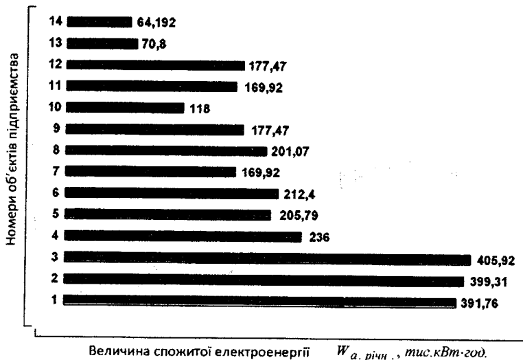
Рисунок А.3 – Баланс використання електроенергії на підприємстві
