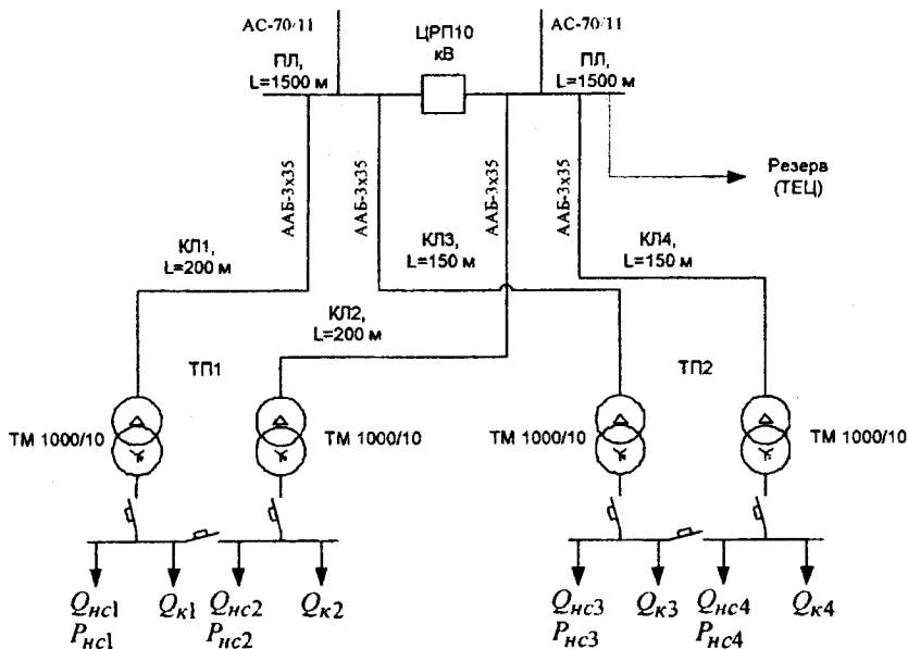
Рисунок А.6 – Однолінійна схема системи електропостачання підприємства
