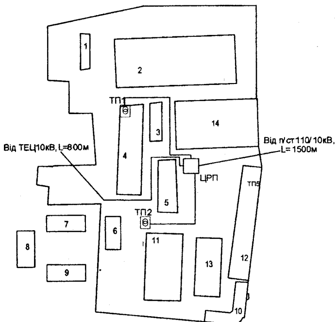
Рисунок А.1 – Генеральний план підприємства
