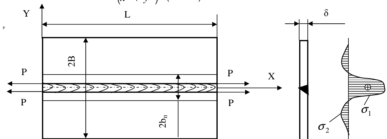
Рис.4.16. Схема попереднього розтягу листів
