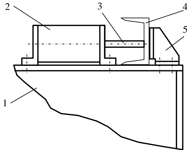
Рис.7.24. Пневмопритискач прямої дії: 1-рама стенда; 2-пнеumoциліндр; 3-шток; 4-заготовка; 5-упор.
