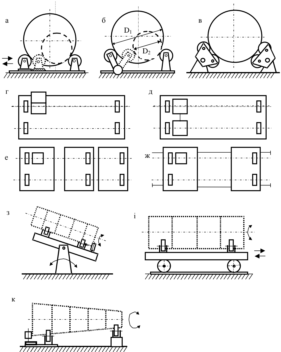
Рис. 8.26. Типові схеми роликів стендів: а- з переставними роликотопорами; б- з перекидними роликотопорами; в- з балансирними роликотопорами; г- на загальній рамі з одним поздовжнім валом; г'- на загальній рамі з двома поздовжніми та поперечним приводними валами; д- стаціонарний з окремих секцій; е- з пересувними секціями; е'- нахильюваний; ж- пересувний; з- для кінцевих виробів з упорним роликом.
