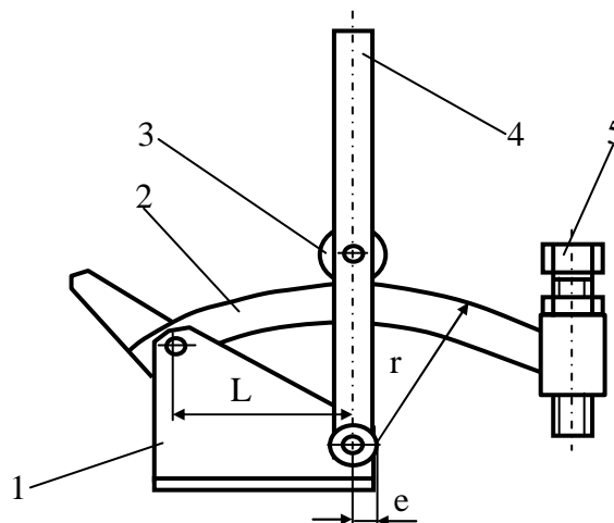
Рис. 7.12. Ексцентриковий притискач з великим робочим ходом (дуговий притискач): 1-корпус; 2-дуга; 3-ролик; 4-рукоятка; 5-гвинт регулювальний.
