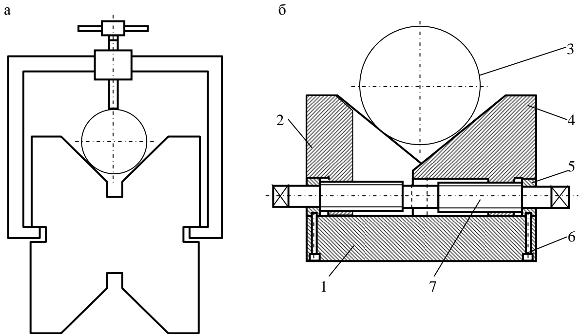
Рис.6.12. Типи призми: а-жорстка; б- регульована; 1-основа; 2,4-щока; 3-виріб; 5-опора; 6-гвинт стопорний; 7-гвинт регулювальний.
