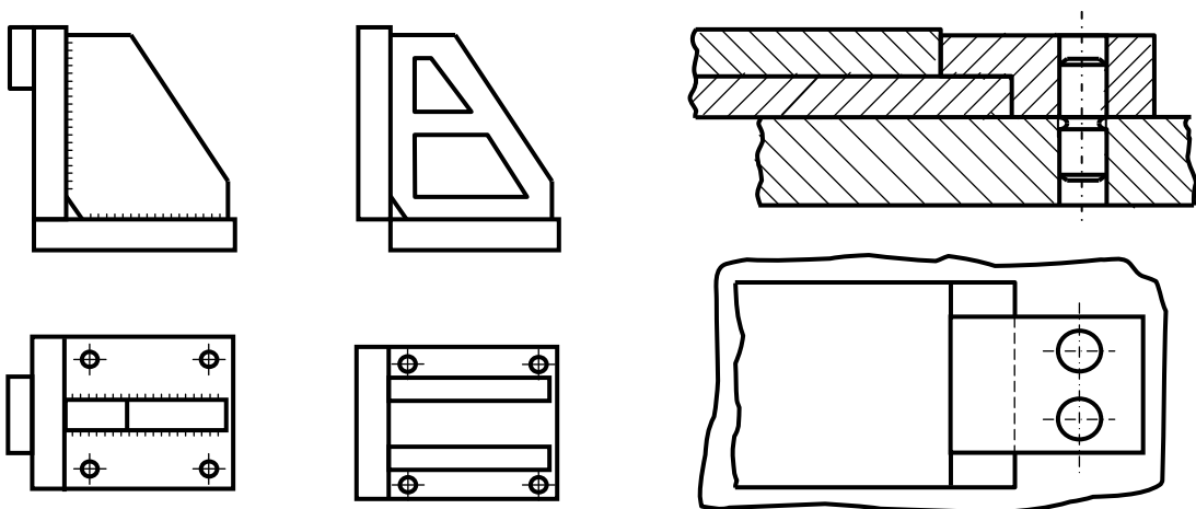
Рис.6.3. Знімні упори
