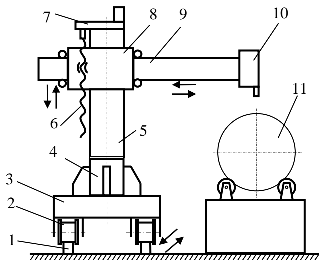
Рис. 9.6. Глагольний візок: 1 – рейка; 2 – каток; 3 – платформа; 4 – основа; 5 – стаяк; 6 – гвинт ходовий; 7 – редуктор; 8 – каретка; 9 – штанга висувна; 10 – зварювальний апарат; 11 – виріб.
