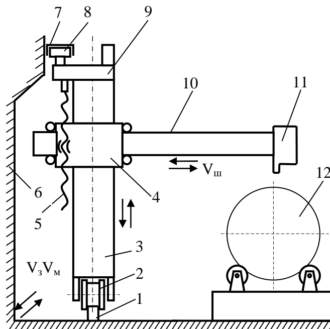
Рис. 9.4. Візок велосипедний для несамохідних зварювальних апаратів: 1 – рейка на підлозі цеху; 2 – каток візка; 3 – стаяк; 4 – каретка; 5 – ходовий гвинт; 6 – колона цеху; 7 – напрямна верхня; 8 – ролик; 9 – редуктор; 10 – консоль висувна; 11 – несамохідний зварювальний апарат; 12 – зварюваний виріб.
