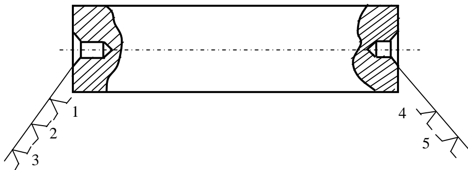
Рис. 2.10. Схема базування вала по центровим отворах
