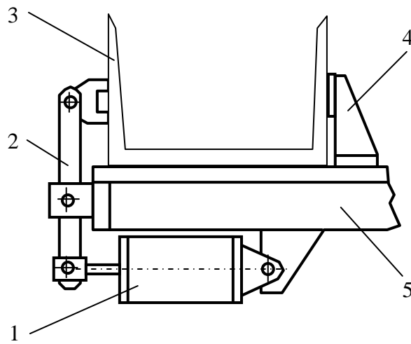
Рис.7.25. Пневмоважільний притискач: 1-пнеumoциліндр; 2-важіль; 3-заготовка; 4-упор; 5-рама стенда.
