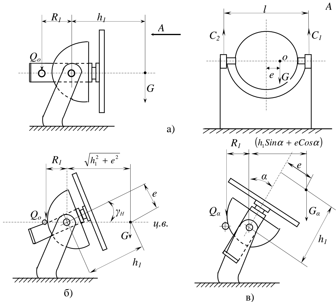
Рис.8.25. Розрахункові схеми механізму нахилення універсального обертача: а-горизонтальне положення при \alpha=90^\circ та \beta=0 ; б-нахилене положення під кутом \alpha=90^\circ - \gamma_H та \beta=90^\circ ; в-нахилене положення під довільним кутом \alpha .
