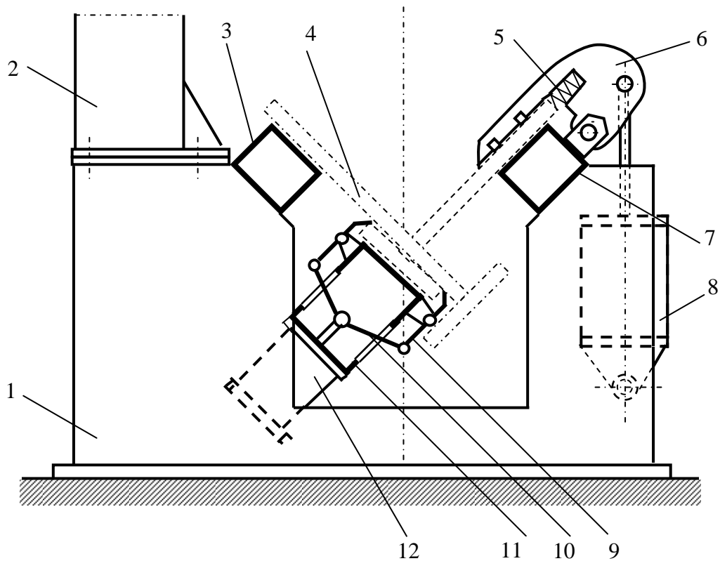
Рис. 3.12. Схема кондуктора-кантувача для складання і зварювання таврових балок: 1- станина; 2- колона для зварювального автомата; 3- ліва опорна балка; 4 – балка, що зварюється; 5- пружина; 6- верхній притискач; 7- права опорна балка; 8 – хитний гідроциліндр; 9- кліщовий захват; 10 - система ламких важелів; 11 - поворотна опорна балка; 12- пневмоциліндр.
