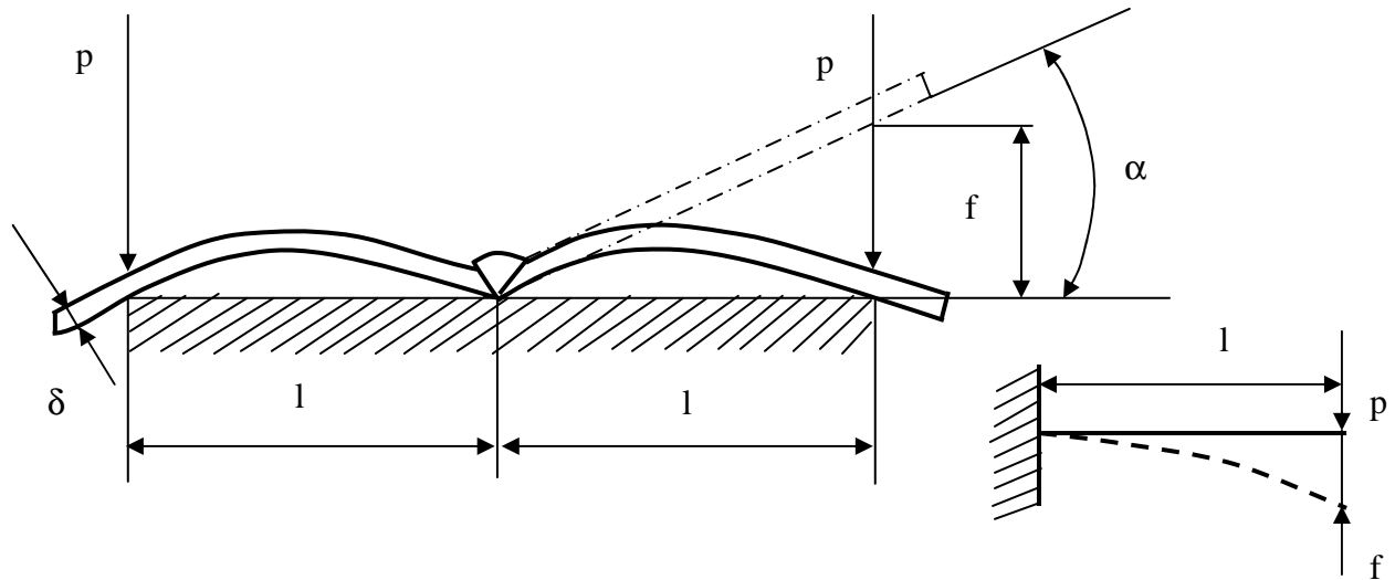
Рис. 4.2. Схема визначення сили притиску заготовок при куткових деформаціях
