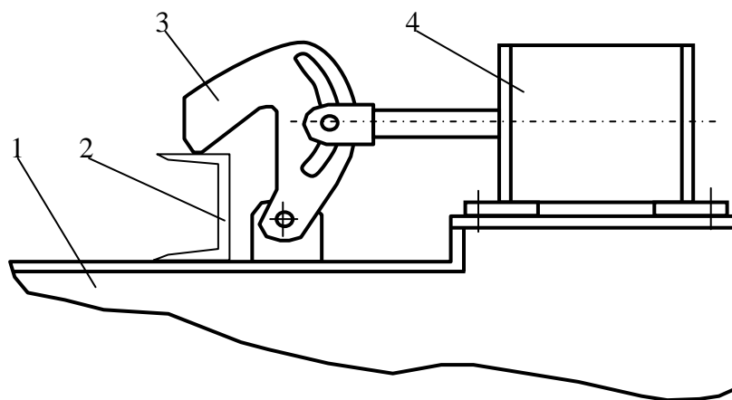
Рис.7.26. Пневмоважільний притискач: 1-рама стенда; 2-заготовка; 3-важіль; 4-пнеumoциліндр.
