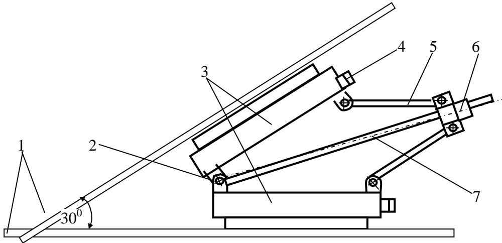
Рис.7.38. Універсальний електромагнітний притискач: 1-заготовки; 2-шарнір; 3-електромагніти; 4-вимикач; 5-шарнірна система; 6-гайка; 7-гвинт.
