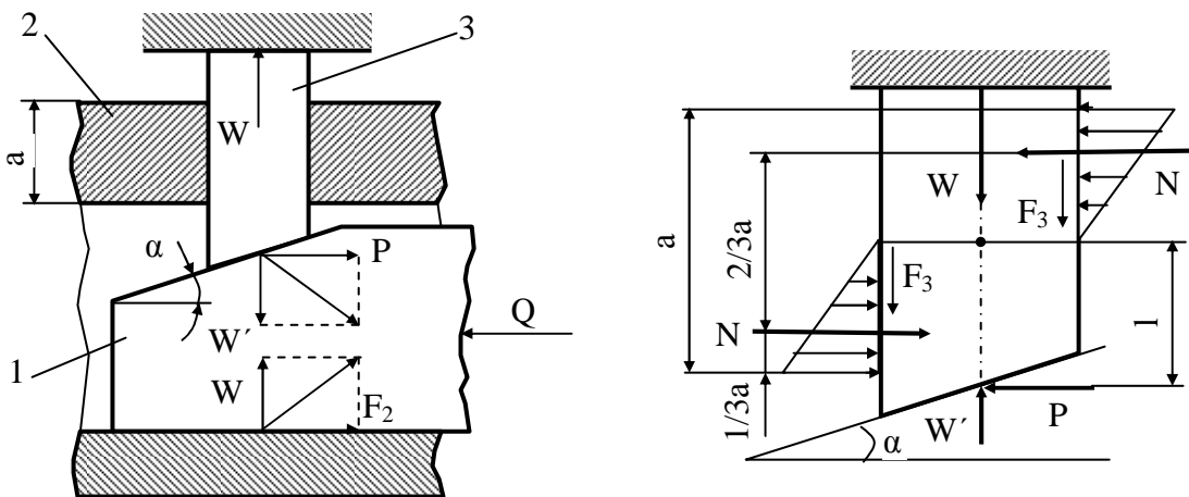
Рис. 7.21. Схема одноплунжерного клинового механізму: 1-односковий клин; 2-напрямна; 3- консольний плунжер.
