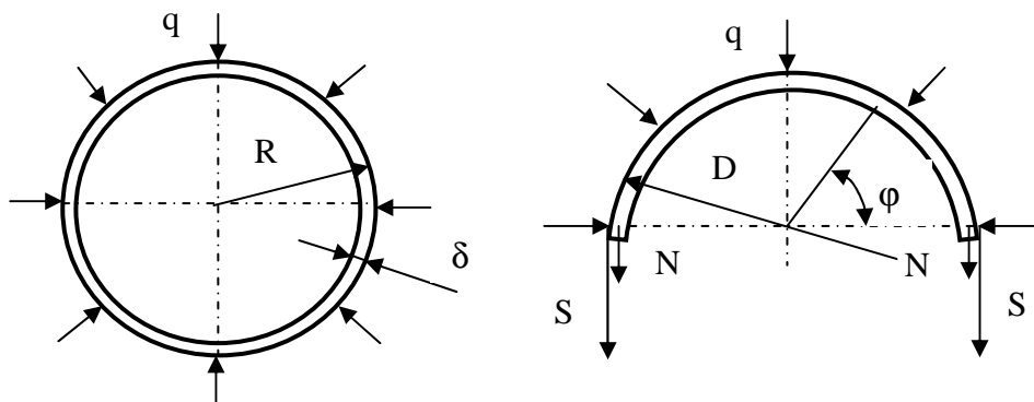
Рис. 4.14. Розрахункова схема навантаження обичайки зовнішнім центра тором
