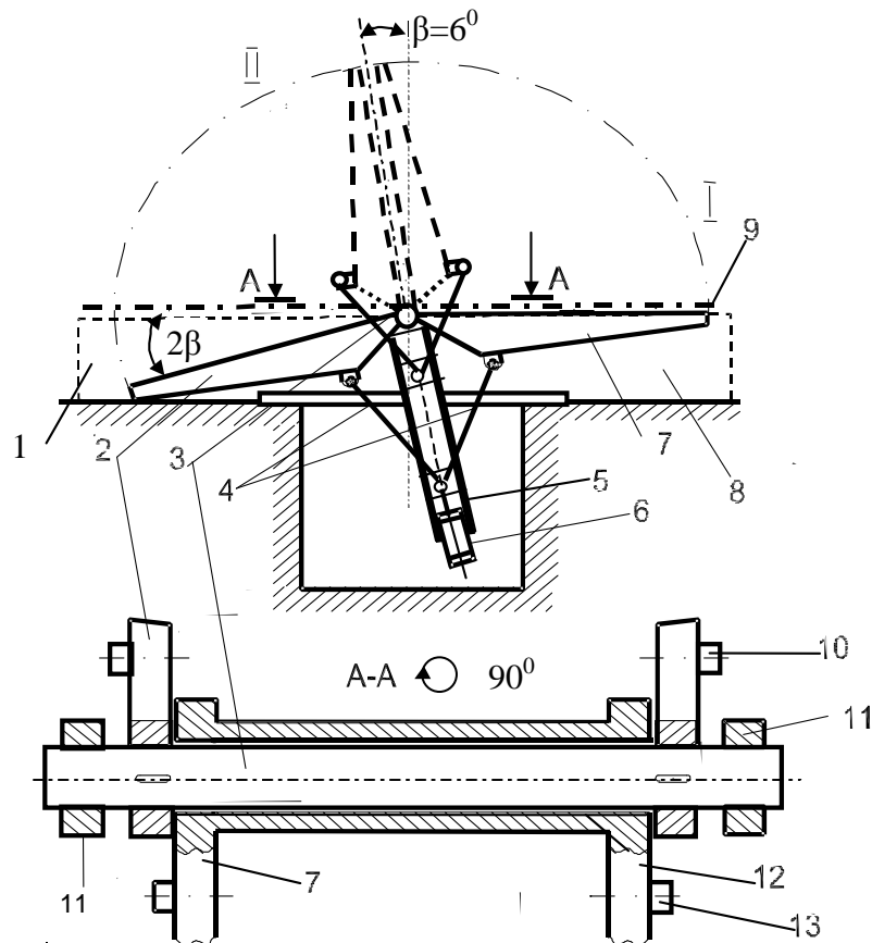
Рис. 8.17. Важільно-книжковий кантувач
