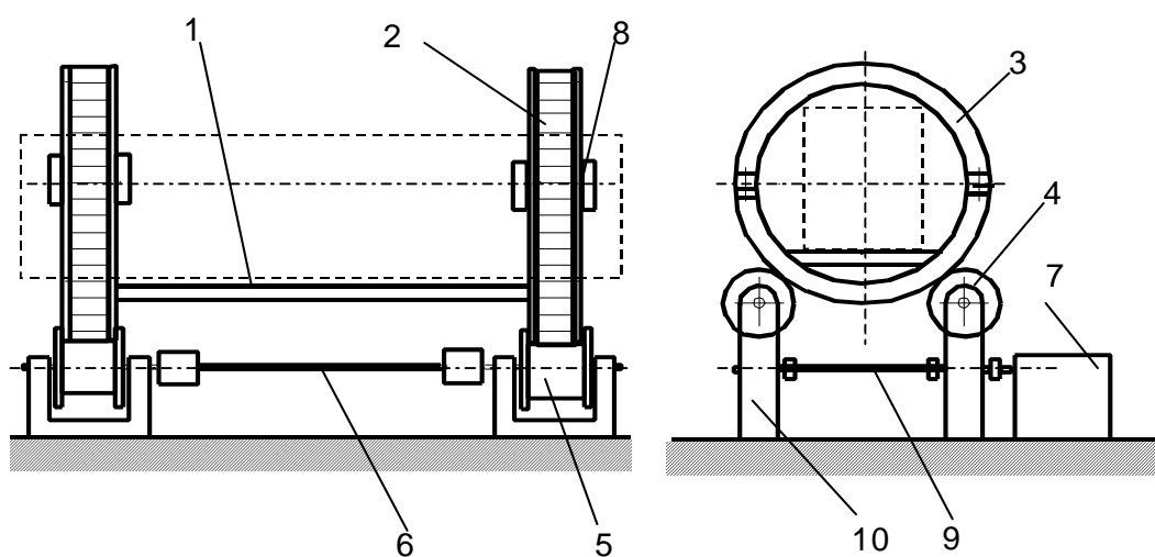
Рис. 8.10. Кільцевий кантувач
