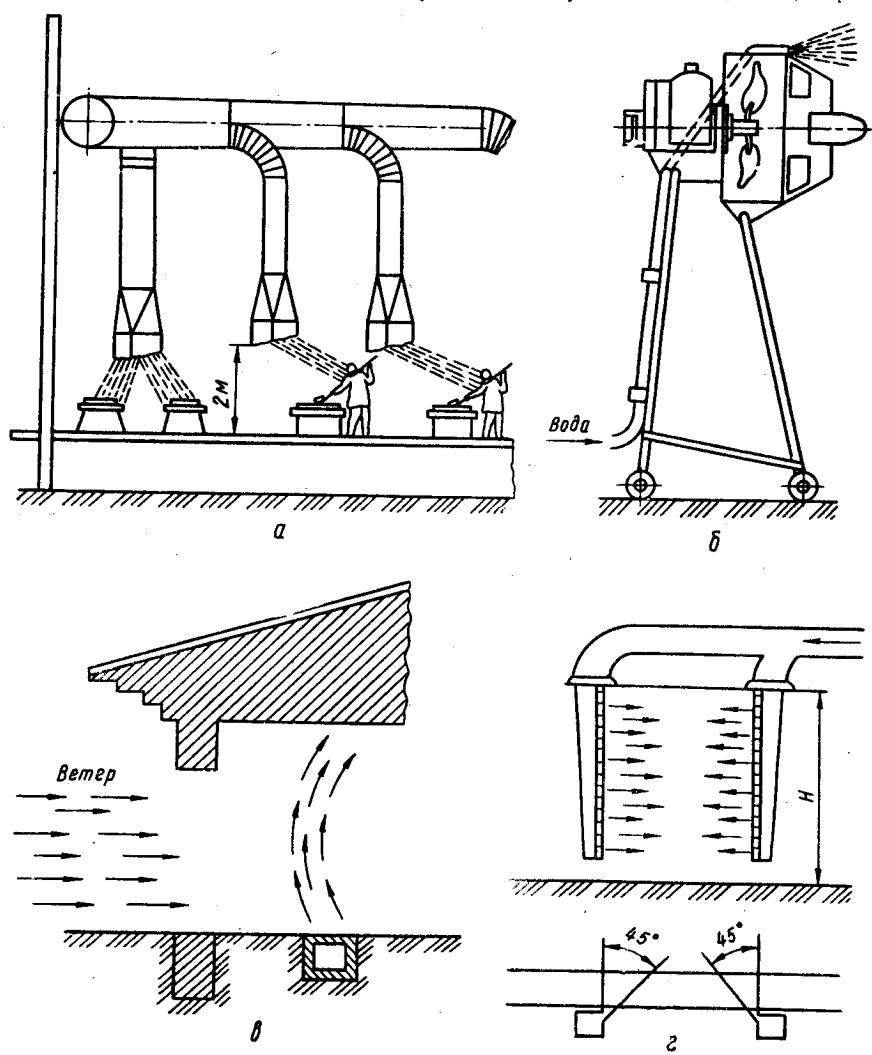
Рис. 3. Местная приточная вентиляция: а — стационарная установка воздушного душирования; б — передвижная установка водо-воздушного душирования; в — воздушная завеса с нижней подачей воздуха; г — воздушная завеса с боковой подачей воздуха.
