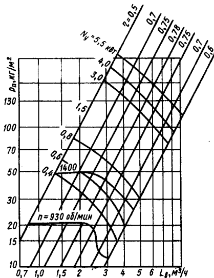
Рис. 8. Типовая рабочая характеристика вентилятора.
