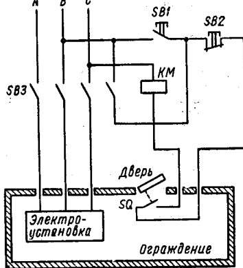
Рис. 46. Схема электрической блокировки.
