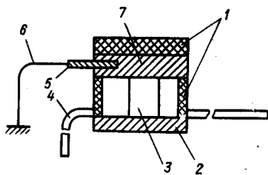
Рис. 25. Антистатический браслет.
