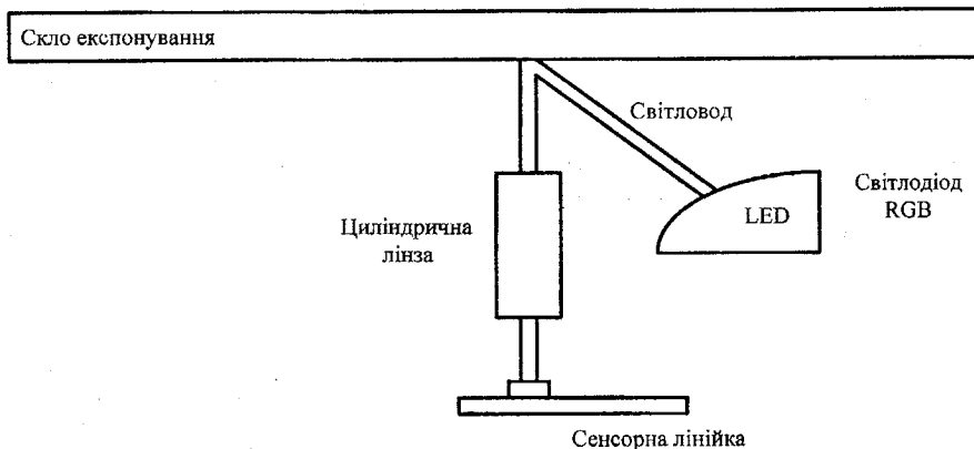
Рисунок 5.3 – Структура LIDE-сканера
