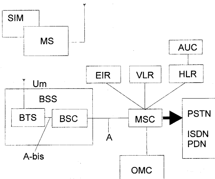
Рисунок 7.7 - Основні елементи мережі GSM
