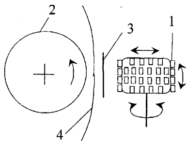
Рисунок 1.3 - Схема одержання відбитка на ДМ з кулькоподібною шрифтовою головкою
