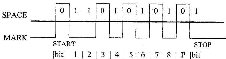
Рисунок 4.4 - Формат даних послідовного інтерфейсу
