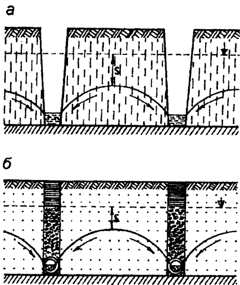
Рисунок 5.15 – Дренажні траншеї: а – відкриті; б – закриті
