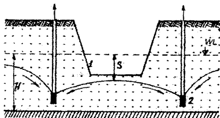
Рисунок 5.16 – Осушення будівельного котлована голкофільтрами: 1 – будівельний котлован; 2 – голкофільтри
