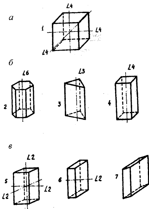
Рисунок 2.2 – Кристаліграфічні сингонії:
