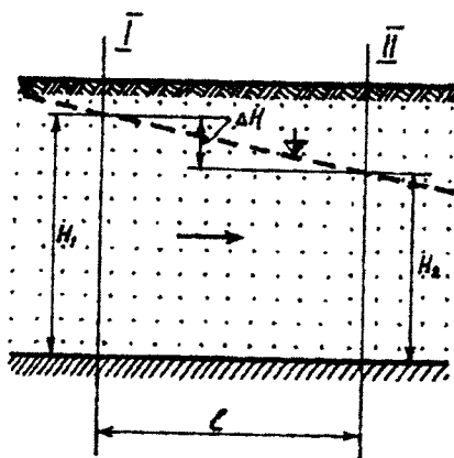
Рисунок 5.8 – Схема руху ґрунтової води
