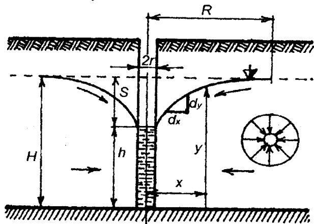
Рисунок 5.13 – Приплив води до досконалої свердловини:
