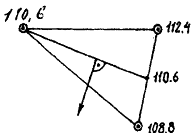
Рисунок 5.10 – Схема визначення напрямку руху ґрунтових вод
