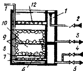
Рисунок 13.1 – Схема каркасно-засипного фільтра:
