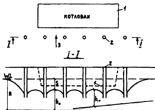
Рисунок 5.17 – Головний дренаж (план і розріз):
