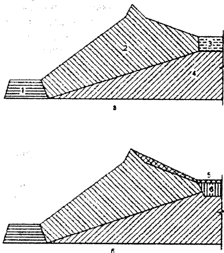
Рисунок 15.2 – Рекультивація гідровідвалу:
