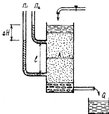
Рисунок 5.9 – Схема приладу для визначення коефіцієнта фільтрації пісків
