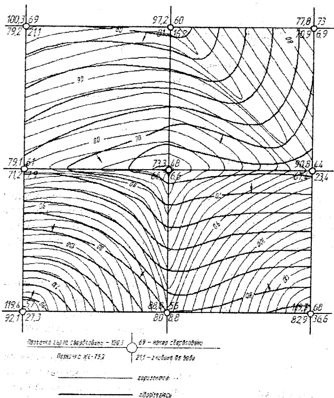
Рисунок 5.12 – Карта гідроізогіпс
