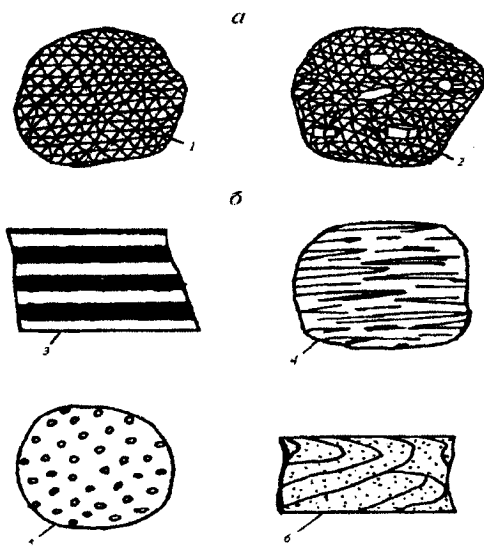
Рисунок 3.1 – Структура та текстура гірських порід:
