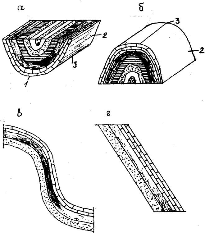
Рисунок 6.4 – Види складок: а – синклінальна; б – антиклінальна; в – флексура; г – монокліналь; 1 – замок; 2 – крило складки; 3 – вісь складки
