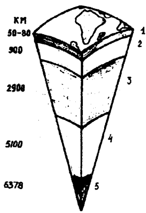
Рисунок 1.1 – Будова Землі:
