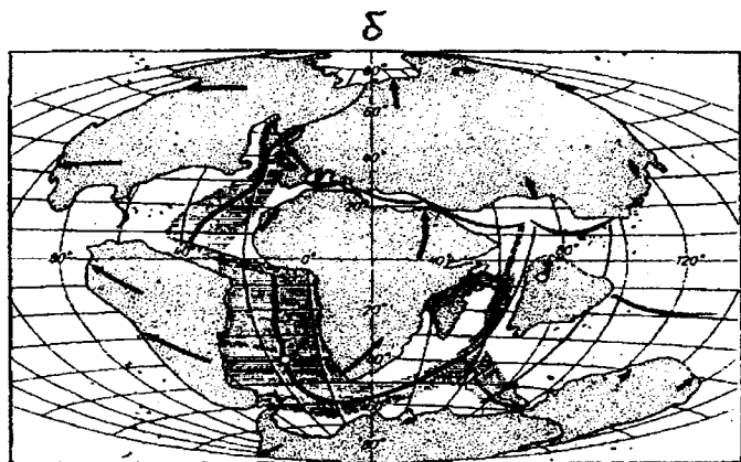
Рисунок 6.11 – Рух континентів:
