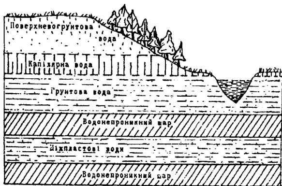
Рисунок 5.4 – Підземні води
