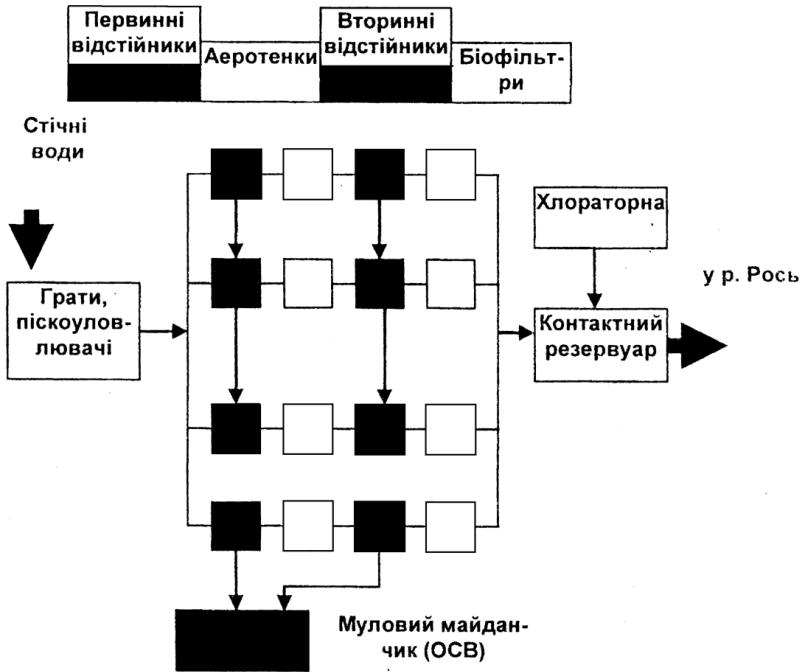
Рис. 4.2. Загальна схема станції очистки стічних вод м. Богуслава Київської області
