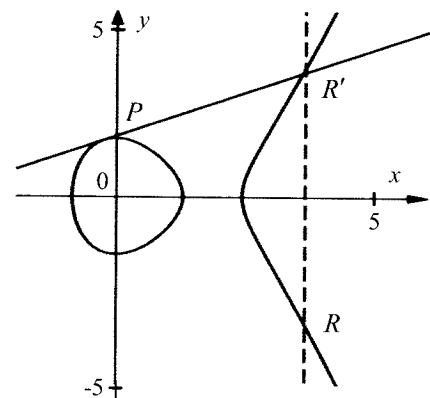
Рис. 2.18. Подвоєння точки R = P + P = [2]P
