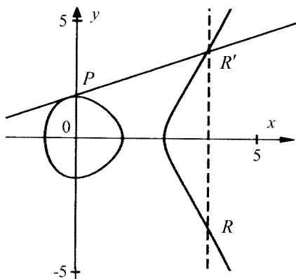
Рис. 2.18. Подвоєння точки R = P + P = [2]P
