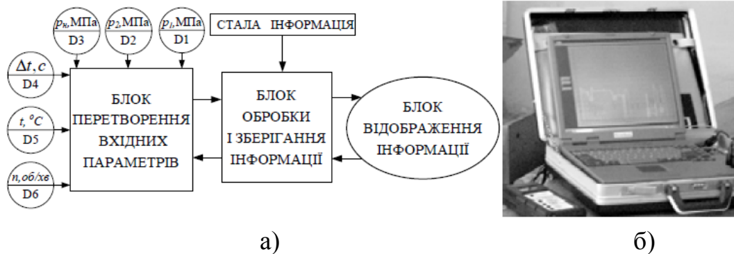
Рисунок 2.3 – Діагностичний комплекс для визначення параметрів гідросистеми: а – структурна схема комплексу, б – фотографія блоку відображення інформації
