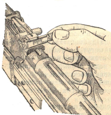
мал. 17. Установлення цілика на РКК-74.
