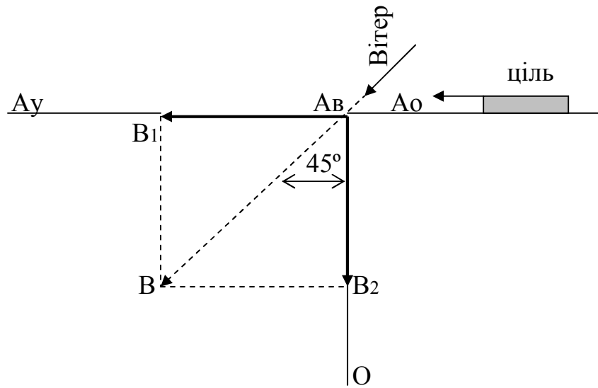
мал. 61 Схема розподілу швидкості вітру на складові O Av – напрямок стрільби; A0 Av Au – курс (напрямок руху) цілі; Av B – напрямок та швидкість вітру; Av B1 і Av B2 – складові швидкості вітру.
