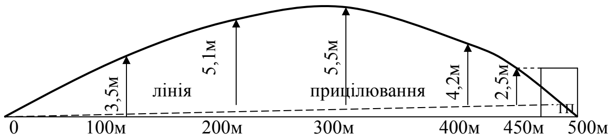
мал. 84. Перевищення траєкторії над лінією прицілювання (приціл 5)
