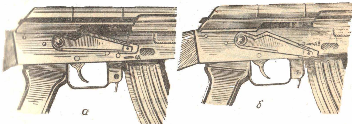
мал. 18. Установлення перевідника на необхідний вид вогню:
