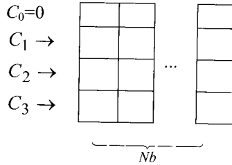
Рис. 3.23. Схема зсуву рядків стану
