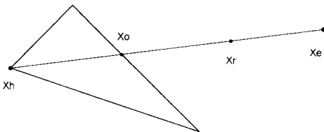
Операція розтягання
