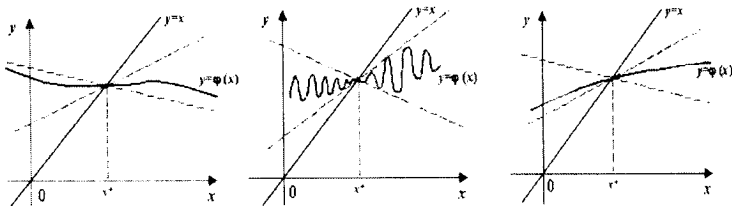
Рис КР.10.Графік перетинає пряму y=x під малим кутom: варіанти розташування.
