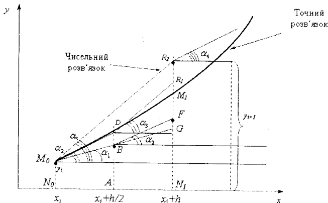
Рис.КР.35. Геометрична інтерпретація методу Рунге-Кутти.
