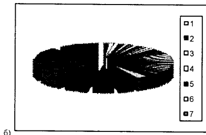
Рис. 2.22. Функція Пауела
