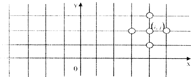
Рис. 1.5. Приклад методу сіток розв'язування задачі Коші для рівнянь гіперболічного типу
