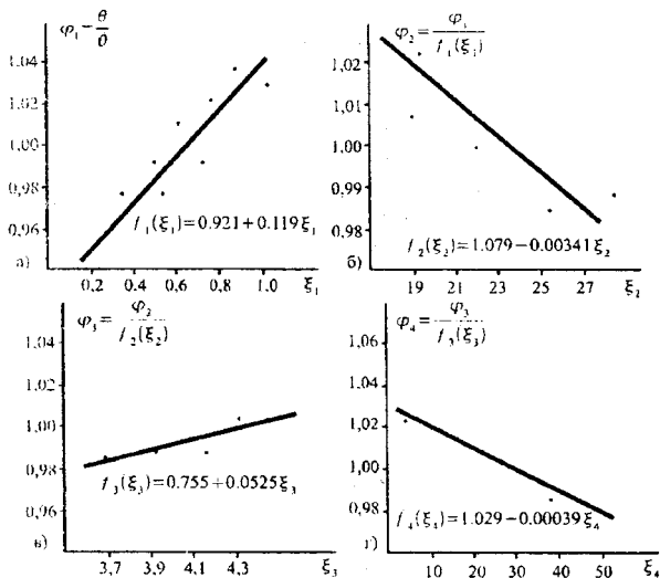
Рис. 3.7. Метод Брандона
