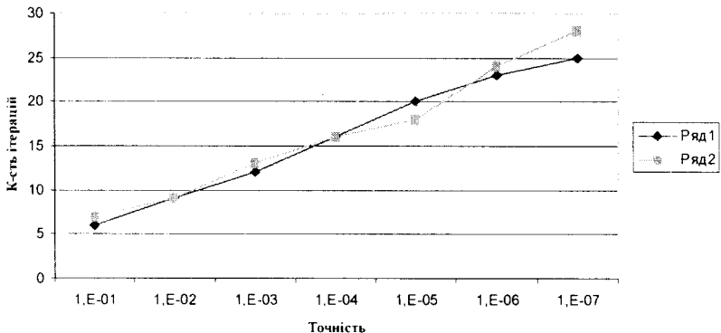
Рис. 2.30. Графічна інтерпретація отриманих результатів
