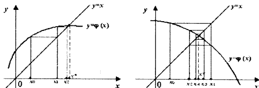
Рис. КР.11. Наближення, що збігаються до кореня у випадку |\varphi'(x)| < 1 .
