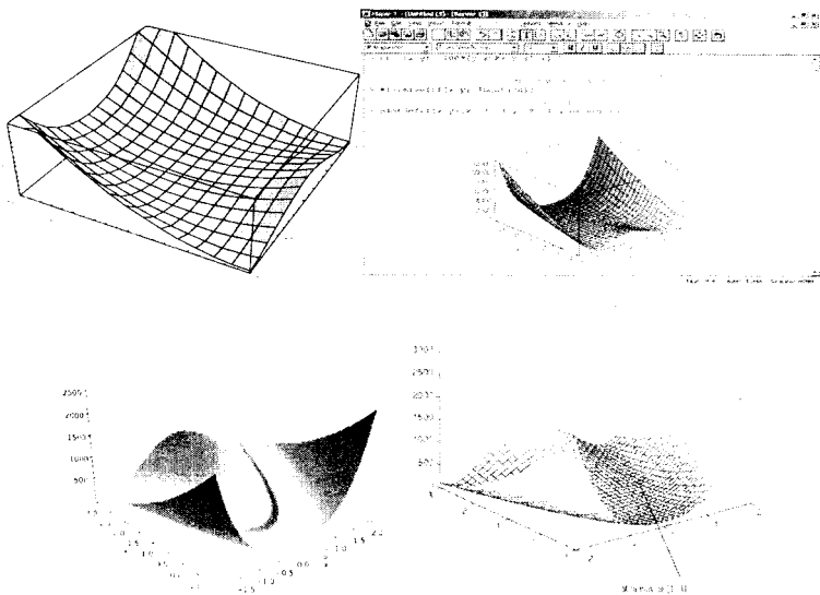
Рис. 2.21. Функція Розенброка
