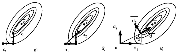
Рис. 2.29. Ефект яркості. а – зупинка в точці x_2 ; б – пошук продовжується паралельно до напрямку x_2-x_1 ; в – побудова нових напрямків пошуку в методі Розенброка
