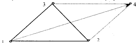
Рис. 2.34. Метод пошуку за симплексом
