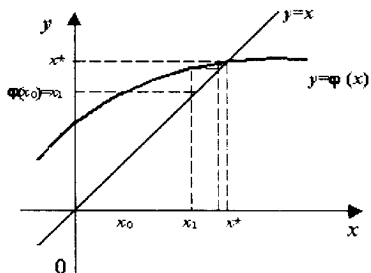
Рис. KP.9. Точка x^* – розв'язок рівняння x = \varphi(x) Побудова точки x_i по точці x_0
