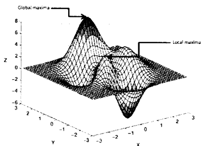
Рис. 2.23. Двовимірні експоненціальна функція
