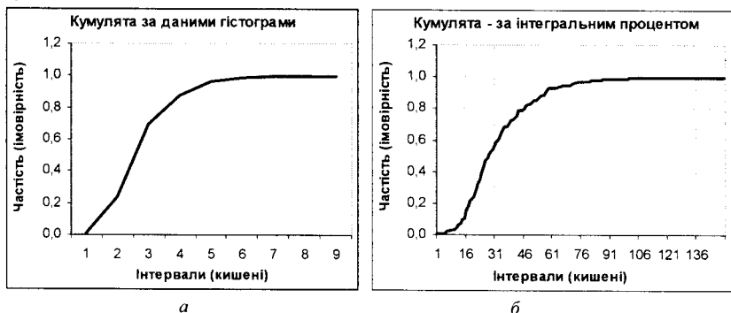
Рис. КП.4. Кумуляти побудовані: а – за даними гістограм; б – за інтегральним процентом.
