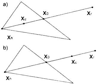
Рис. 2.26. Операції відбивання та розтягування
