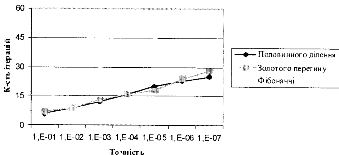
Рис. 2.12. Порівняння результатів оптимізації різними методами
