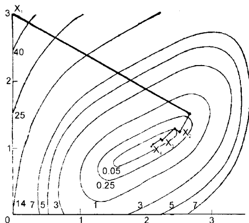
Рис. 2.31. Метод Девідона-Флетчера-Пауелла
