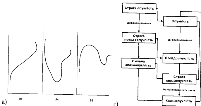
Рис. 2.19. Квазіопуклість та псевдоопуклість. а - функція квазіопукла та псевдоопукла; б - функція квазіопукла, але не псевдоопукла; в - функція не квазіопукла і не псевдоопукла г - зв'язок різних типів опуклості
