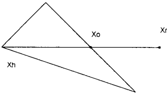
Операція відбивання
