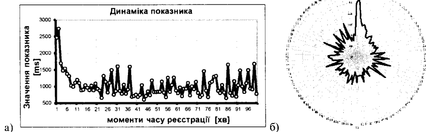
Рис. КП.1. Графічне подання динаміки показника: а – в декартовій системі координат, б – в полярній системі координат.
