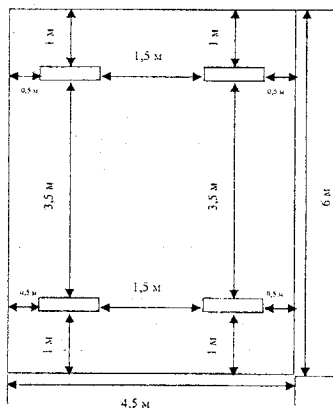
Рисунок 6.3 – Схема розміщення світильників [10]
