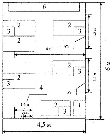
Рисунок 5.1 – Схема приміщення
