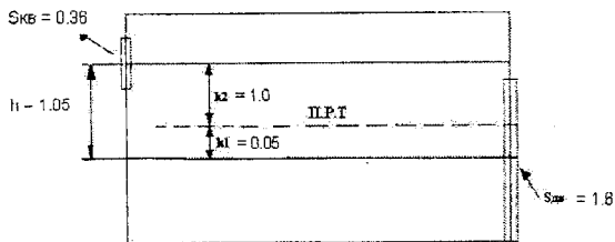
Рисунок 6.5 – Схема розрахунку природної вентиляції
