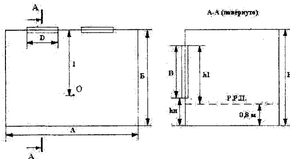
Рисунок 6.1 – Схема розрахунку природного освітлення
