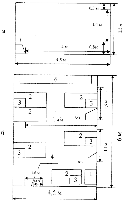
Рисунок 6.2 – Схема розрахунку природного освітлення де: а, б – вигляд збоку та зверху.
