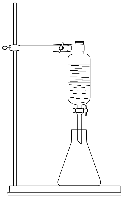
Рисунок 3.6 – Установка для вилучення речовин екстракцією
