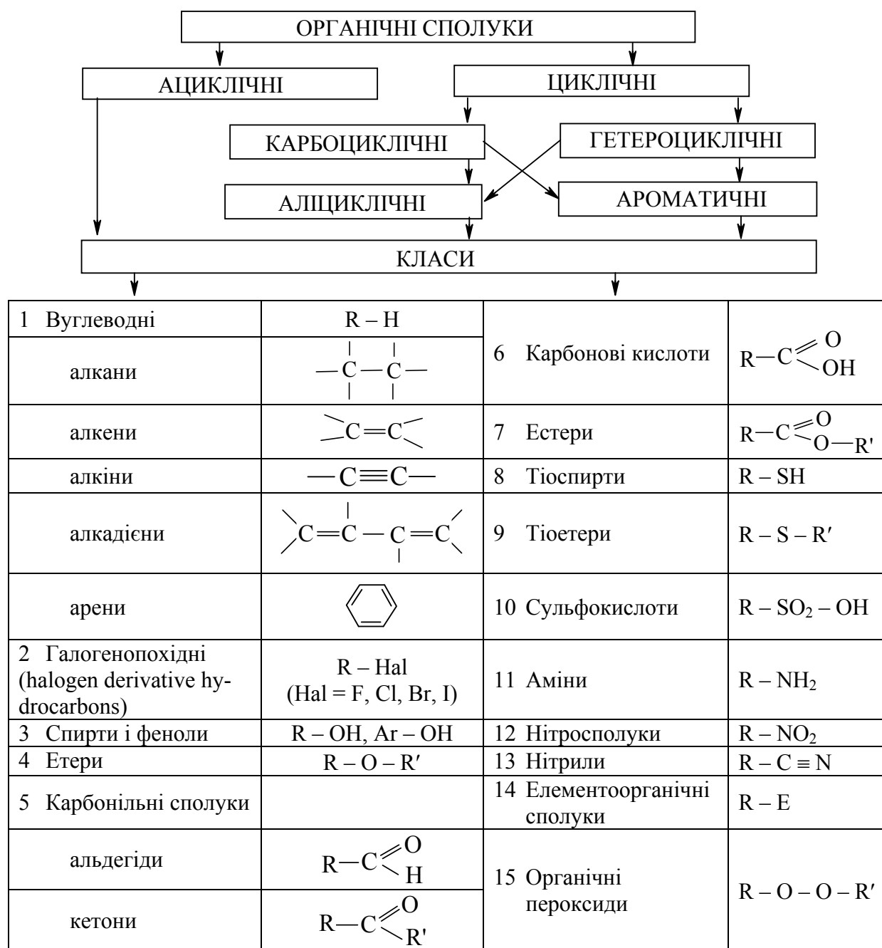
Рисунок 4.1 – Найважливіші класи органічних сполук за їх функціональними групами
