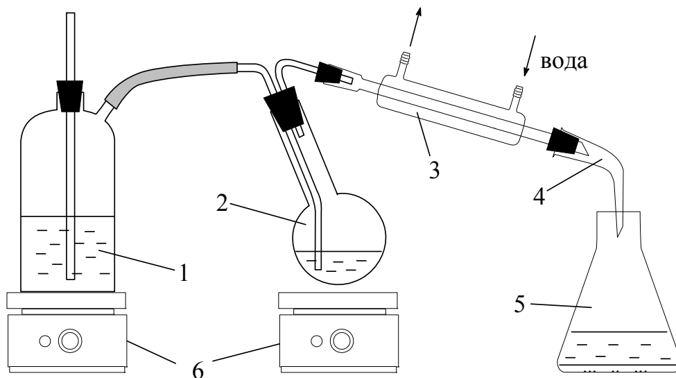
Рисунок 3.5 – Установка для перегонки з водяною парою
