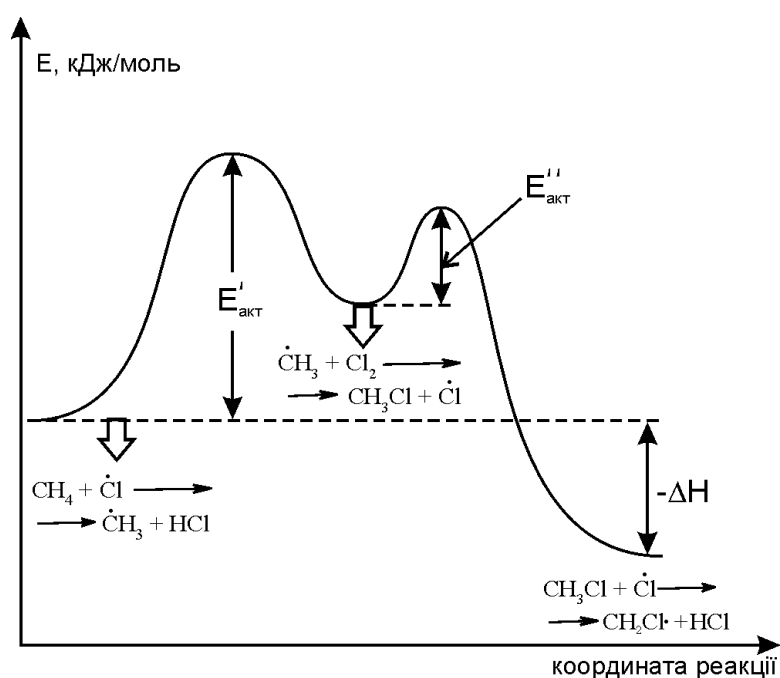
Рисунок 5.3 – Енергетична діаграма реакції хлорування метану
