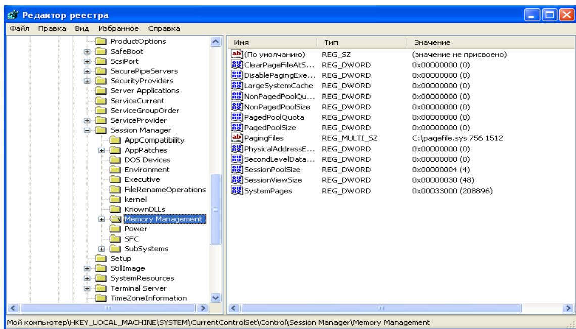
Рисунок 21 – Вікно очищення файла довантаження
