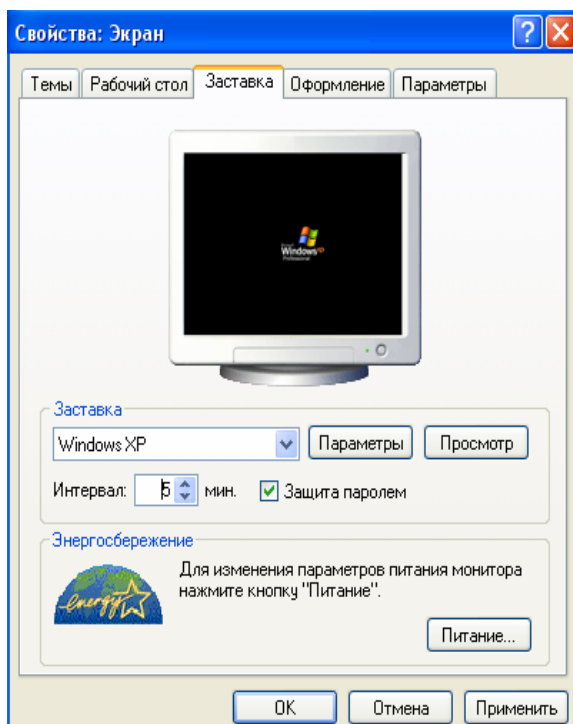
Рисунок 18 – Активізація програми-заставки
