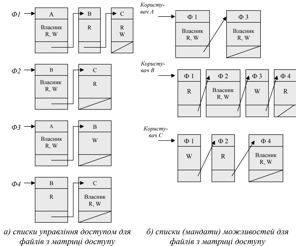
Рисунок 4 – Приклад структур управління доступом
