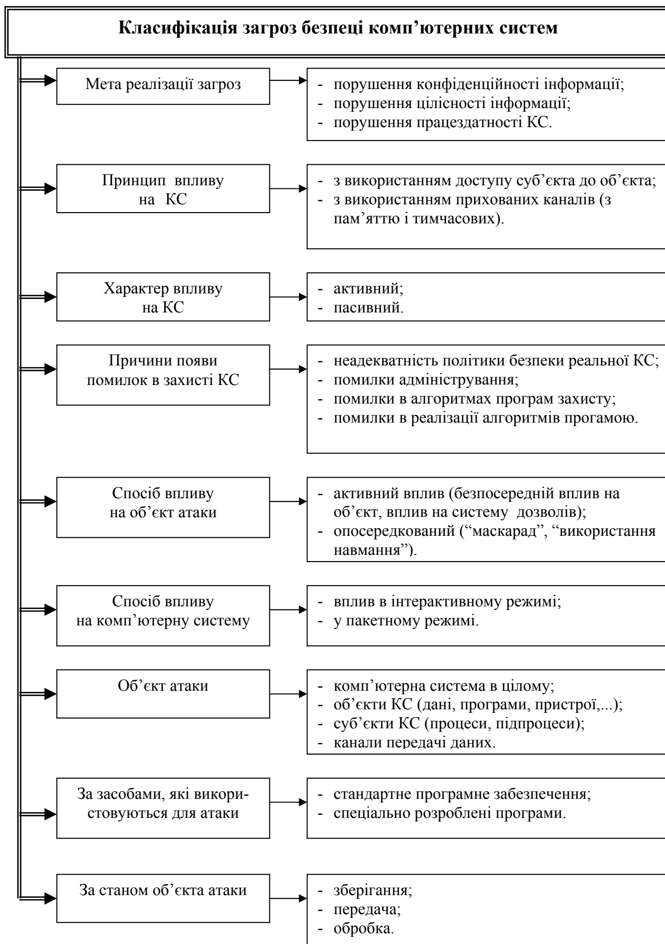
Рисунок 1 – Класифікація загроз безпеці комп'ютерних систем
