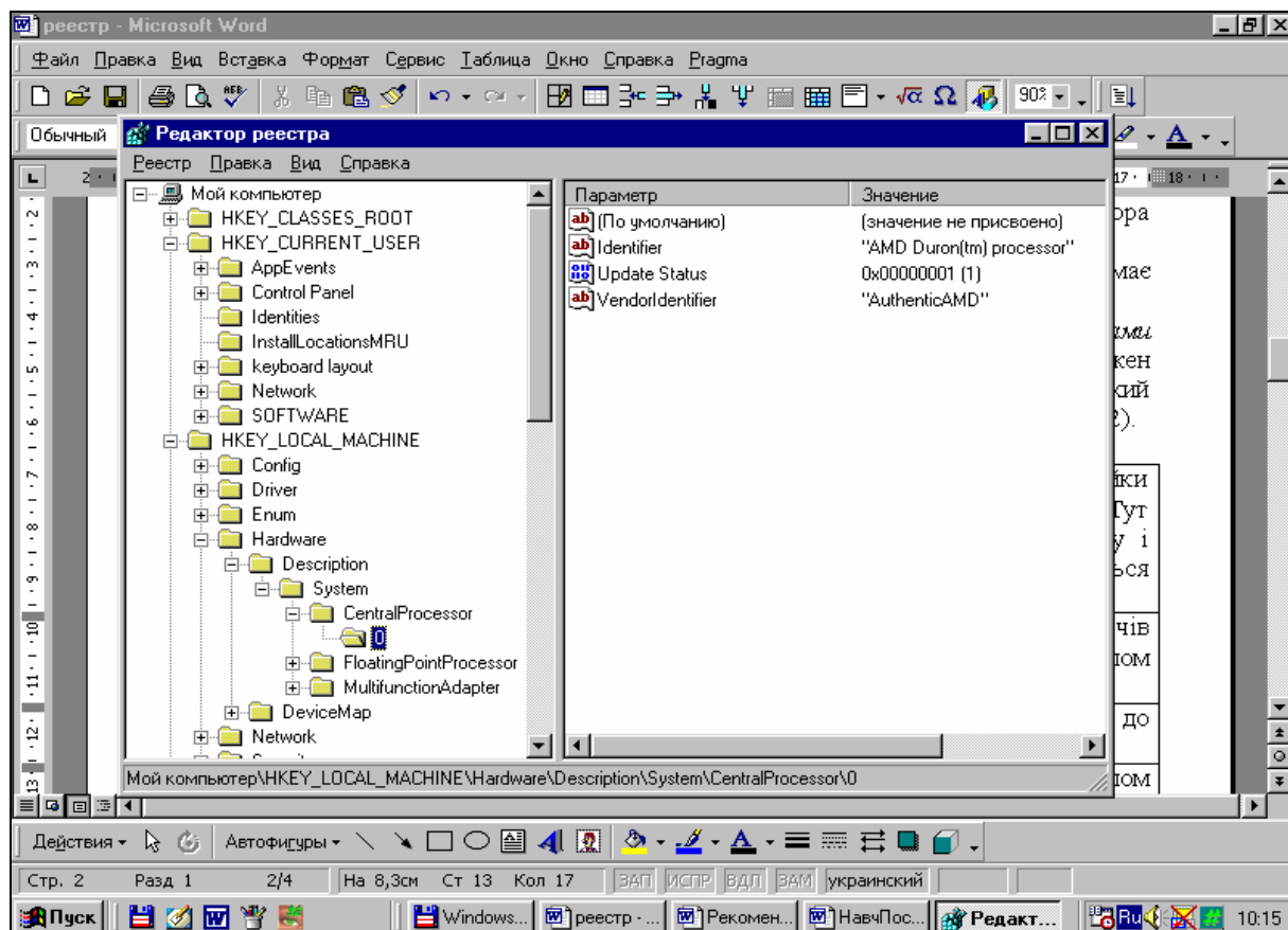
Рисунок 20 – Ієрархічна структура реєстру
