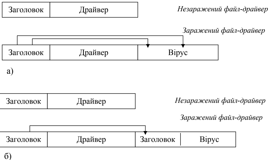
Рисунок 8 – Впровадження вірусу у SYS-файли
