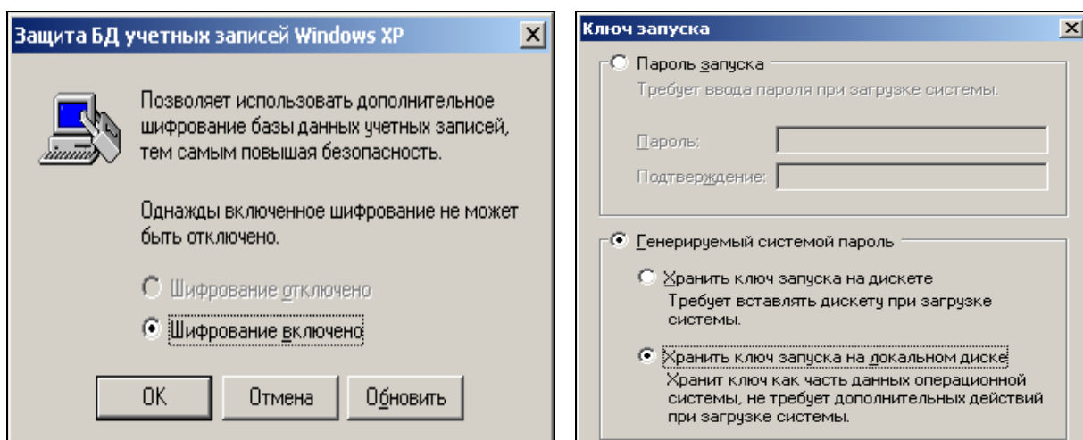
Рисунок 26 – Додаткове шифрування файла з паролями
