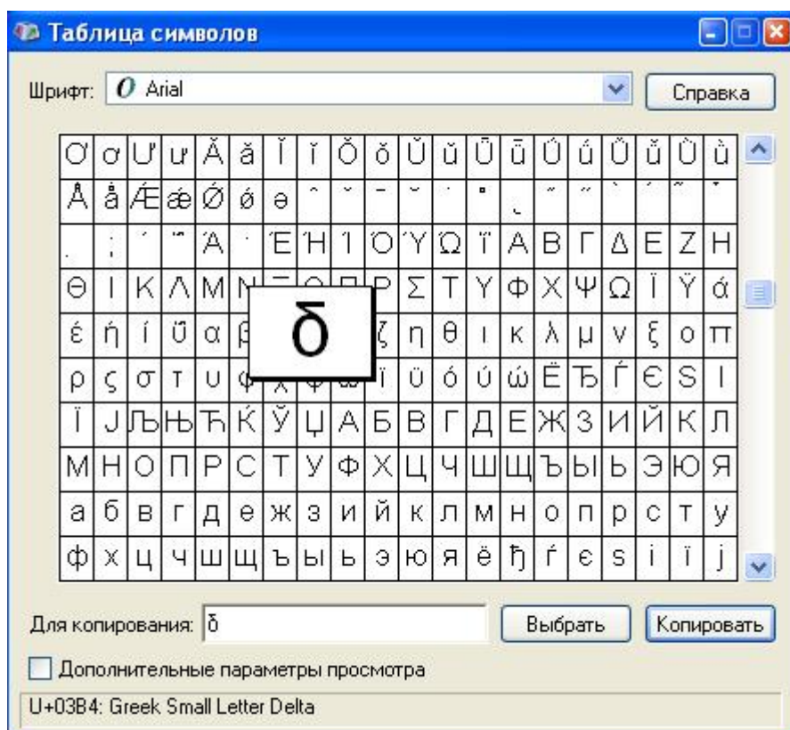
Рисунок 8.6 – Таблица символів
