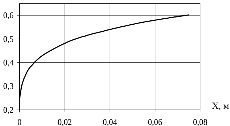
Рисунок 3.3 - Розрахункові значення відношення температурних напорів при значеннях параметрів : q = 7,6 \text{ кВт/м}^2 ; w_r = 0,052 \text{ м/с} ; t_p = 30^\circ\text{C}
