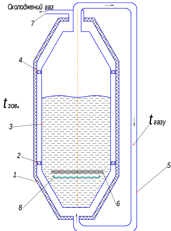
Рисунок 2.4 - Біогазовий реактор з утепленням корпусом
