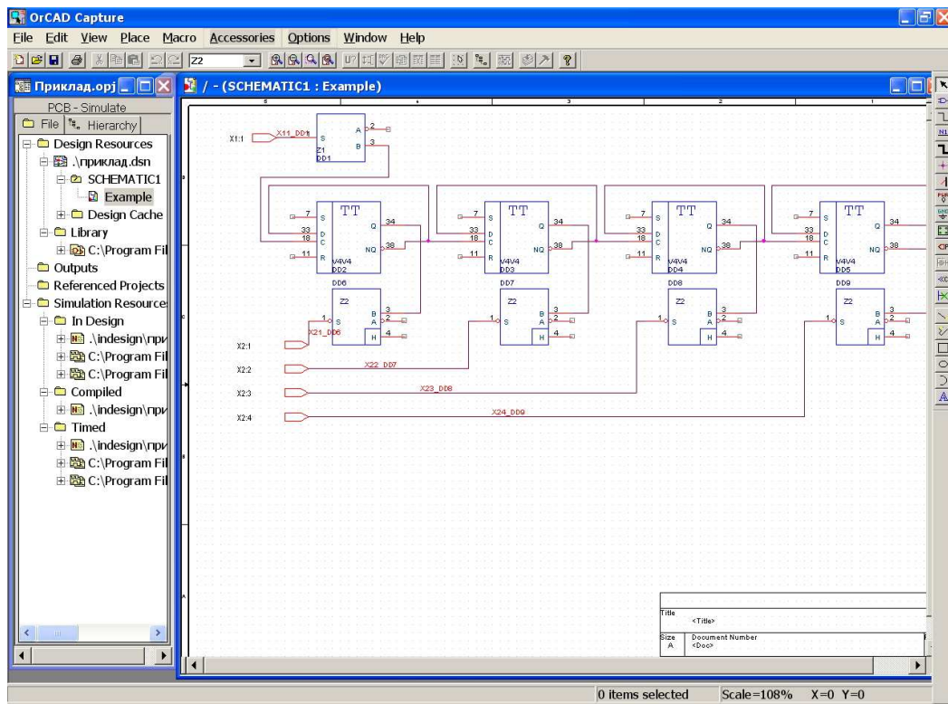
Рисунок 5.16 – Схема електрична принципова
