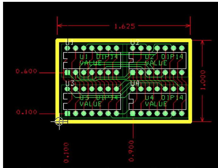
Рисунок 8.1 – Приклад трасування друкованої плати в "OrCAD Layout"
