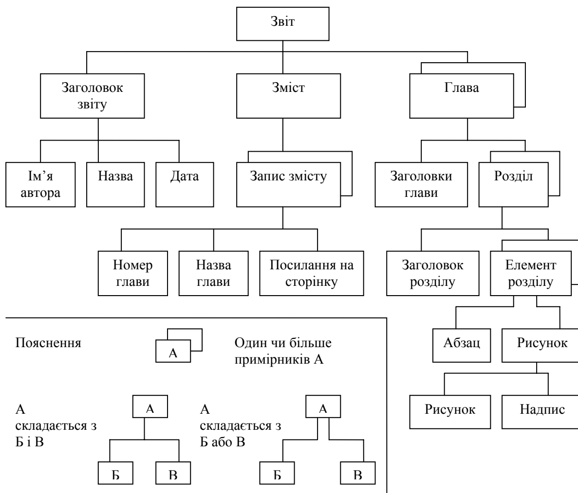
Рисунок 2.1 – Приклад логічного вигляду документа
