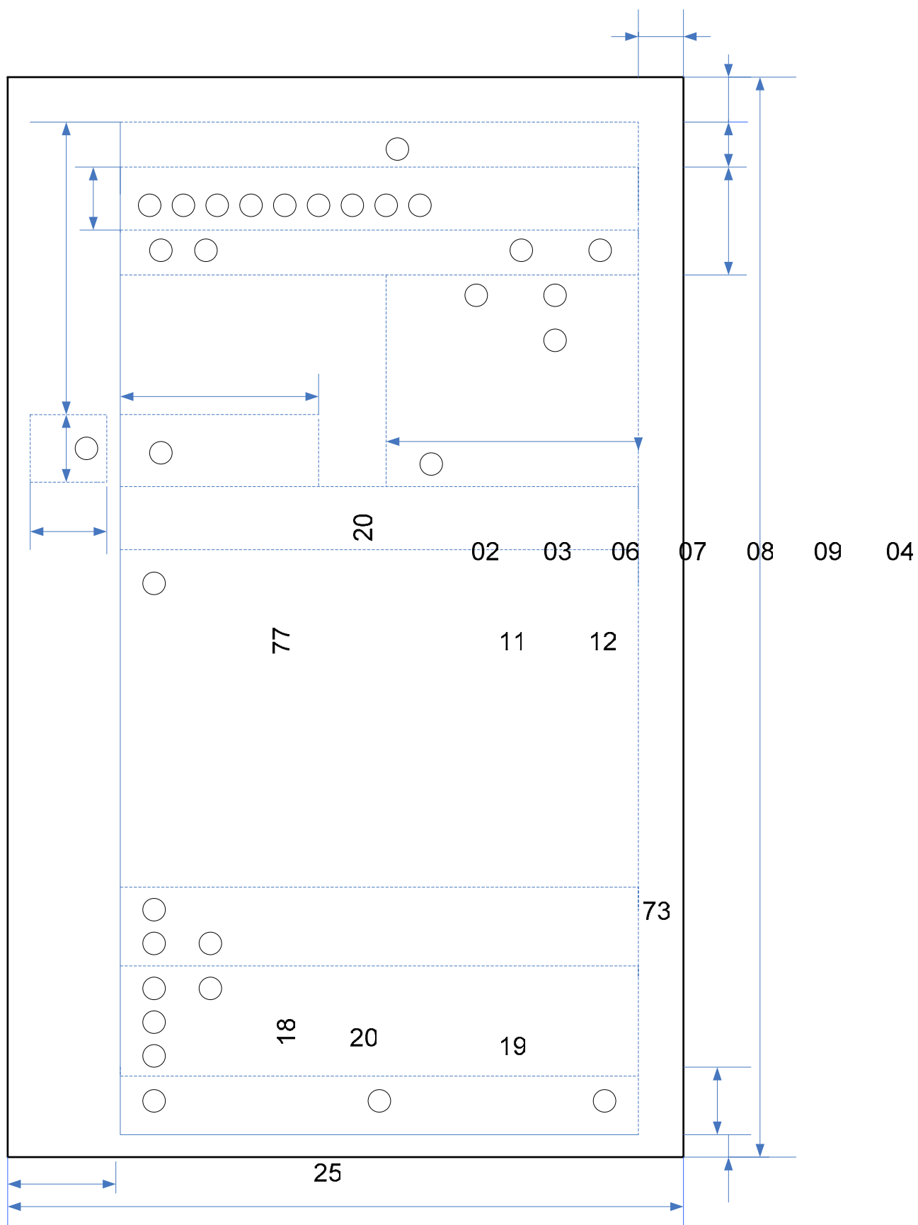
Рисунок А.2 – Розташування реквізитів та меж зон на форматі А4 поздовжнього бланка
