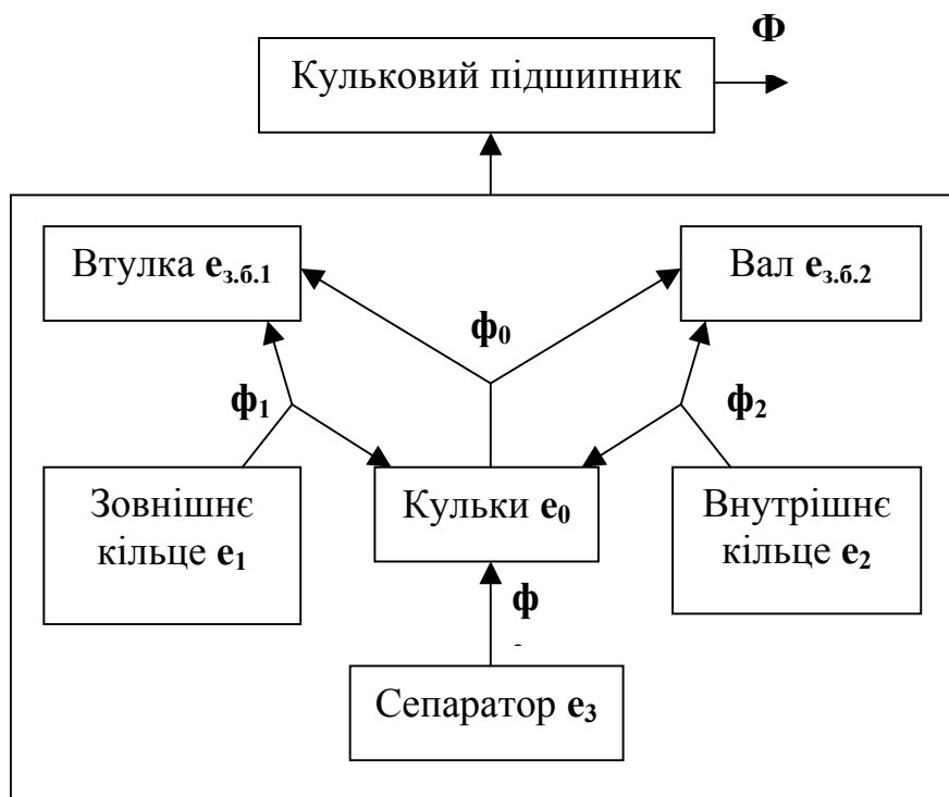
Рис. 5.3. ФС кулькового підшипника
