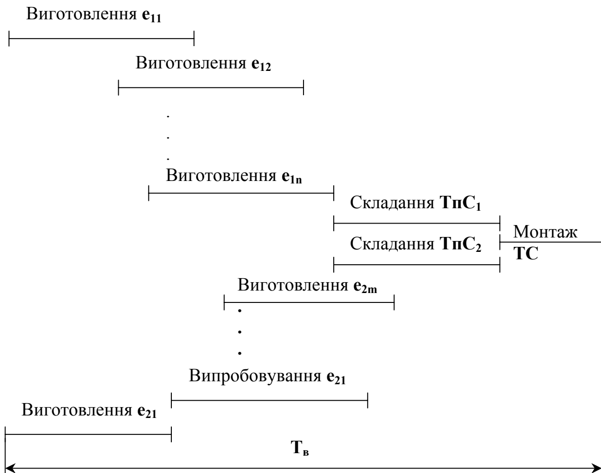
Рис. 10.4. Схема обчислення фактичної тривалості виробничого процесу ( T_v ) виготовлення ТС при певній технології
