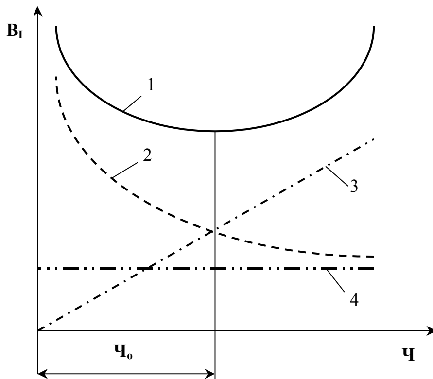
Рис. 7.9. Залежність для орієнтовного визначення оптимального числа ТО в партії ( \mathcal{C}_0 ) виходячи із витрат на один зразок ( B_I ): 1 – загальних; 2 – на виготовлення; 3 – на зберігання та транспортування; 4 – на матеріали
