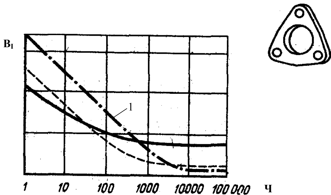
Рис. 7.8. Залежність вартості виготовлення ( B_I ) зразка ТО типу „прокладка” від варіанта технології його виготовлення та числа зразків в партії ( \mathcal{C} ): 1- технологія, орієнтована на масове виробництво
