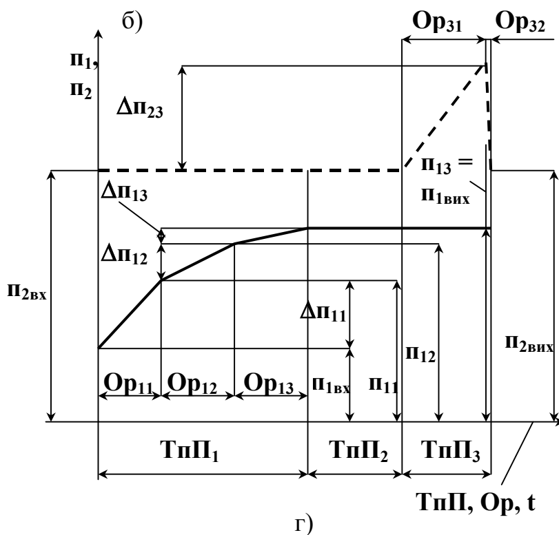
Рис. 4.3. Способи представлення ТП: а – блок-схема послідовності; б – структурна схема; в – ієрархічна схема; г – графіки основних робочих параметрів ТП
