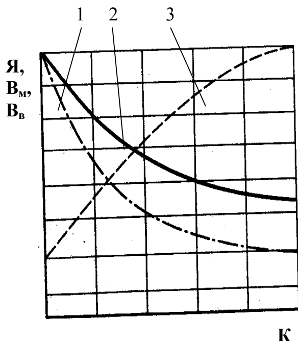
Рис. 7.12. Залежності: 1 - якості розробки (Я) ТО; 2 - витрат на матеріали ( B_m ); 3 - виробничих витрат ( B_v ) - від кваліфікації конструктора (К)
