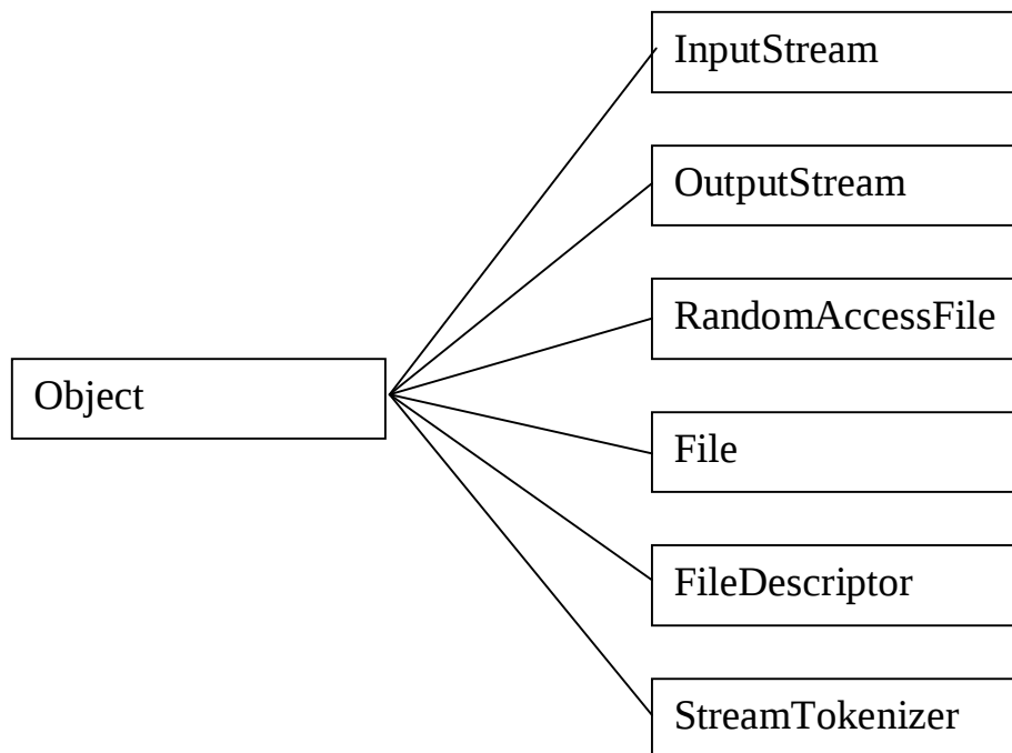
Рисунок 9 – Основні потокові класи
