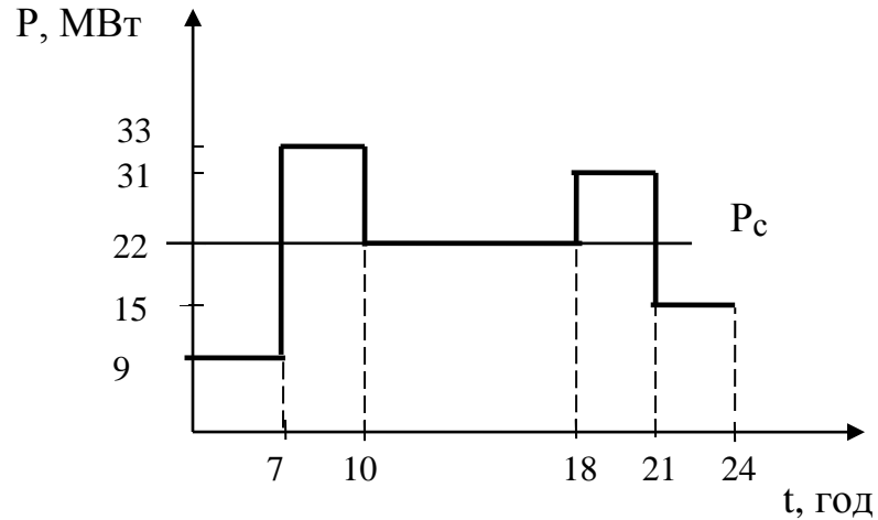
Рис. 2.5. Добовий графік навантаження промислового підприємства
