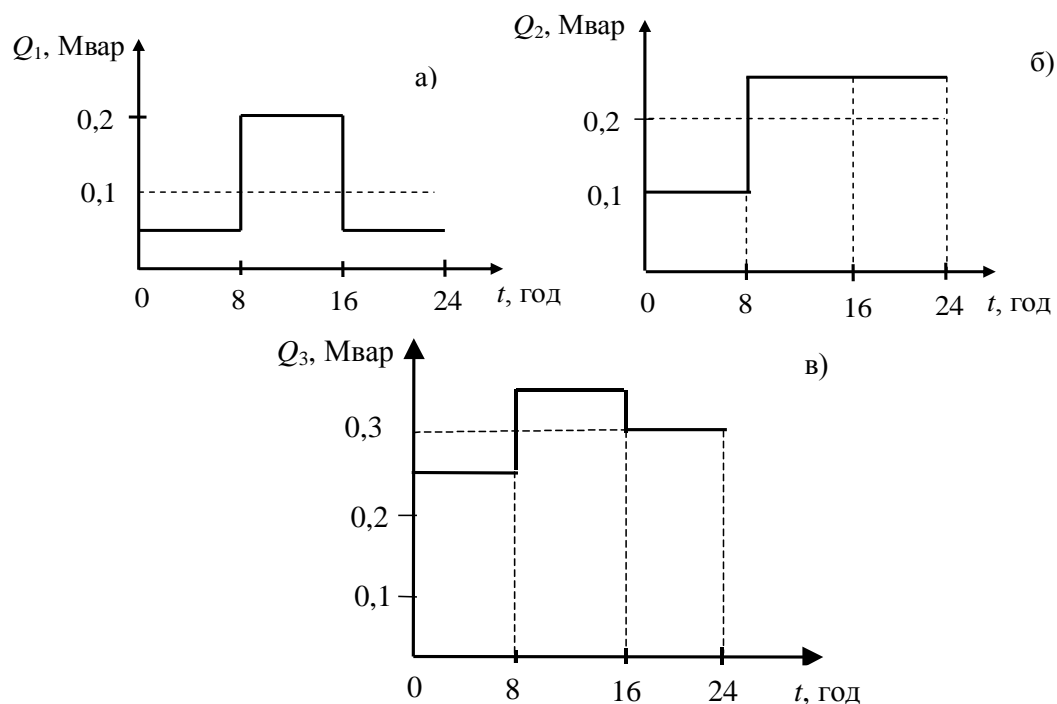
Рис. 3.6. Графіки реактивних навантажень споживачів магістральної мережі
