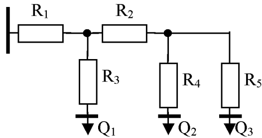
Рис. 3.5. Схема заміщення магістральної розподільної мережі
