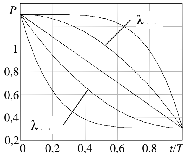
Рис. 1.5. Універсальні графіки навантажень за тривалістю
