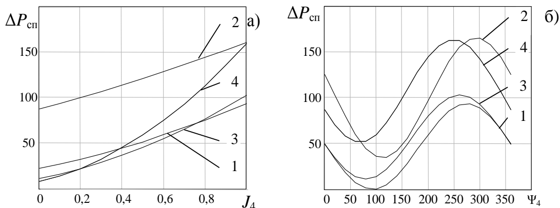
Рис. 2.2. Графіки втрат в навантаженнях споживачів
