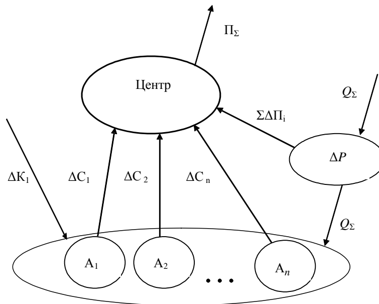
Рис. 3.2. Модель активної системи компенсації реактивної потужності
