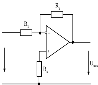
Рисунок 4.4 – Схема включення операційного підсилювача
