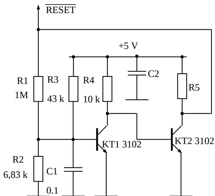
Рисунок 4.6 – Схема скидання мікроконтролера
