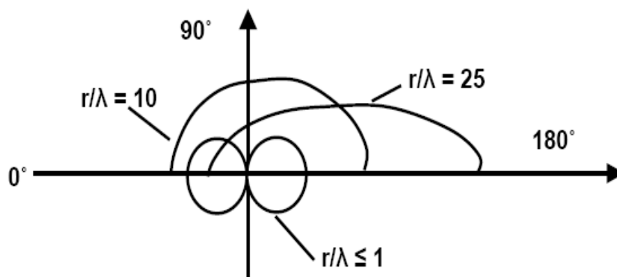
Рисунок 1.3 – Характерні індикатрисы аерозольного розсіювання
