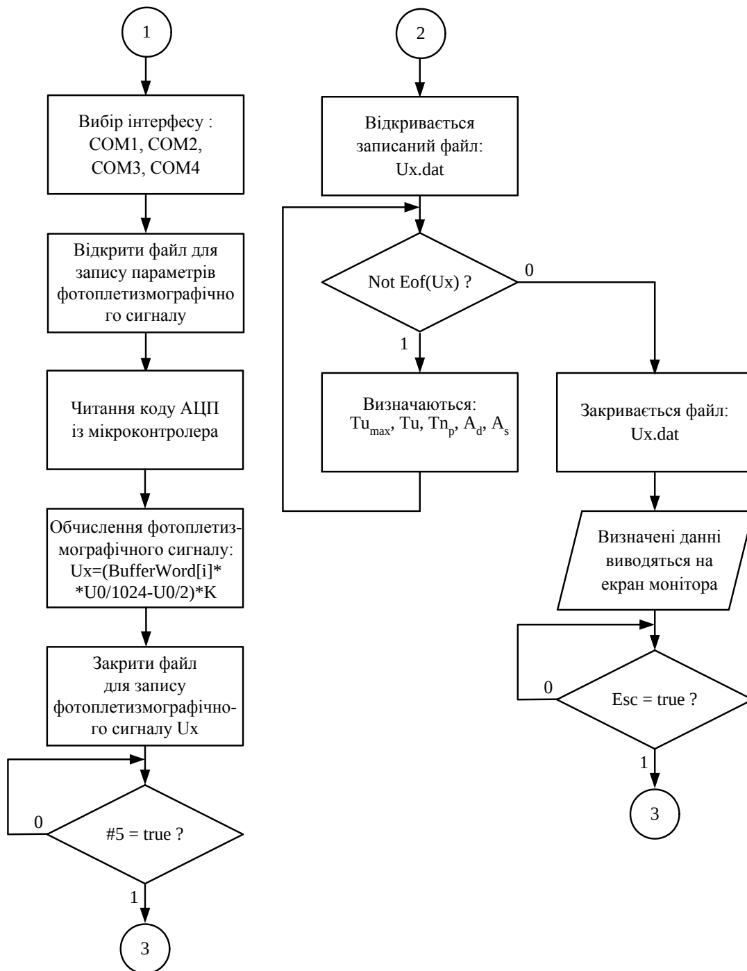
Рисунок 4.7 – Схема програми для персонального комп'ютера
