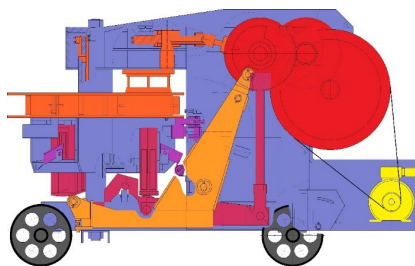
Напівавтомат для виготовлення цегли напісхум пресуванням
