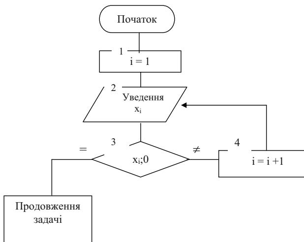
Рисунок 7.7 – Блок-схема до приклада 7.7.
