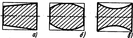
Рис. 3.20. Отклонения от цилиндричности в осевом сечении: а — конусообразность; б — бочкообразность; в — вогнутость
