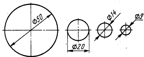
Рис. 2.43. Нанесение размеров диаметра окружности
