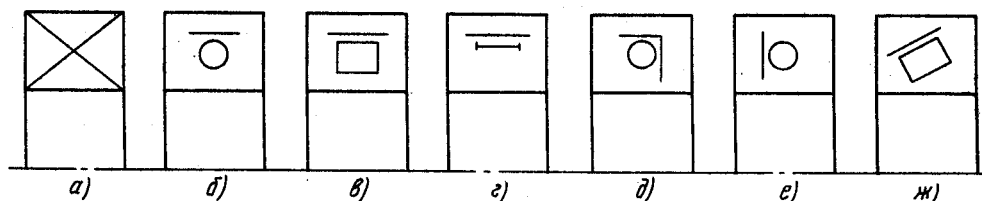
Рис. 3.14. Условное изображение подшипников качения: а — без указания типа; б — радиальный шариковый; в — радиальный роликовый; г — игольчатый; д — радиально-упорный шариковый; е — упорный шариковый; ж — роликовый конический
