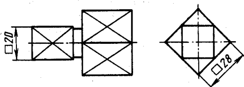
Рис. 2.46. Нанесение размеров квадрата
