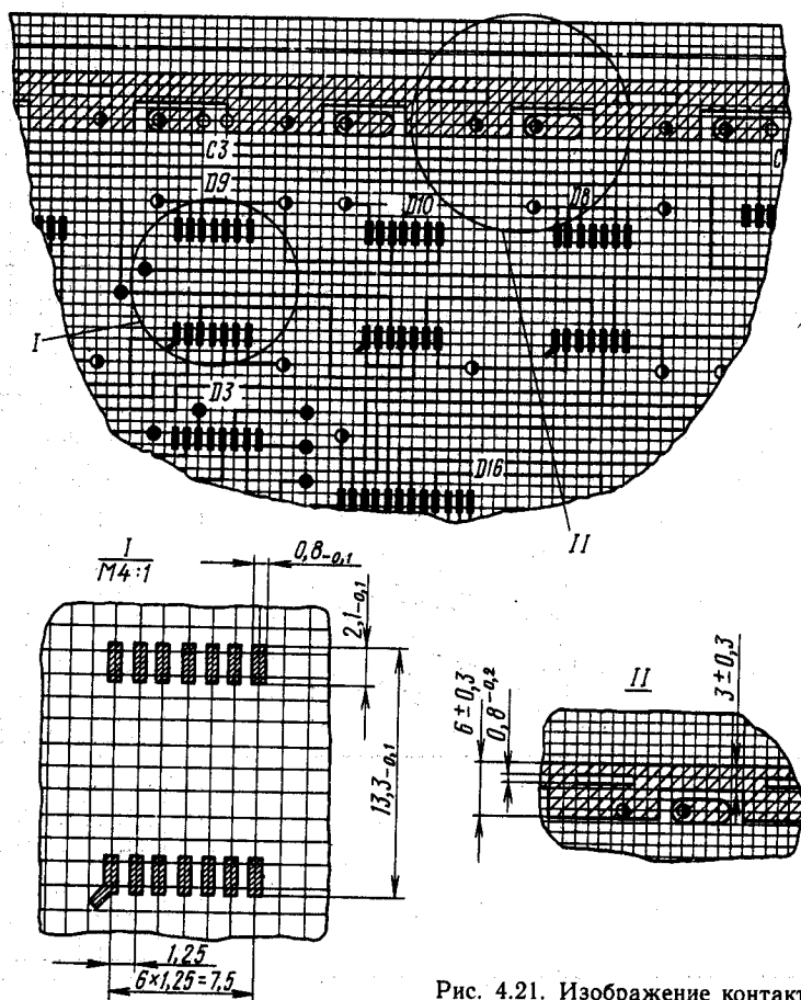
Рис. 4.21. Изображение контактной группы
