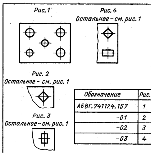
Рис. 3.46. Изображение исполнений на групповом чертеже
