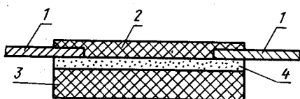
Рис. 8.2. Устройство тонкопленочного линейного резистора:
