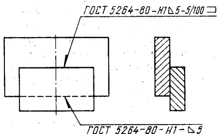
Рис. 3.9. Сварное соединение
