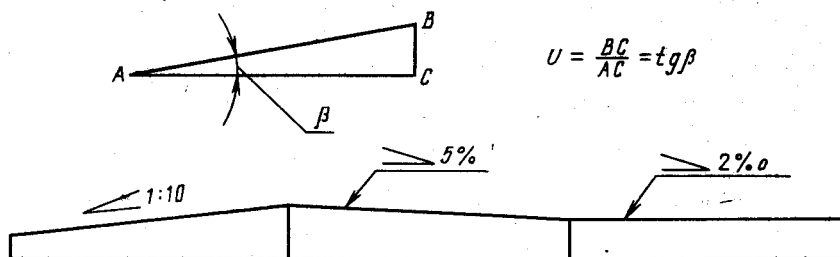
Рис. 2.47. Обозначение уклона
