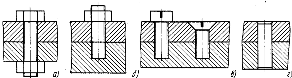
Рис. 3.8. Упрощенное изображение крепежных соединений: а — болтовое; б — шпильчатое; в — винтовое; г — штифтовое
