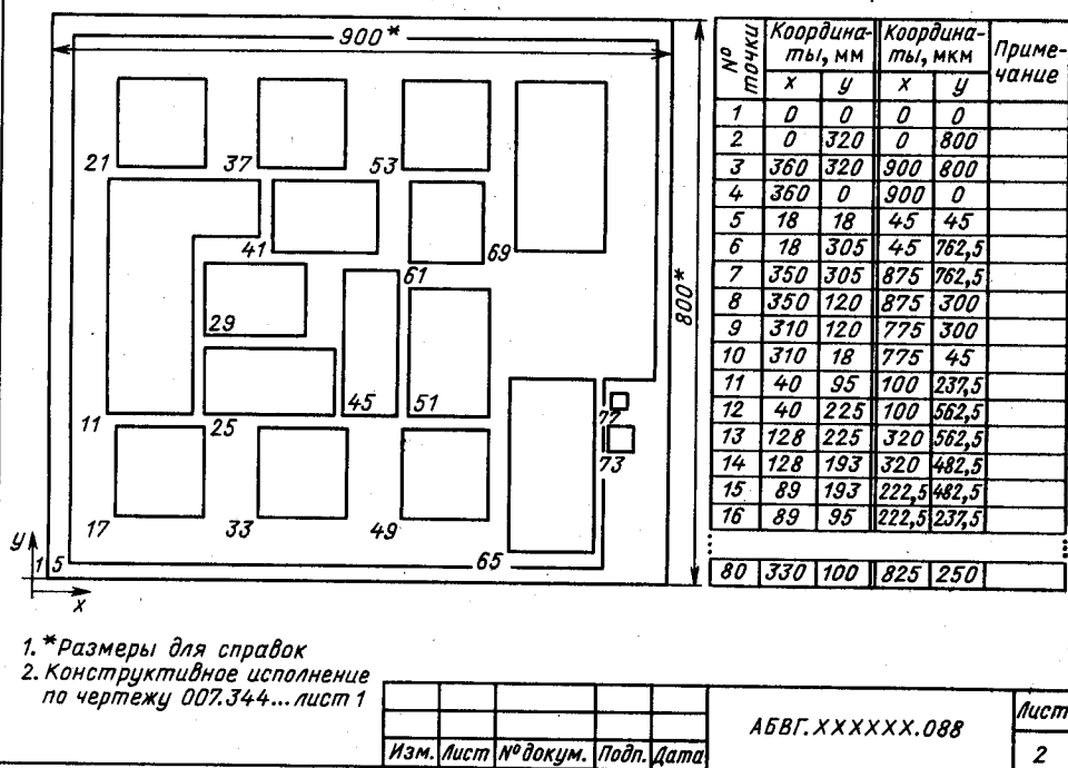
Рис. 8.24. Чертеж слоя полупроводниковой ИС, входящего в состав топологического чертежа
