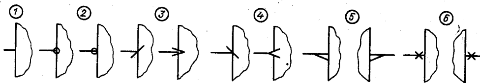
Рис. 7.15. Обозначение указателей входов-выходов:
