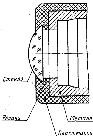
Рис. 2.30. Штриховка разнородных материалов
