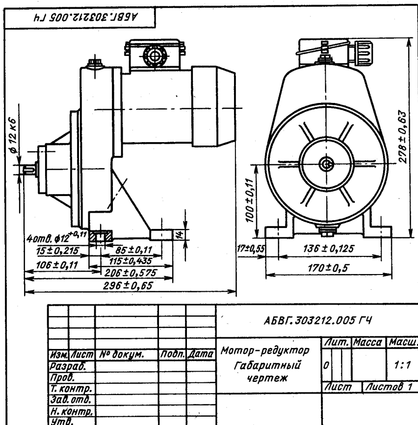
Рис. 3.39. Оформление габаритного чертежа
