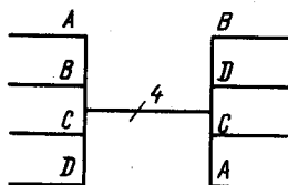
Рис. 5.10. Изображение слияния и разветвления линий связи
