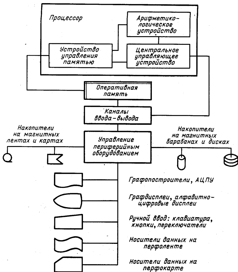
Рис. 10.1. Структурная схема ЕС ЭВМ
