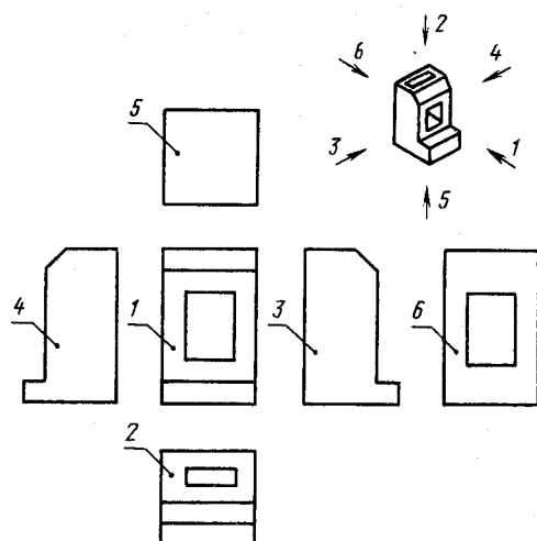
Рис. 2.20. Основные виды:
