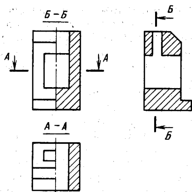
Рис. 2.22. Обозначение разрезов
