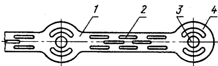
Рис. 4.24. Изображение проводников шириной более 5\text{ мм}
