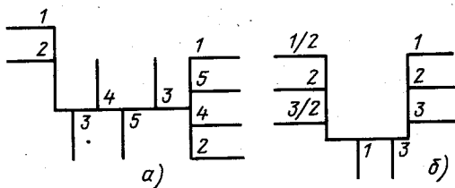
Рис. 5.7. Изображение групповых линий связи: а — без разветвлений; б — с разветвлениями
