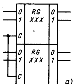
Рис. 7.20. Пример упрощенного изображения элементов
