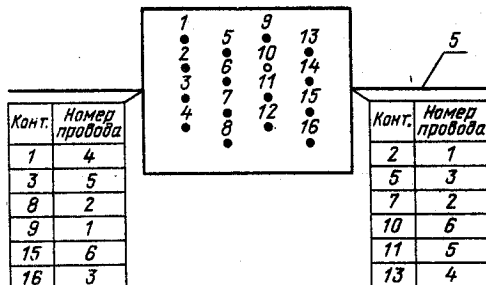
Рис. 6.19. Многоконтактное устройство с та- блицей соединений
