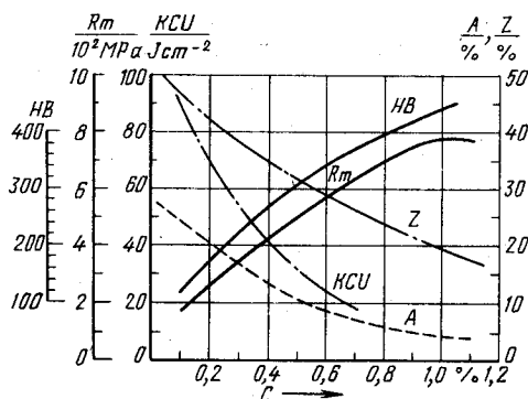
Рис. 9.4. Использование линий различных типов для изображения функциональных зависимостей
