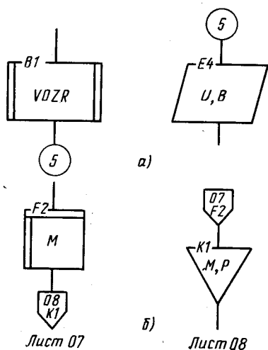
Рис. 10.9. Использование соединителей: а — на одной странице; б — межстраничный
