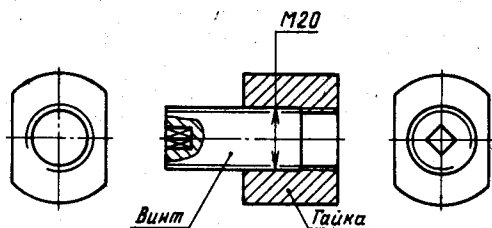
Рис. 3.7. Изображение резьбы
