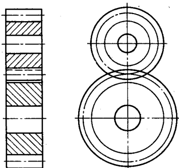
Рис. 3.11. Условное изображение зацепления цилиндрическими зубчатыми колесами
