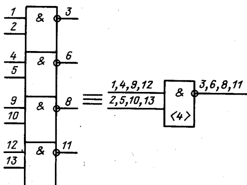
Рис. 7.23. Пакетное изображение элементов и связей
