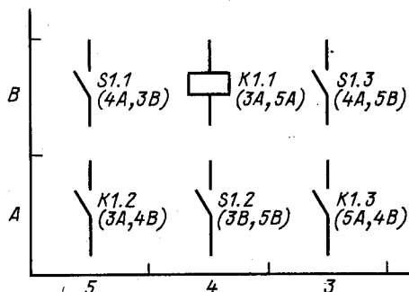
Рис. 5.17. Обозначение элементов на чертеже, разбитом на зоны
