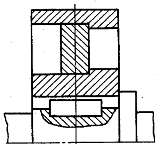
Рис. 3.40. Сварная сборочная единица на сборочном чертеже
