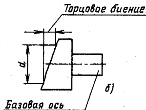
Рис. 3.22. Радиальное (а) и торцовое (б) биение
