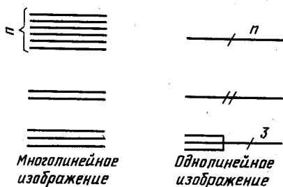
Рис. 5.9. Однолинейное представление линий связи
