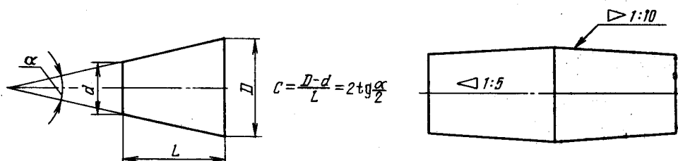
Рис. 2.48. Обозначение конусности
