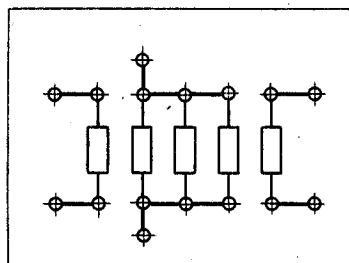
Рис. 4.26. Изображение контактов для подключения печатной платы:
