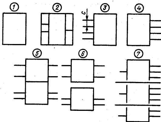
Рис. 7.14. Начертание условных графических обозначений:
