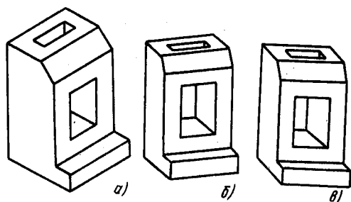
Рис. 2.32. Стандартные аксонометрические проекции:
