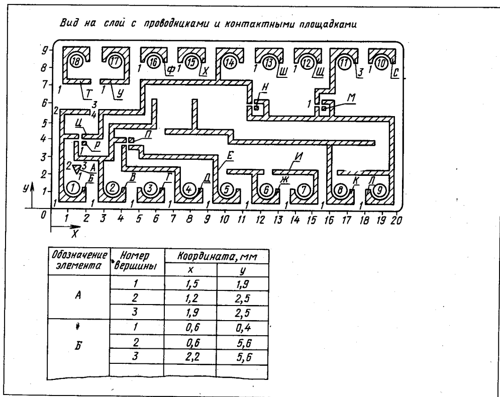
Рис. 8.16. Топологический чертёж слоя с проводниками и контактными площадками гибридной толстоплёночной микросхемы (3-й лист)
