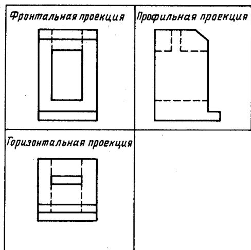
Рис. 2.19. Комплексный чертёж
