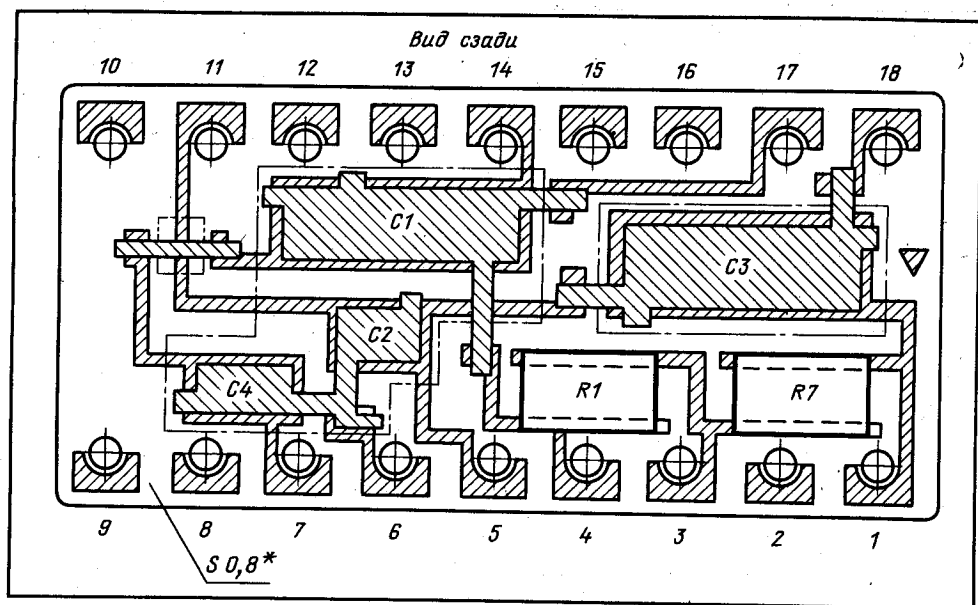
Рис. 8.15. Топологический чертёж гибридной толстоплёночной микросхемы, вид сзади (2-й лист)
