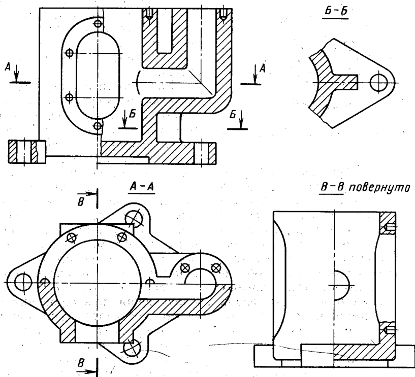
Рис. 2.24. Построение разрезов
