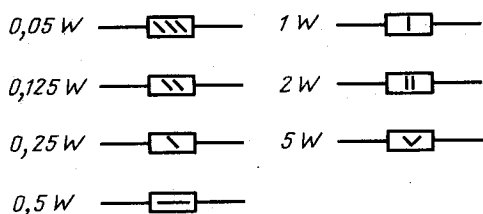
Рис. 5.23. Символы, обозначающие номинальную мощность резисторов
