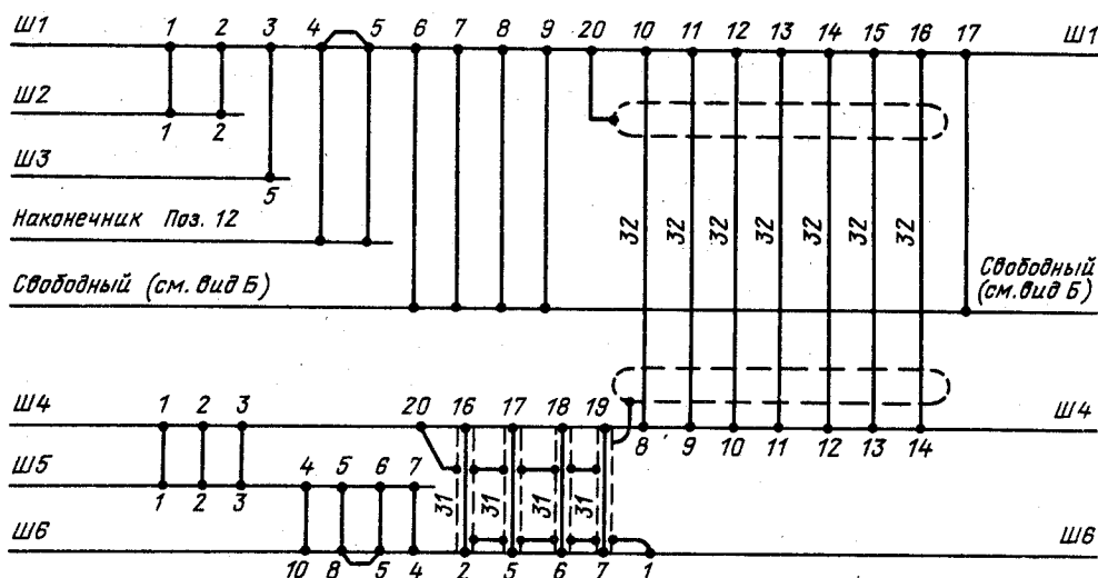
Рис. 4.9. Схема соединений
