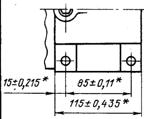
Рис. 3.38. Оформление сборочного чертежа
