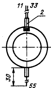
Схема обмотки
