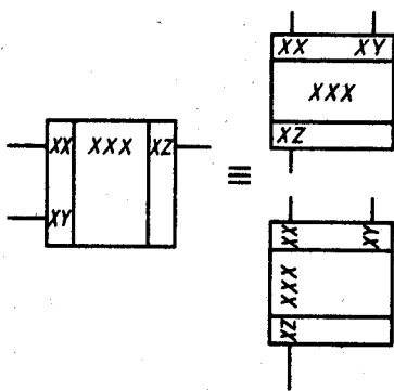
Рис. 7.13. Ориентация условного графического обозначения на схеме
