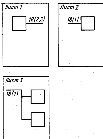
Рис. 7.1. Обозначение обрывов линий электрической связи
