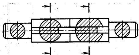
Рис. 2.28. Наложенные сечения
