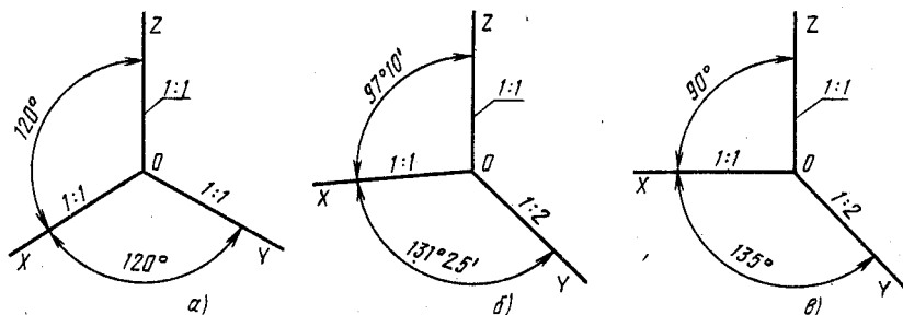
Рис. 2.33. Положение аксонометрических осей:
