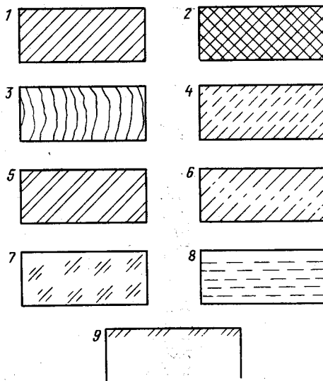
Рис. 2.29. Графические обозначения материалов:
