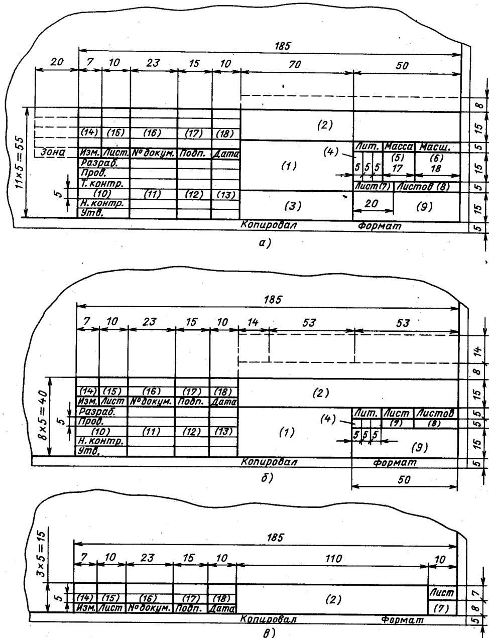
Рис. 2.2. Основная надпись:
