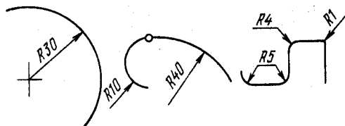
Рис. 2.44. Нанесение размеров радиуса
