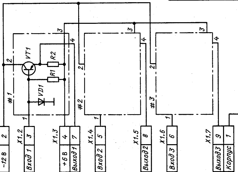
Рис. 6.11. Модуль П. Схема электрическая принципиальная
