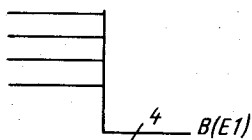
Рис. 5.19. Изображение обрыва линий связи в однолинейном представлении
