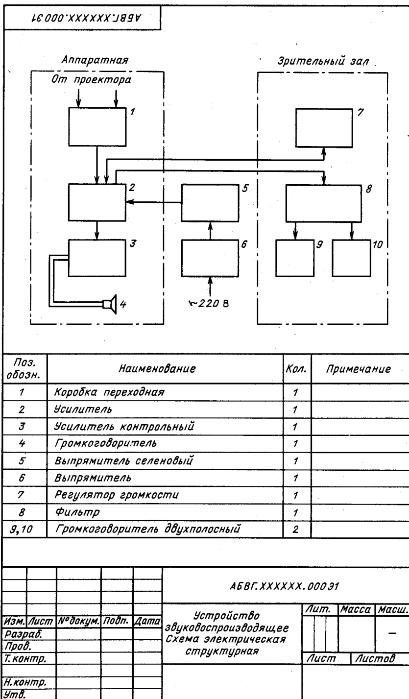
Рис. 6.2. Звукоспроизводящее устройство. Структурная схема
