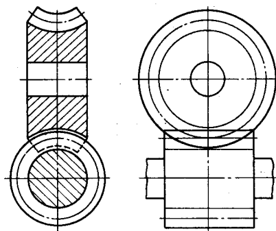
Рис. 3.13. Условное изображение червячного зацепления
