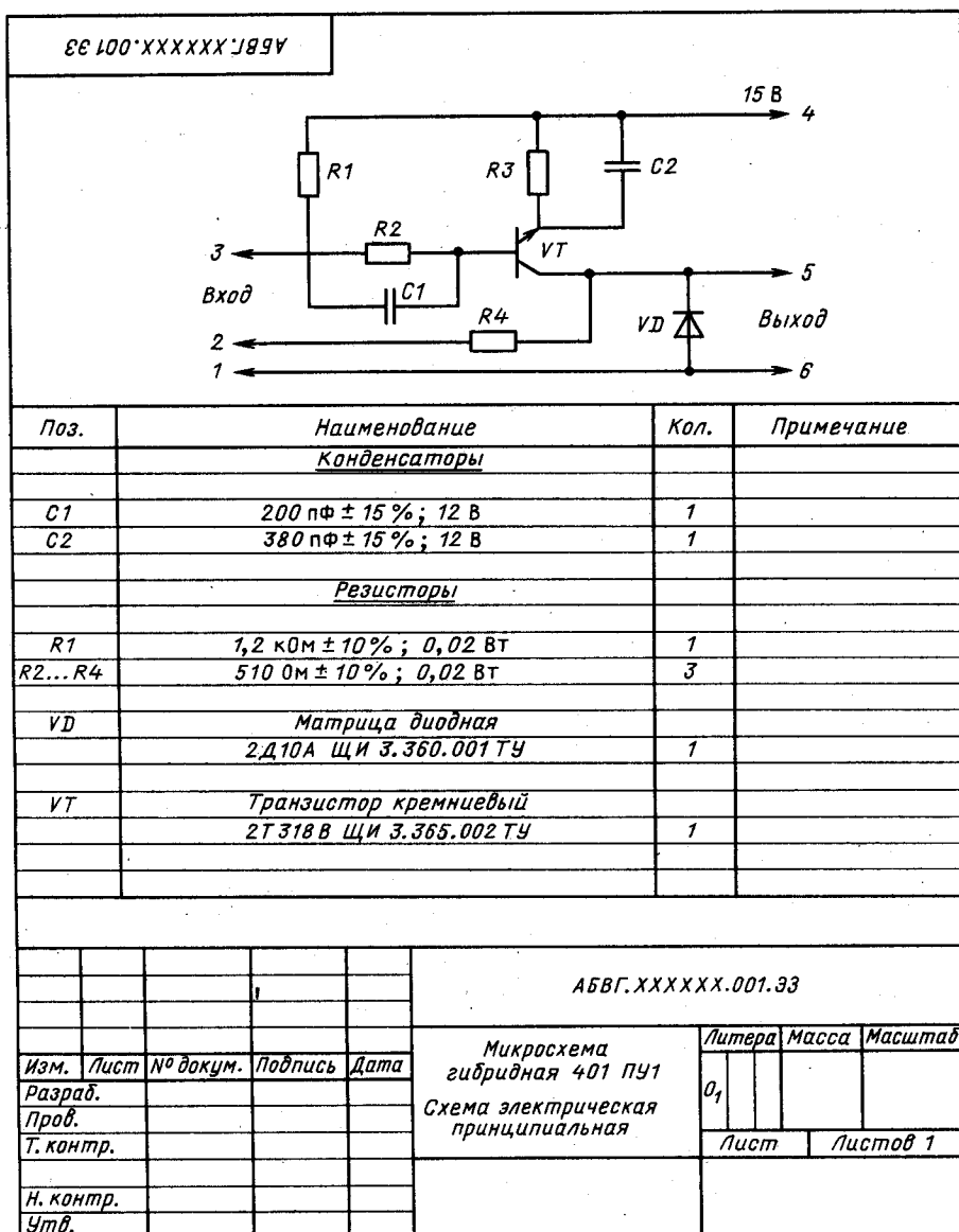
Рис. 8.6. Схема электрическая принципиальная тонкопленочной гибридной ИС
