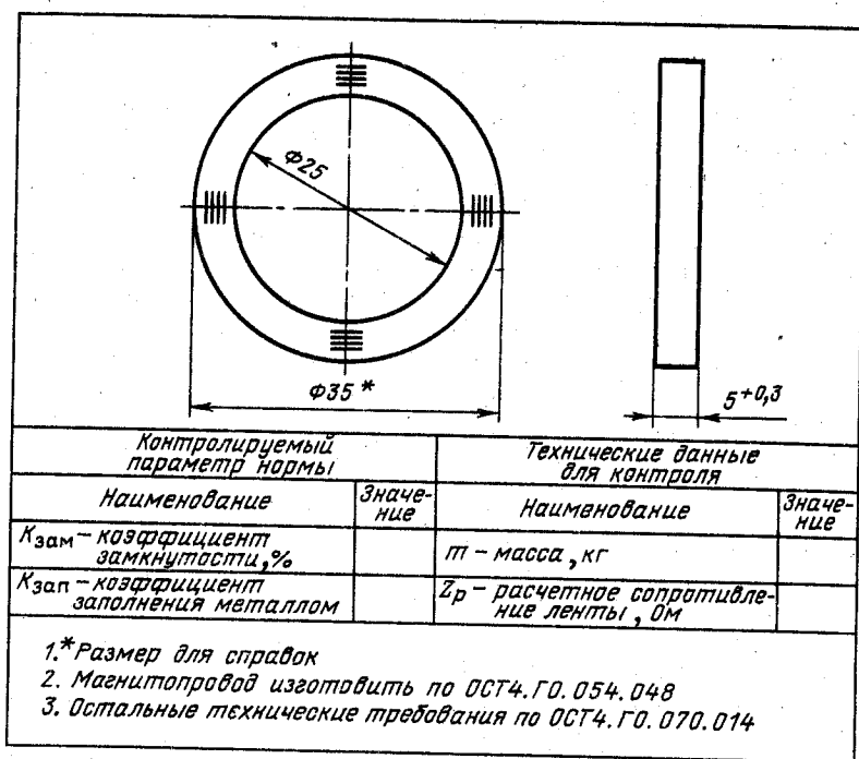
Рис. 4.17. Магнитопровод
