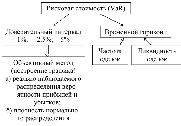
Рис. 4.2 – Ключевые параметры определения рисковой стоимости (VAR)
