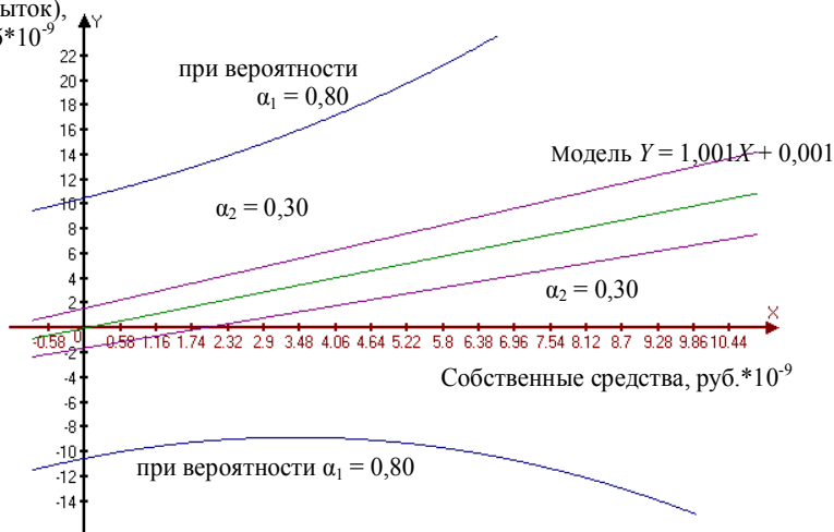
Рис. 5.9 – Доверительные интервалы линии регрессии 1.
