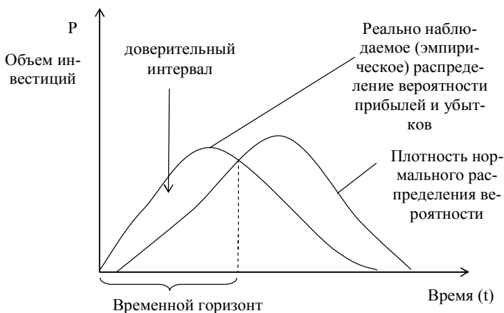
Рис. 4.3 – Объективный метод установления доверительного интервала и временного горизонта
