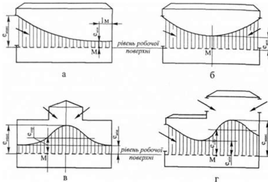
Рисунок 3.1 – Графічне зображення розподілу природної освітленості в приміщенні: а – в приміщенні з одностороннім боковим освітленням; б – в приміщенні з двостороннім боковим освітленням; в – верхнім освітленням; г – комбінованим (боковим + верхнім) освітленням
