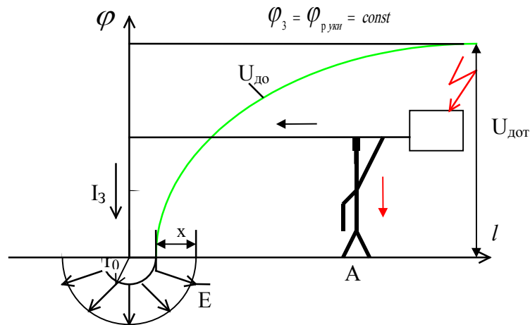
Рисунок 2.4 – Напруга дотику
