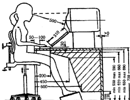
Рисунок 2.1 – Вимоги до організації робочого місця користувача ЕОМ
