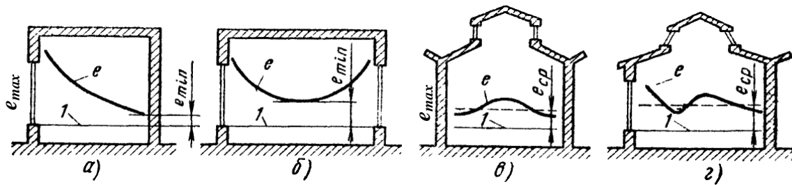
Рисунок 3.1 – Графічне зображення розподілу природного освітлення в приміщенні:
