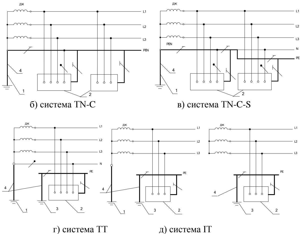
Рисунок 2.2 – Приклади виконання систем TN-S, TN-C, TN-C-S, TT та IT в трифазних електроустановках змінного струму:
