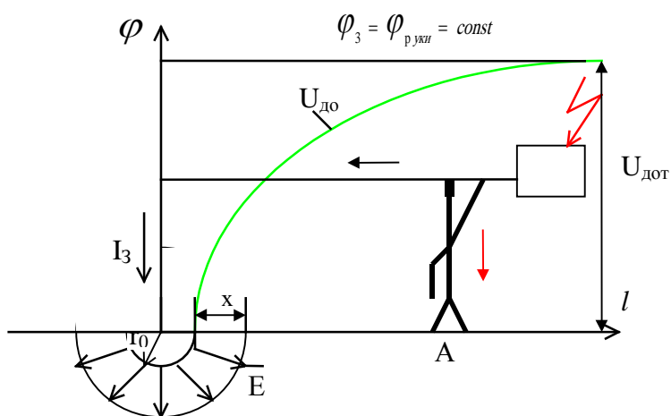
Рисунок 2.4 – Напруга дотику
