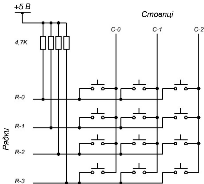
Рисунок 3.10 – Матрична клавіатура 4×3
