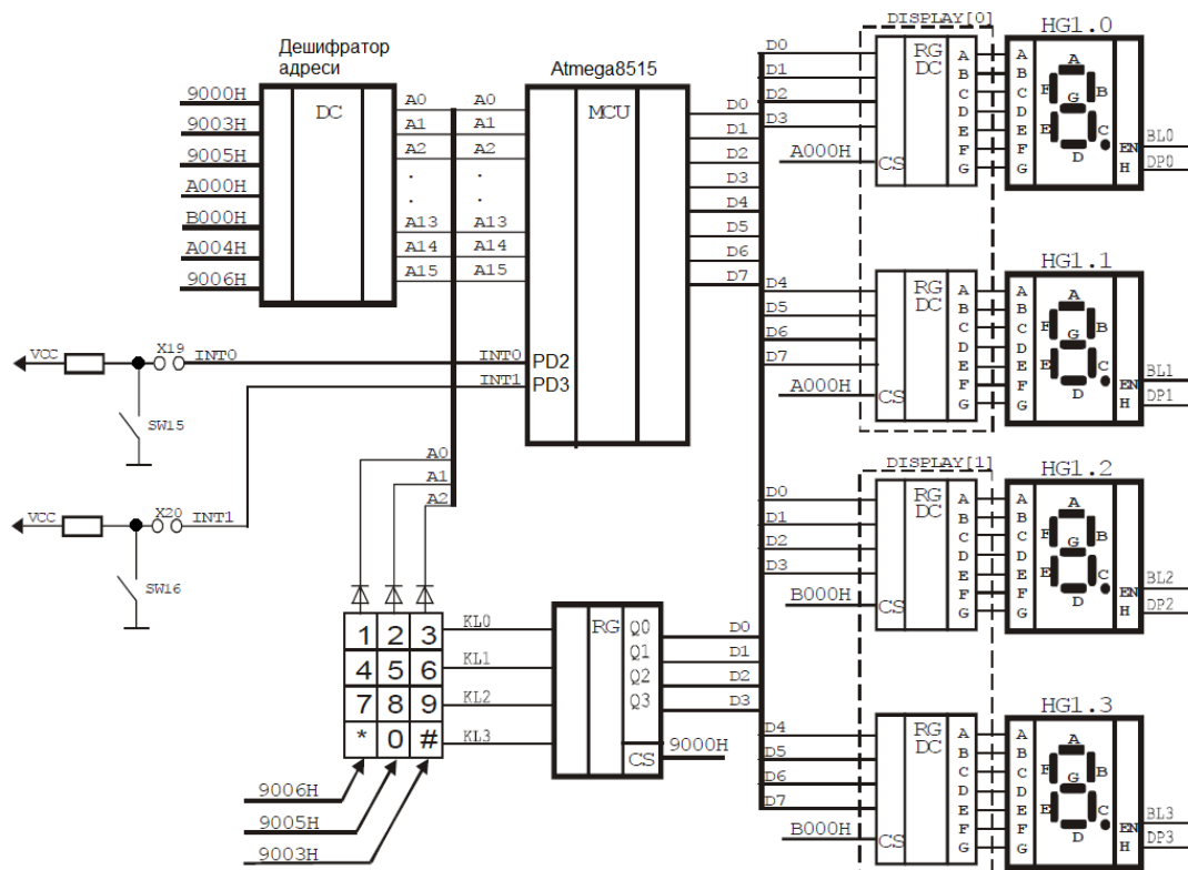
Рисунок 3.12 – Схема організації клавіатури та дискретних датчиків стенда EV8031/AVR
