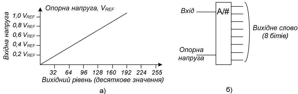
Рисунок 3.21 – До розгляду роботи АЦП
