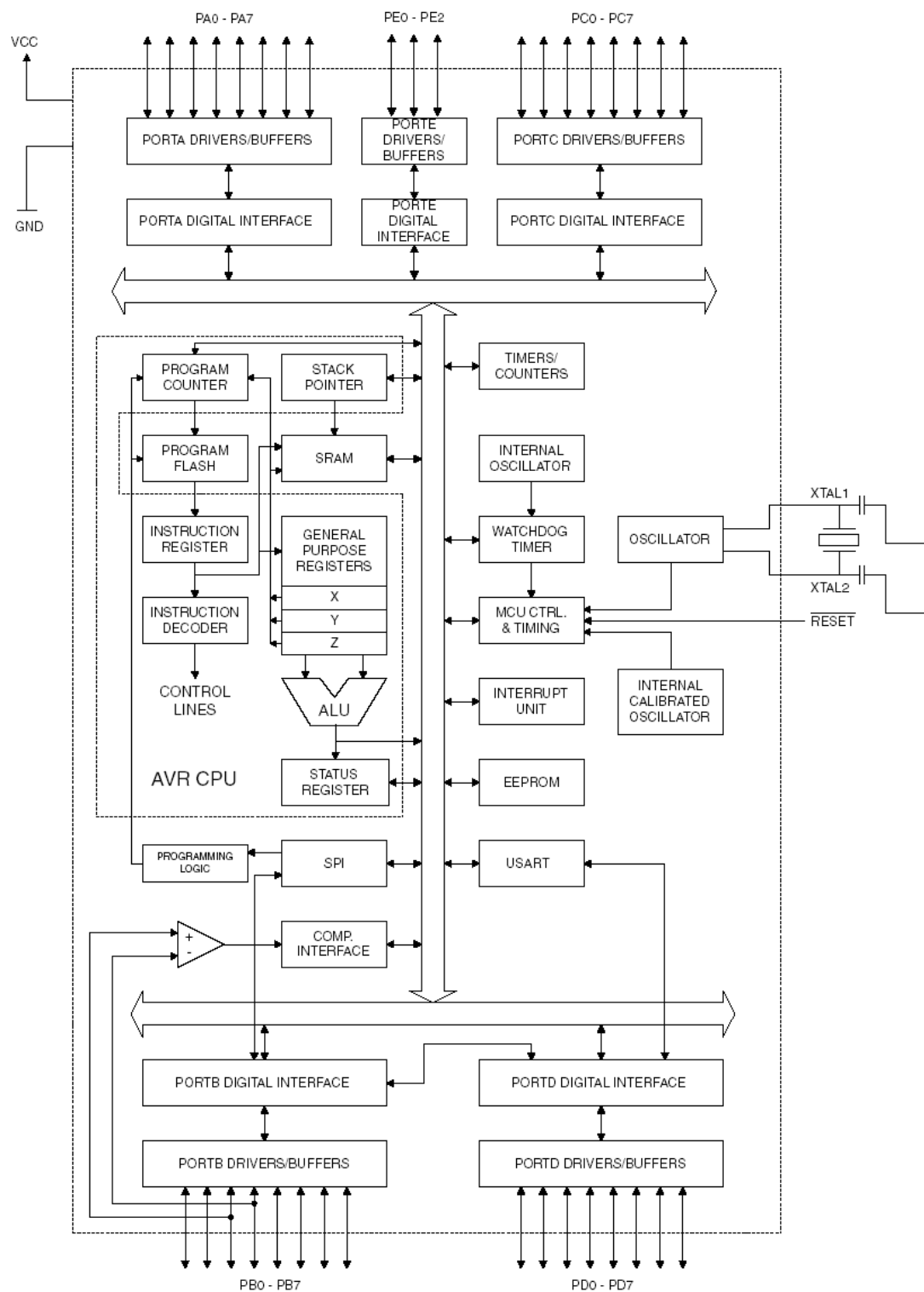
Рисунок 1.11 – Архітектура мікроконтролера ATmega8515
