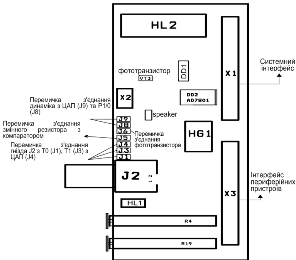
Рисунок 1.6 – Схема розміщення елементів плати розширення EV8031/AN
