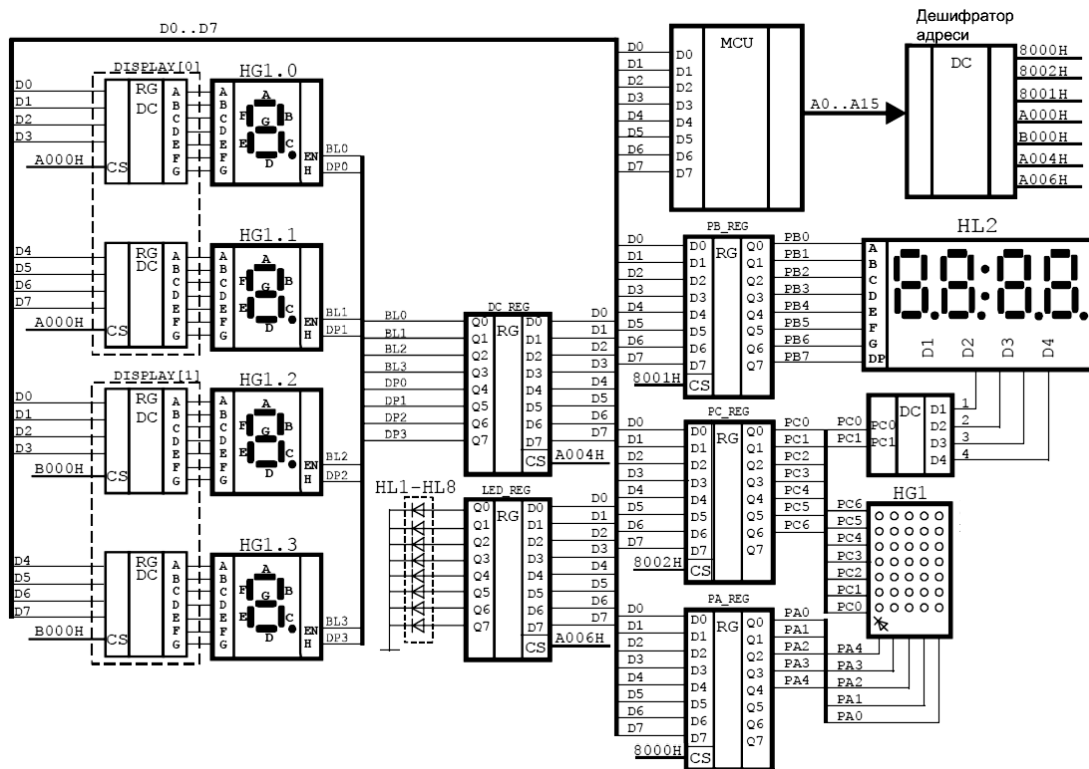
Рисунок 3.3 – Схема статичної та динамічної індикації стенда EV8031/AVR
