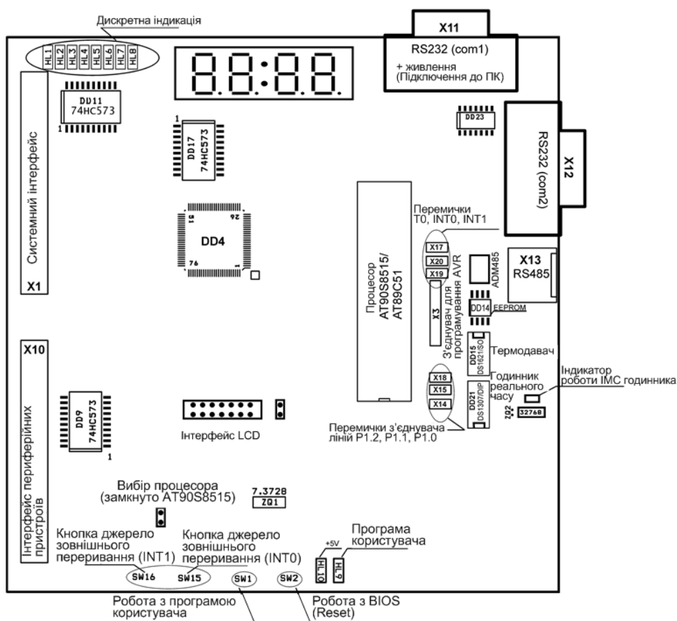
Рисунок 1.4 – Схема розміщення елементів лабораторного макета
