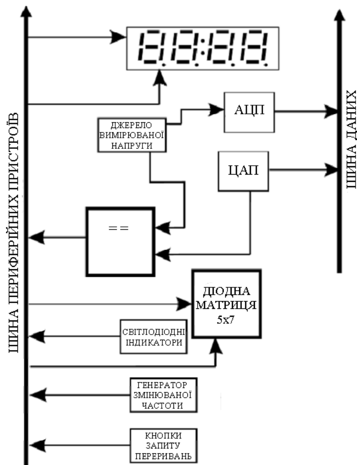
Рисунок 1.5 – Структурна схема плати розширення EV8031/AN
