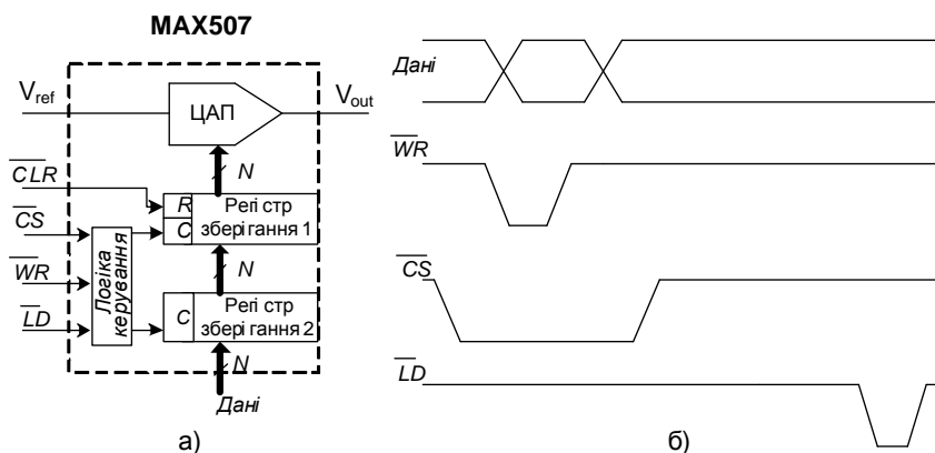
Рисунок 3.16 – ЦАП з паралельним інтерфейсом: а) структурна схема; б) часова діаграма
