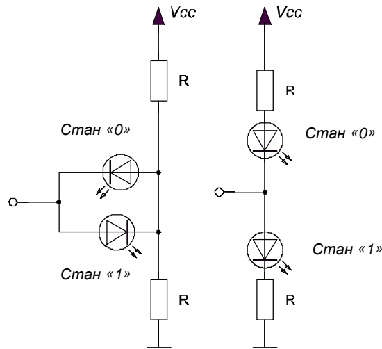
Рисунок 3.2 – Керування двома світлодіодами одним виводом МК
