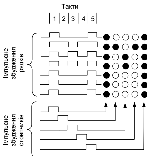
Рисунок 3.6 – Часова діаграма формування матричним індикатором літери М
