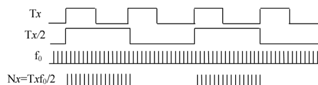
Рисунок 3.24 – Вимірювання періоду методом підрахунку імпульсів відомої частоти
