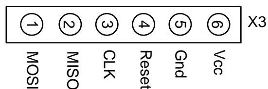
Рисунок 1.2 – З'єднувач для програмування мікроконтролера AVR
