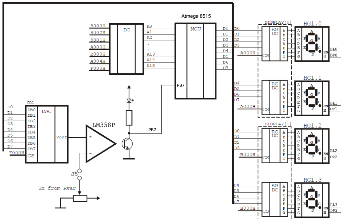
Рисунок 3.19 – Схема підключення мікросхеми ЦАП AD7801 на платі розширення стенда EV8031/AN
