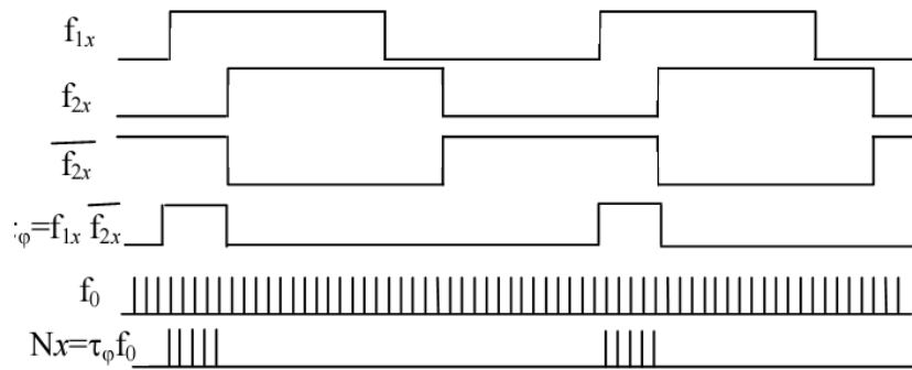
Рисунок 3.25 – Вимірювання зсуву фаз
