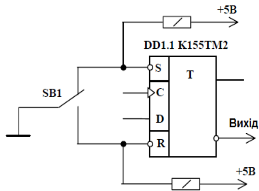
Рисунок 3.11 – Схема усунення «тремтіння» контактів RS-тригером
