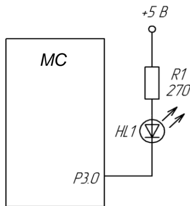
Рисунок 3.1 – Схема під'єднання світлодіодного індикатора
