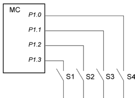
Рисунок 3.8 – Підключення кнопок або простих датчиків до МК
