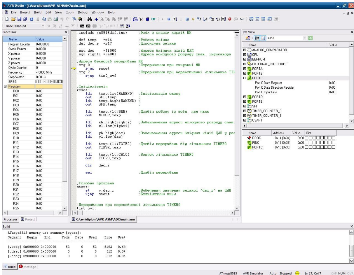
Рисунок 2.1 – Вікно середовища AVR Studio
