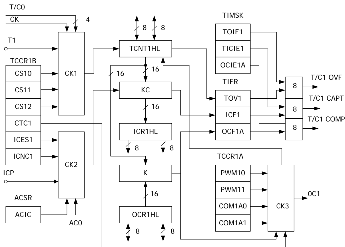
Рисунок 3.27 – Структурна схема таймера-лічильника типу D
