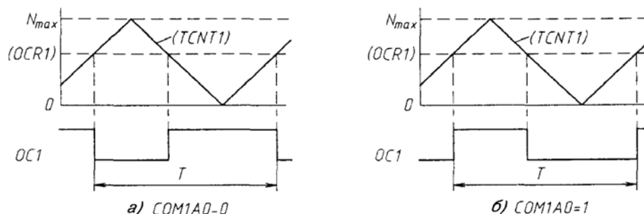
Рисунок 3.28 – Графіки зміни числа в базовому лічильнику (TCNT1) і часові діаграми сигналу PWM при різних станах розряду COM1AT
