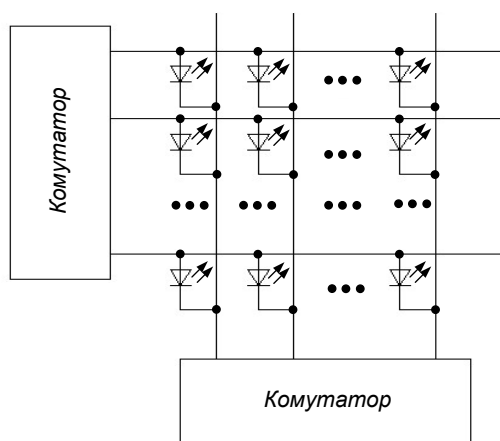
Рисунок 3.4 – Організація динамічної індикації
