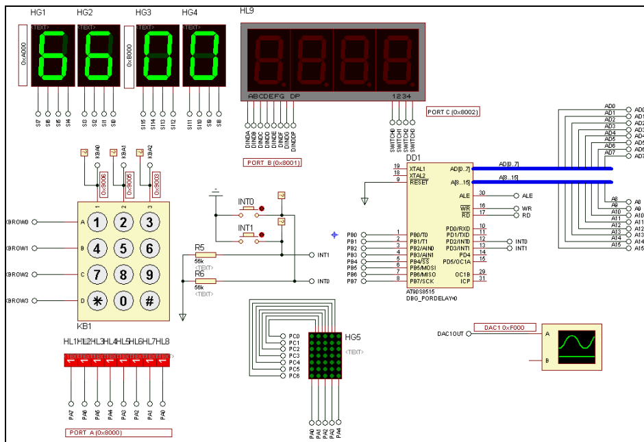
Рисунок 1.7 – Фрагмент віртуального стенда у середовищі Proteus VSM
