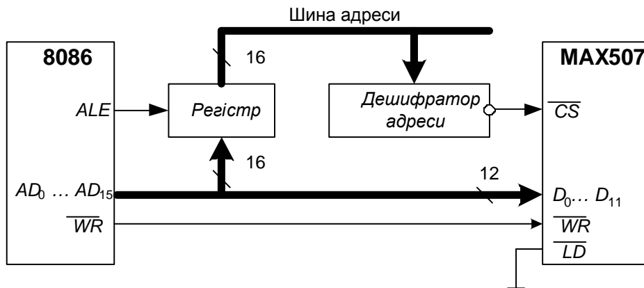
Рисунок 3.17 – Підключення ЦАП з паралельним інтерфейсом до МП 8086
