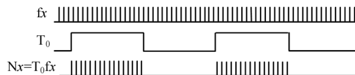
Рисунок 3.23 – Вимірювання частоти
