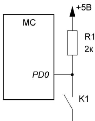
Рисунок 3.7 – Підключення контактного датчика до МК
