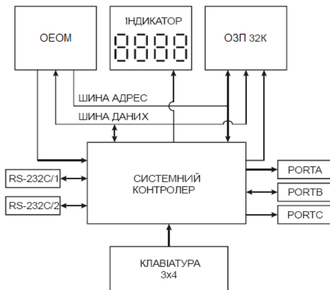
Рисунок 1.3 – Структурна схема стенда
