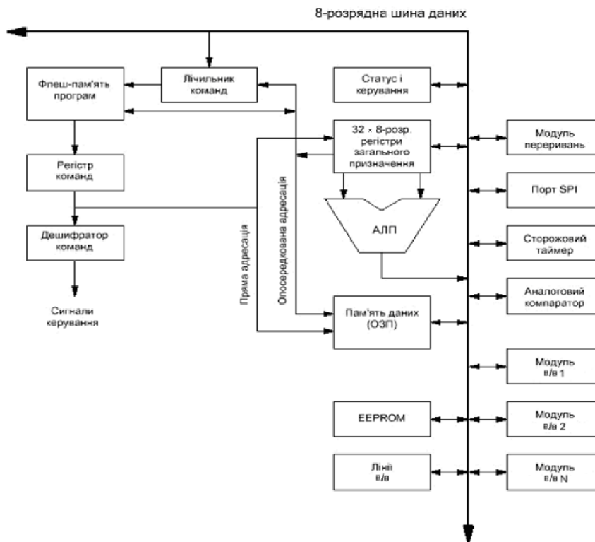
Рисунок 1.10 – Блок-схема архітектури AVR
