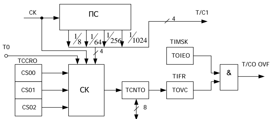
Рисунок 3.26 – Структурна схема таймера-лічильника типу А
